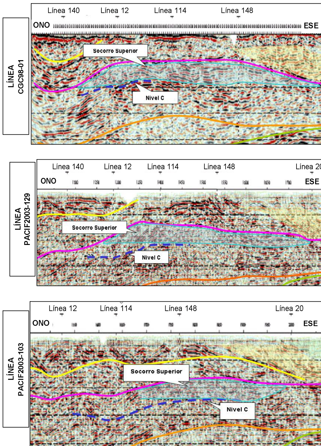
Figura 5.16.- Sección superior de la Fm. Socorro en líneas impares del área de estudio.
