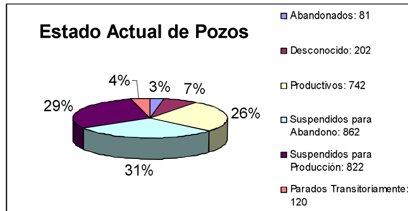
Figura 3.2.- Estado de pozos a Diciembre de 1998 (CGC, 1999).
