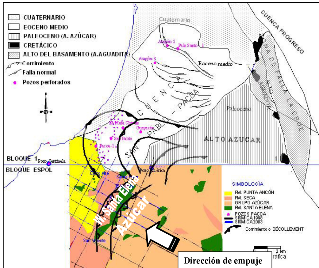
Figura 6.6.- Dirección de sobrecorrimientos de las Napas del Wildflysch Santa Elena y Azúcar (Modificado de Benitez, 1995)
