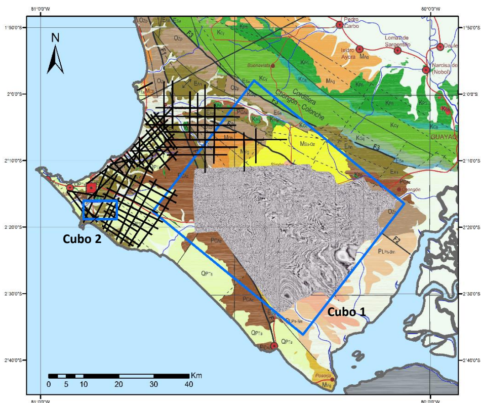
MAPA I Mapa geológico del área de interés y distribución de datos utilizados (Modificado de Reyes & Michaud, 2012)
