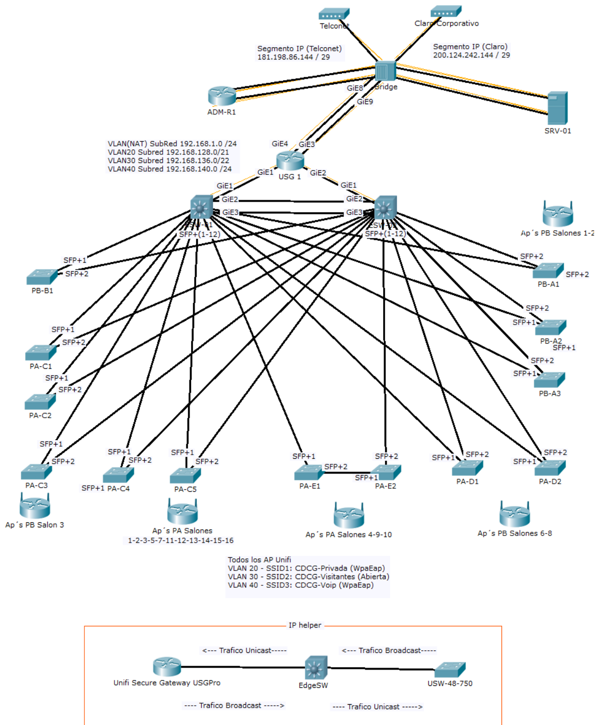
Figura 2.11: Diagrama Lógico de Red.
