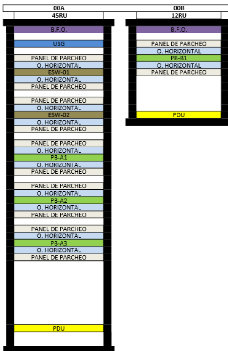
Figura 2.6: Elementos que conforman los rack – Planta Baja.
