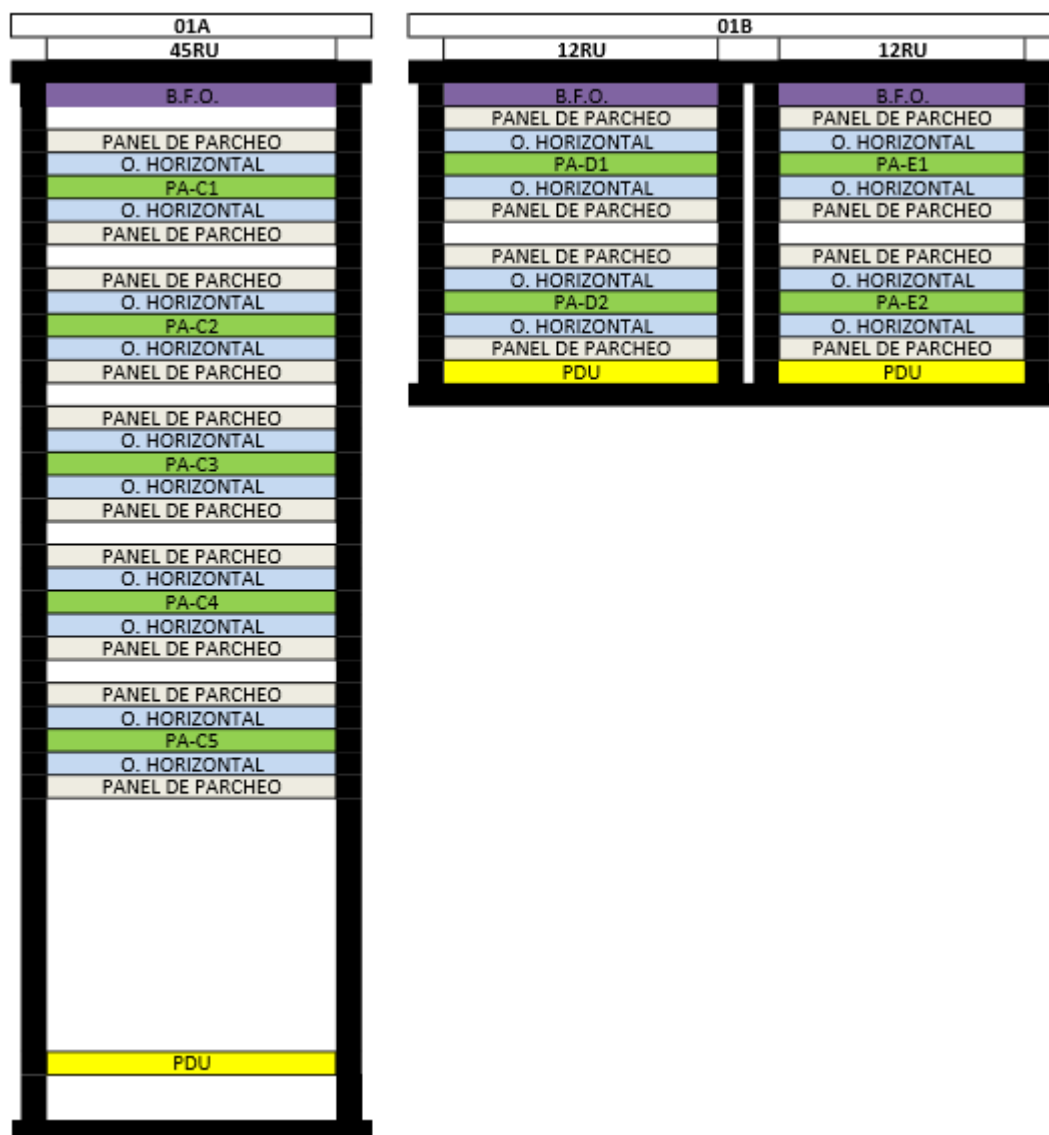
Figura 2.7: Elementos que conforman los rack – Planta Alta.
