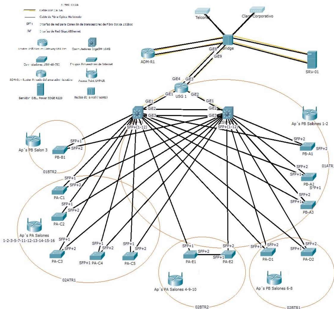
Figura 2.10: Diagrama Físico de Red.
