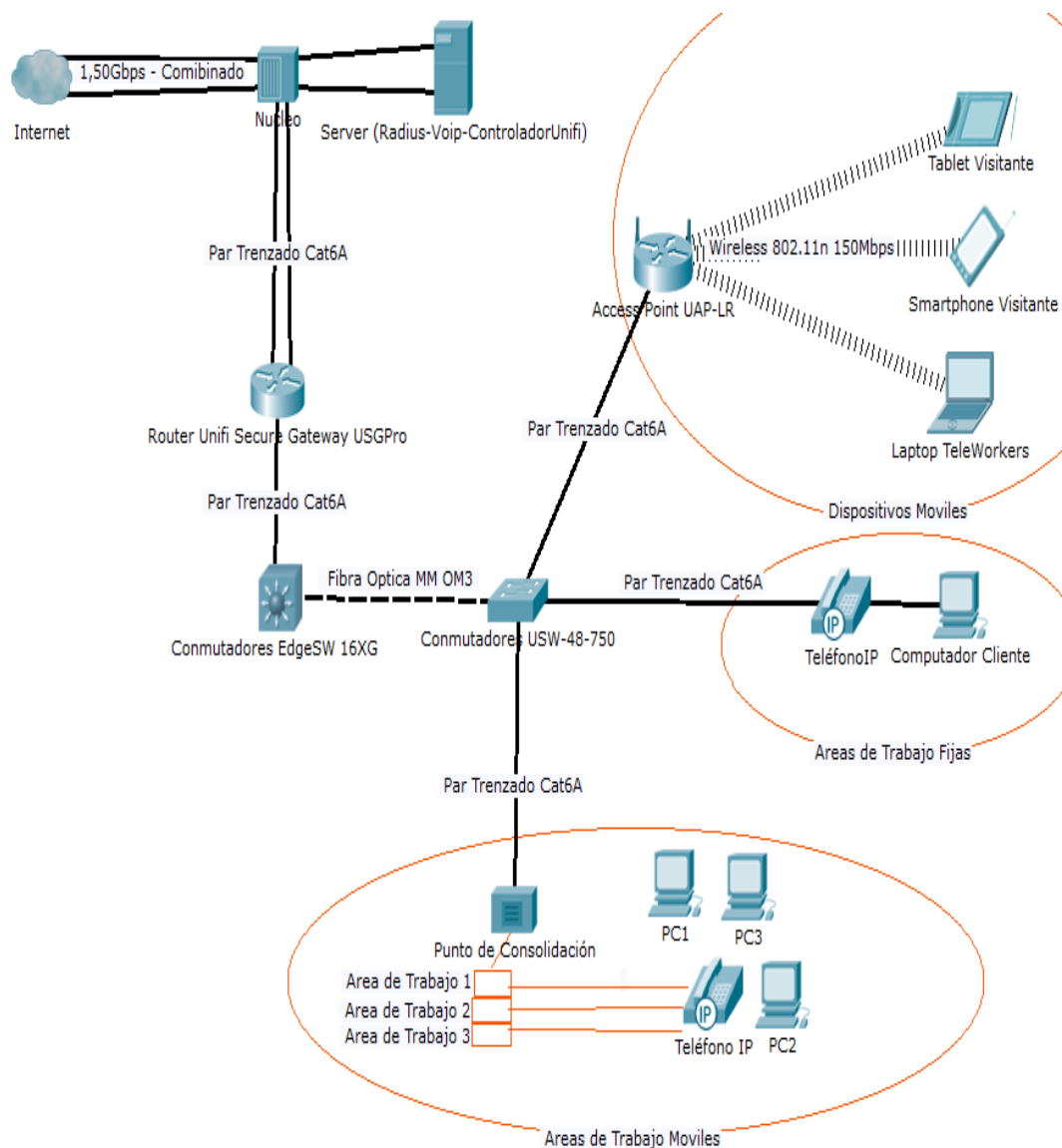
Figura 2.1: Diseño de Solución de Red Convergente.
