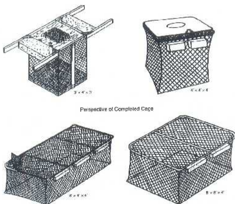
Fig # 2 Tipos de jaulas cuadradas o rectangulares
