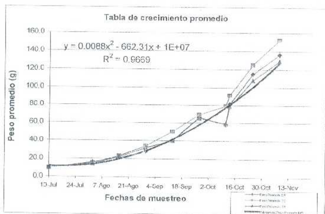
Gráfico # 1 Crecimiento promedio de las tres densidades en las jaulas
