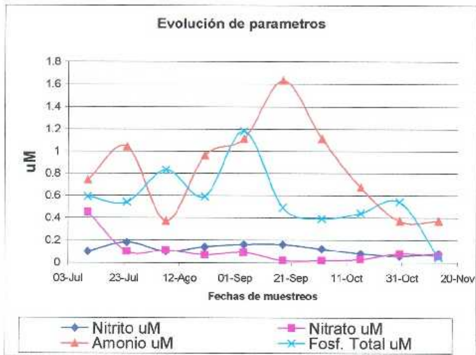
Grafico # 12 Evolución de Parámetros (Nitritos, Amonio, Nitratos y fósforo total)
