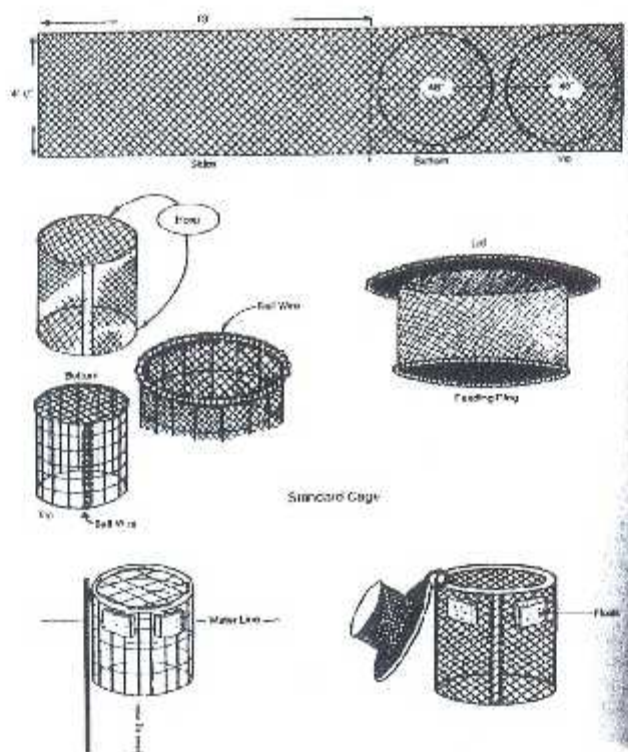
Fig # 1 Forma de construcción de una jaula circular
