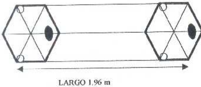
Fig # 4 Diseño de las jaulas para el cultivo de tilapia
