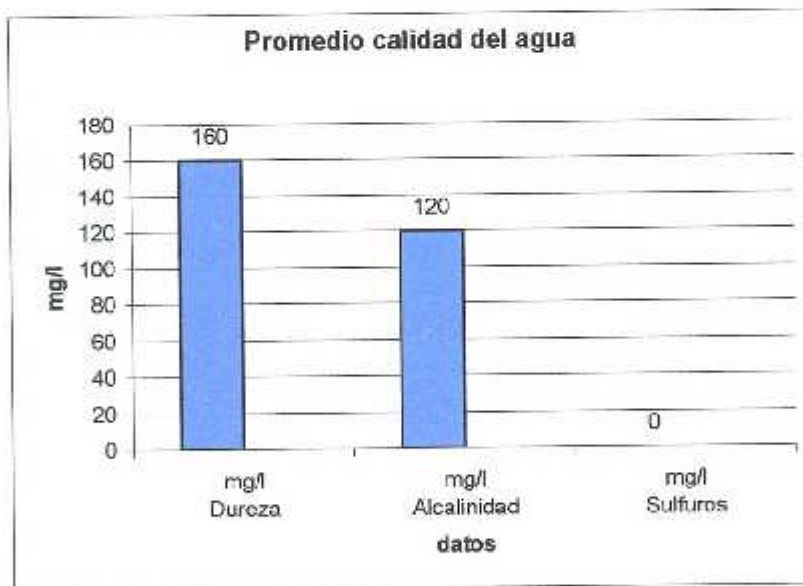
Grafico # 15 Valores Promedios de dureza, alcalinidad y sulfuros
