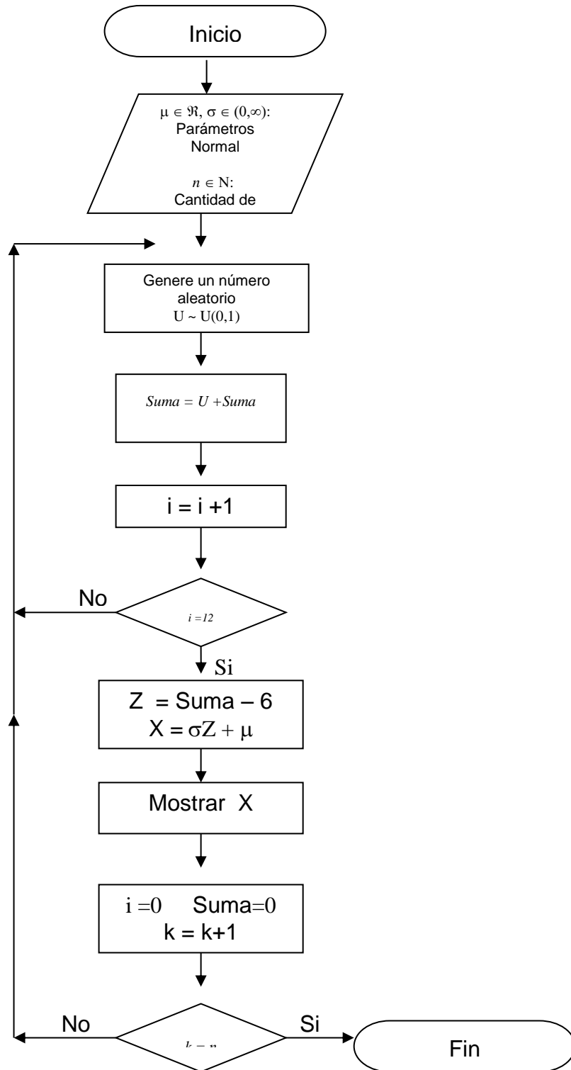
Diagrama de flujo de la simulación de una muestra de tamaño n proveniente de una población normal con parámetros \mu y \sigma^2
