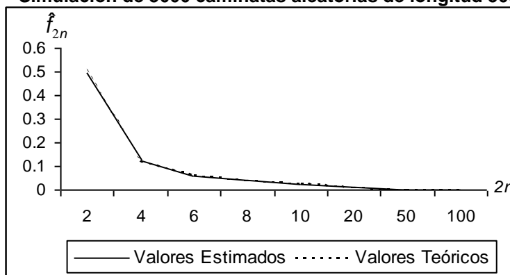
Gráfico 3.25 Caminatas Aleatorias Valores estimados para f_{2n} Simulación de 3000 caminatas aleatorias de longitud 5000
