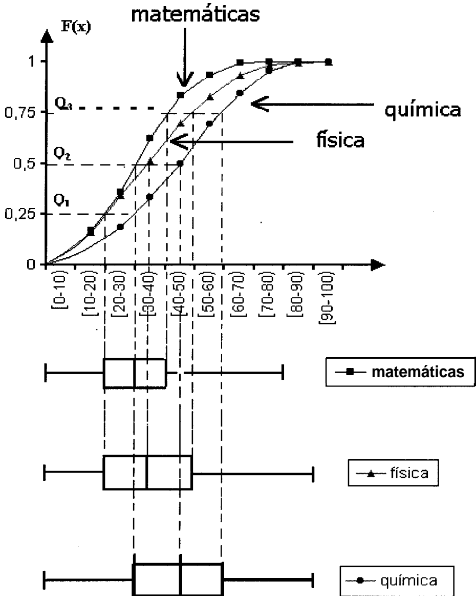
Figura 3.12 Admisión 1993: ingenierías Ojiva: nota total en matemáticas, física, y química correspondiente al primer examen de ingreso
