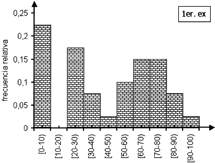
Figura 3.57 Admisión 1993: tecnología eléctrica-electrónica Histograma de frecuencias relativas: nota total en matemáticas
