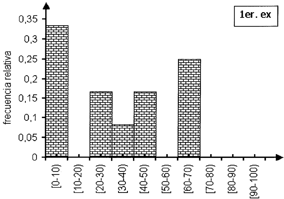
Figura 3.43 Admisión 1993: tecnología agrícola Histograma de frecuencias relativas: nota total en química
