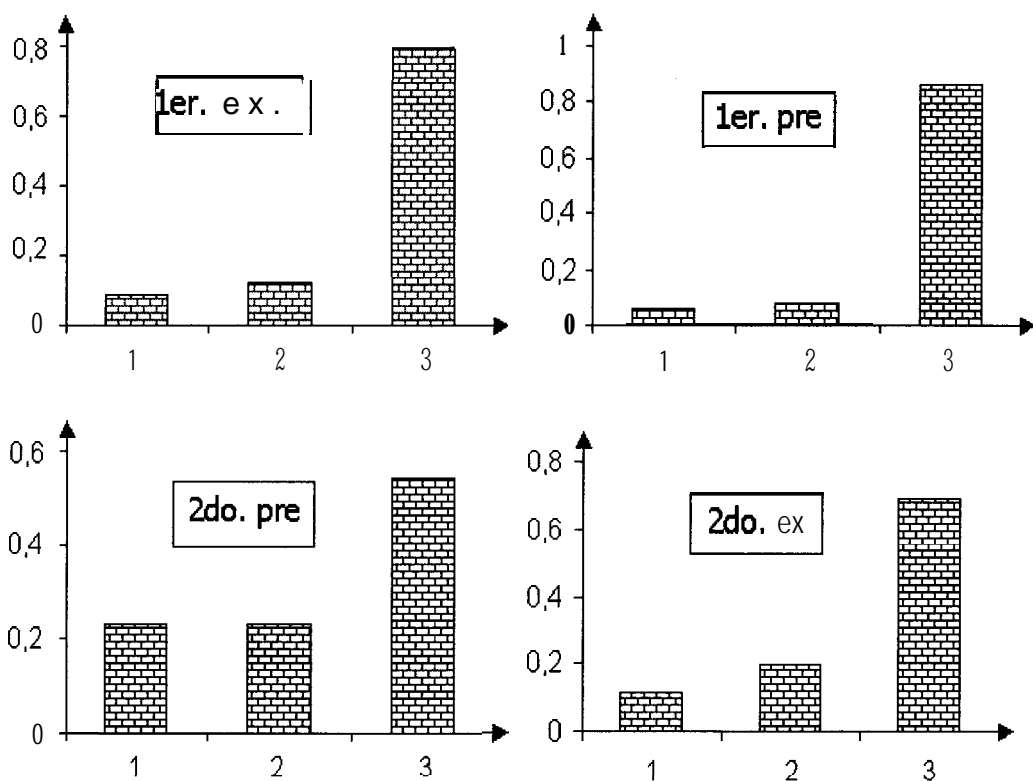
Figura 3.13 Admisión 1993: ingenierías Histograma de frecuencias relativas: Número de materias tomadas
