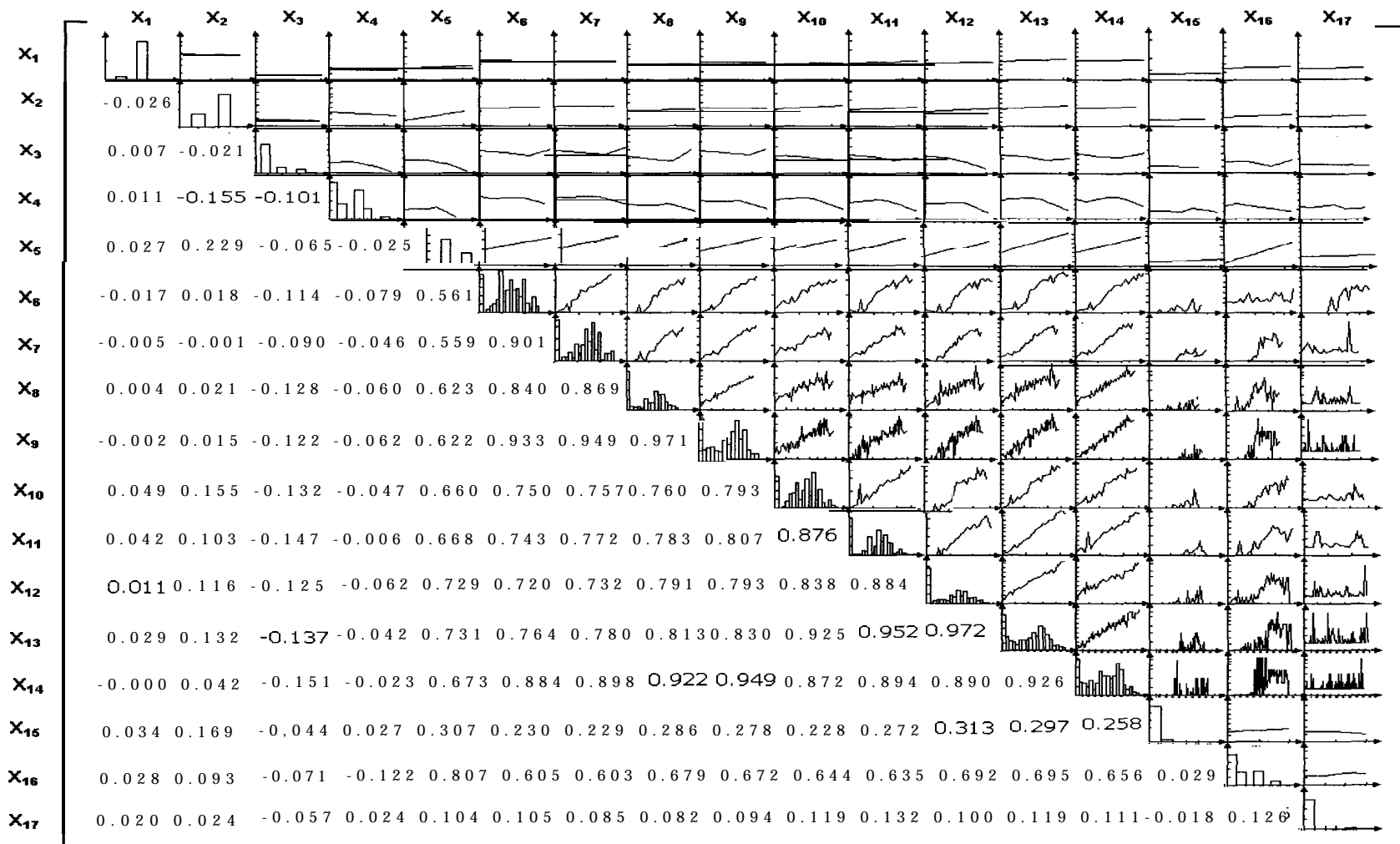
Figura 4.6 Admisión 1993: tecnologías Matriz de correlación entre las variables
