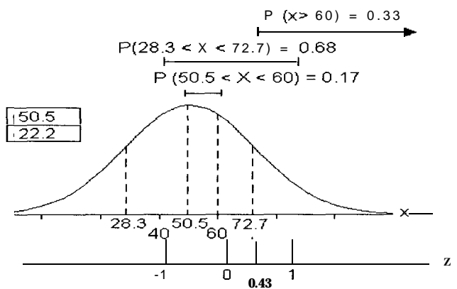
Figura 3.9 Admisión 1993: ingenierías - 2do. pre Función de densidad: nota total en física correspondiente de los colegios particulares
