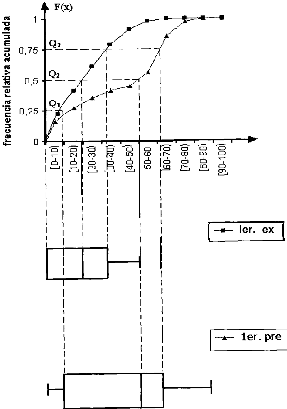
Figura 3.42 Admisión 1993: tecnología agrícola Ojiva: nota total en física
