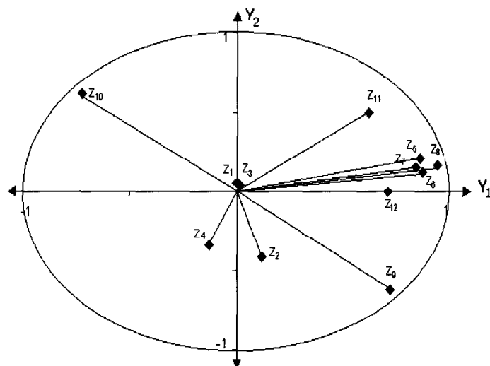
Figura 4.4 Admisión 1993: ingenierías Representación de las variables en el plano ( Y_1, Y_2 )
