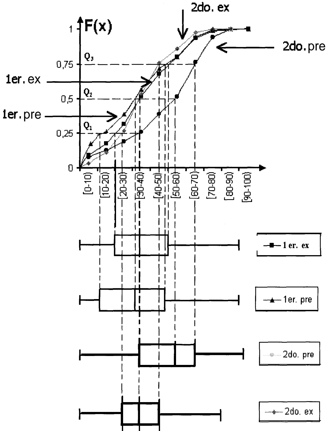
Figura 3.7 Admisión 1993: ingenierías Ojiva: nota total en física
