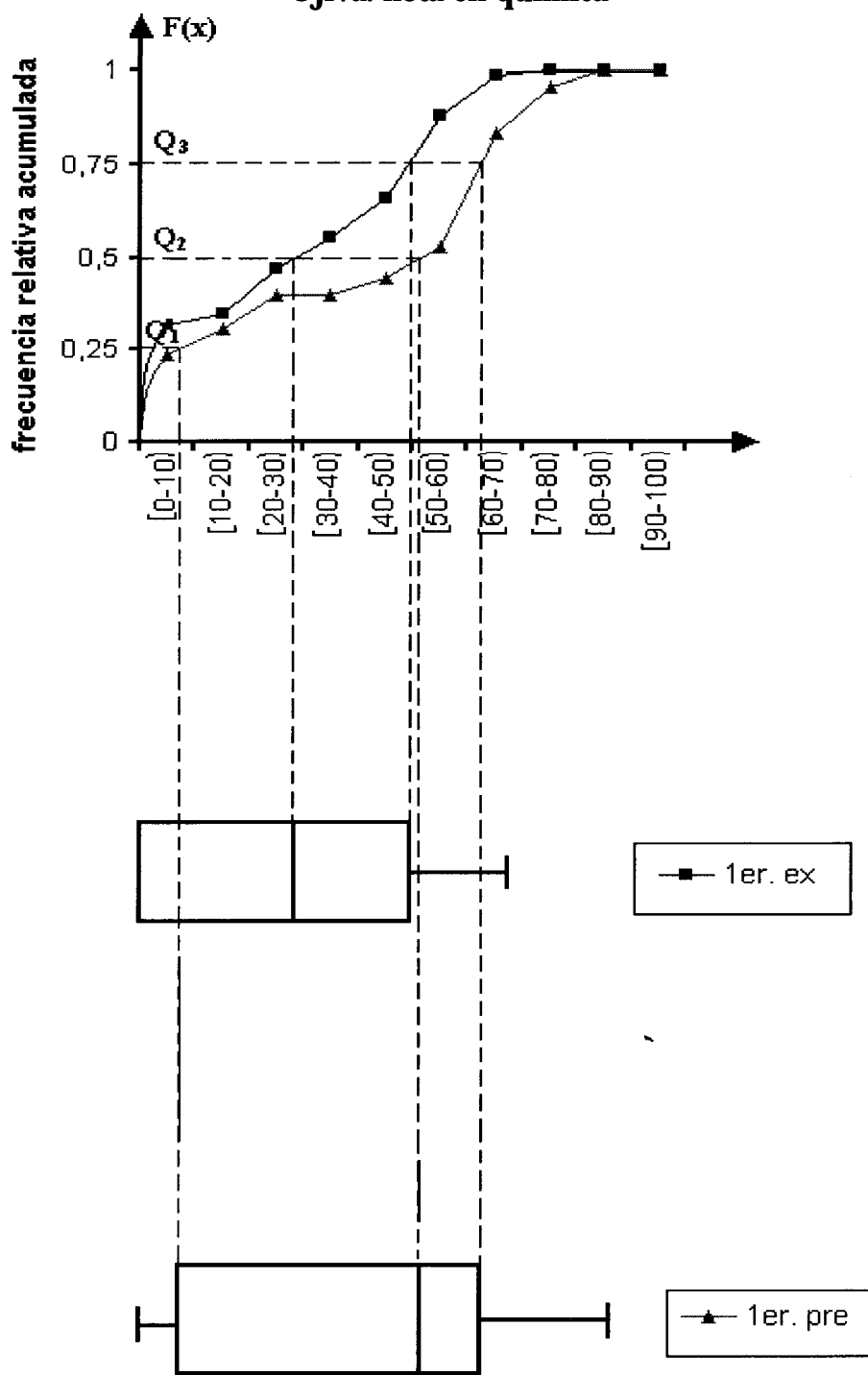
Figura 3.45 Admisión 1993: tecnología agrícola Ojiva: nota en química
