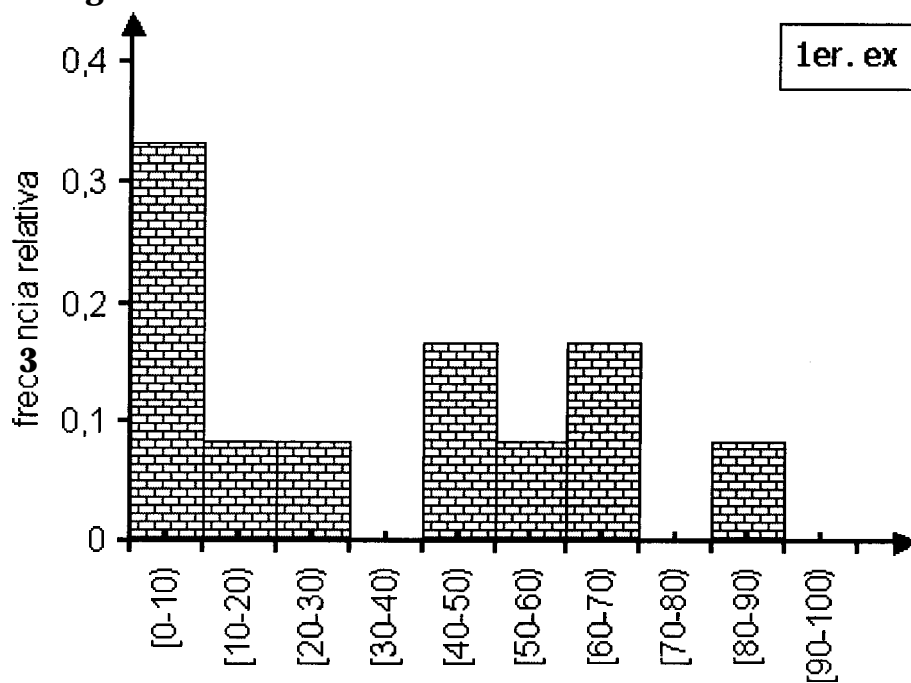
Figura 3.34 Admisión 1993: tecnología agrícola Histograma de frecuencias relativas: nota total en matemáticas
