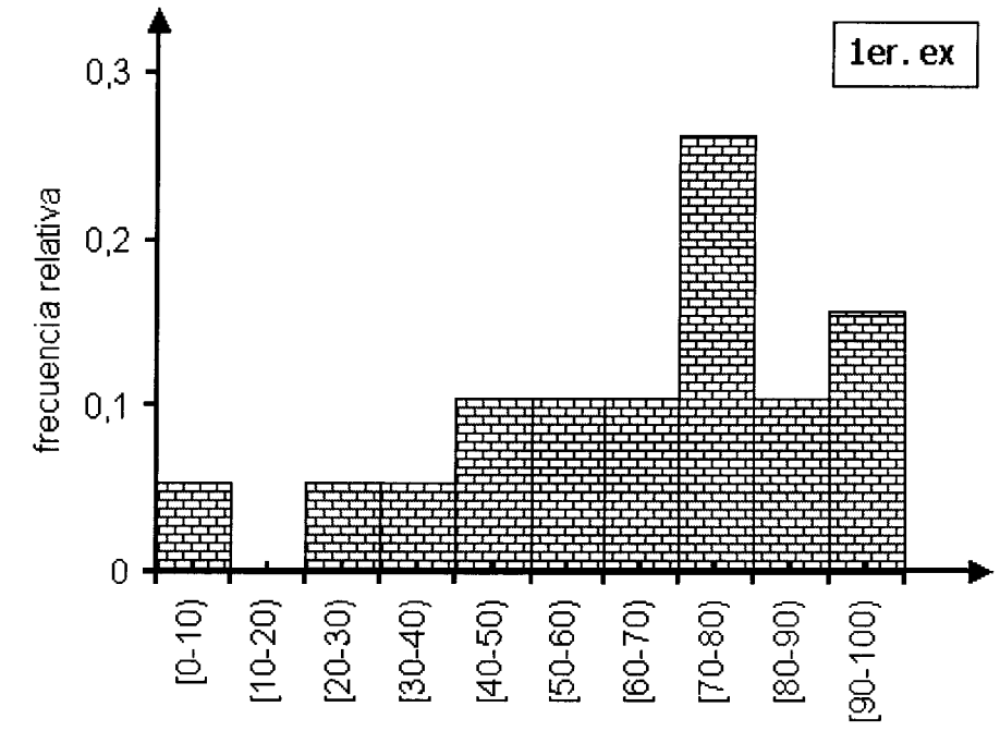
Figura 3.25 Admisión 1993: tecnología mecánica Histograma de frecuencias relativas: nota total en matemáticas
