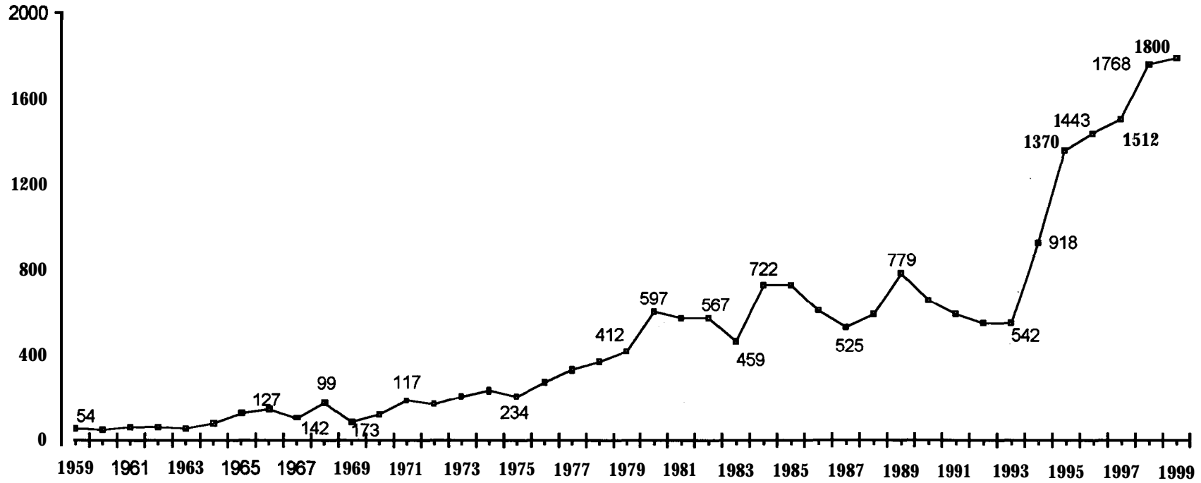
Figura 1.1 ESPOL: Ingreso de estudiantes 1959 - 1999
