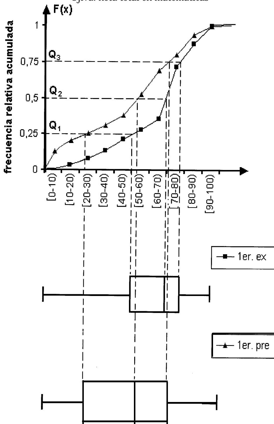
Figura 3.27 Admisión 1993: tecnología mecánica Ojiva: nota total en matemáticas
