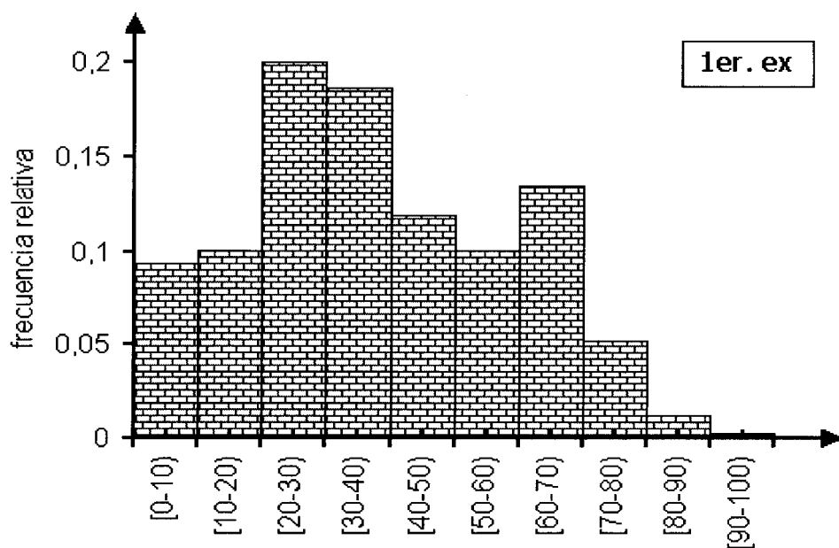
Figura 3.5 Admisión 1993: ingenierías Histograma de frecuencias relativas: nota total en física
