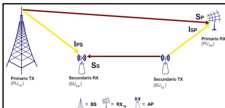
Figura 3.2 Caracterización de interferencias para reuso del espectro
