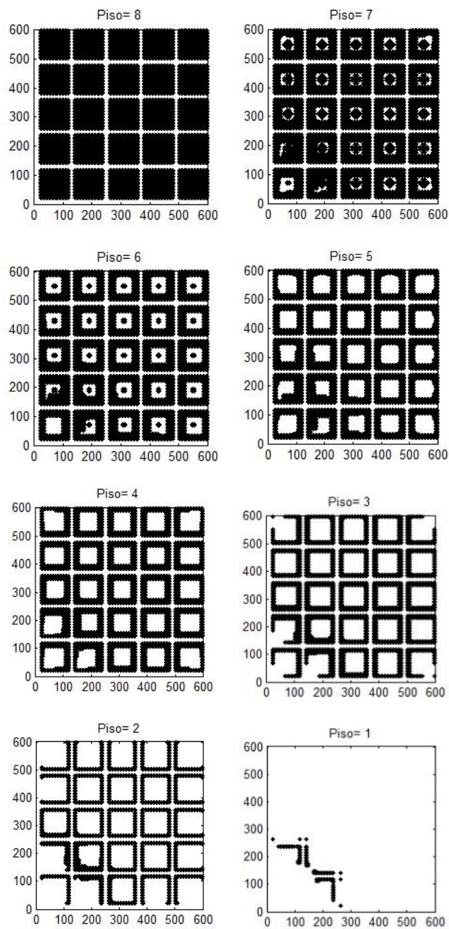
Figura 4.4 Resultado total de disponibilidad para edificios de 8 pisos
