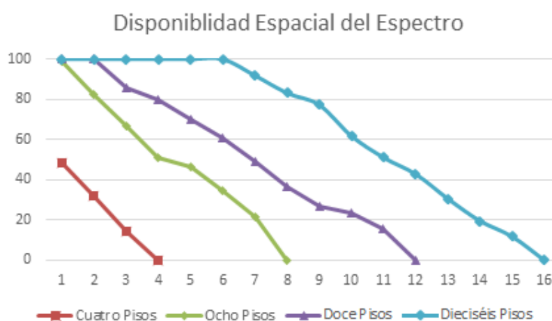
Figura 4.9 Disponibilidad Espacial del Canal para Escenarios de Varios Pisos
