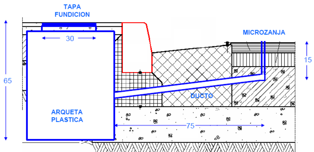
Fig. 4.21 Modelo para Arquetas que alojarán las cajas de empalmes
