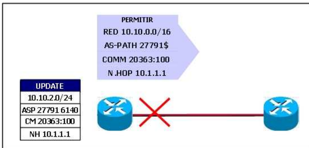
Fig. 2-43.- Filtros BGP
