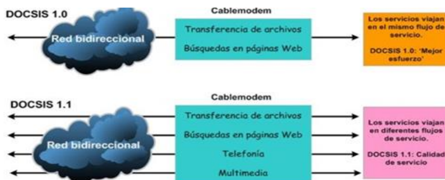
Figura 3.4. Flujos de servicio en DOCSIS 1.x. [19]
