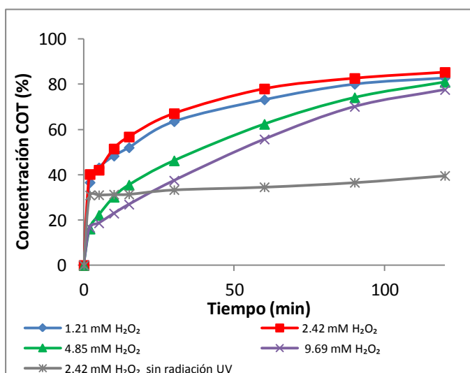
Gráfico 19. Reacción foto-Fenton utilizando \text{C}_0 : 0.207 mM QCL, 0.90 mM \text{Fe}^{2+} y diferentes concentraciones de \text{H}_2\text{O}_2
