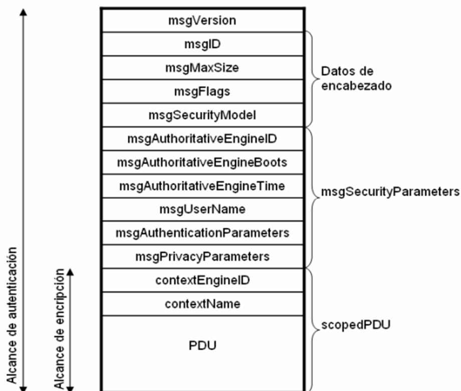
Figura 2.13 – Formato del mensaje SNMPv3 con el campo msgSecurityParameters . [23]
