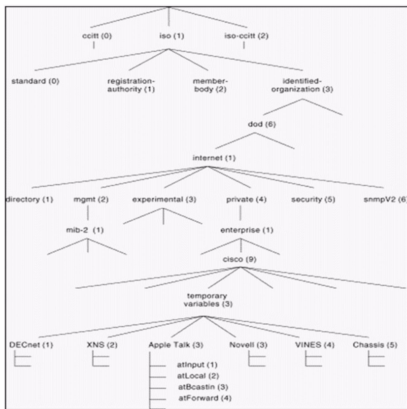
Figura 2.4 – Ejemplo de árbol MIB. [7]
