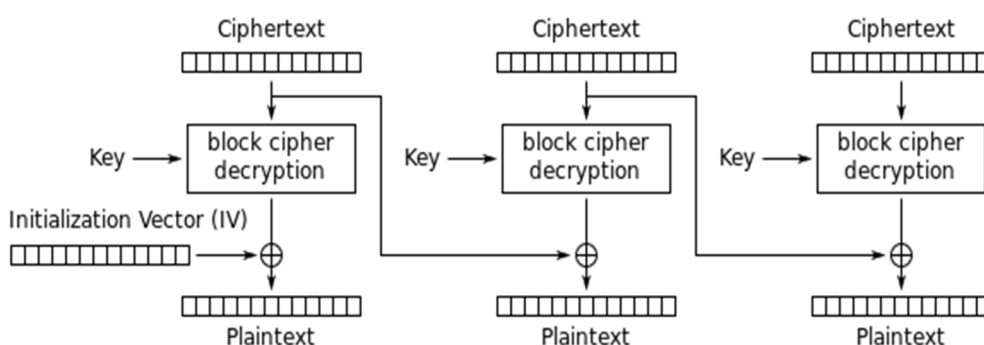
Figura 2.7 - Descifrado DES en modo Encadenamiento de Bloques de Cifrado. [28]
