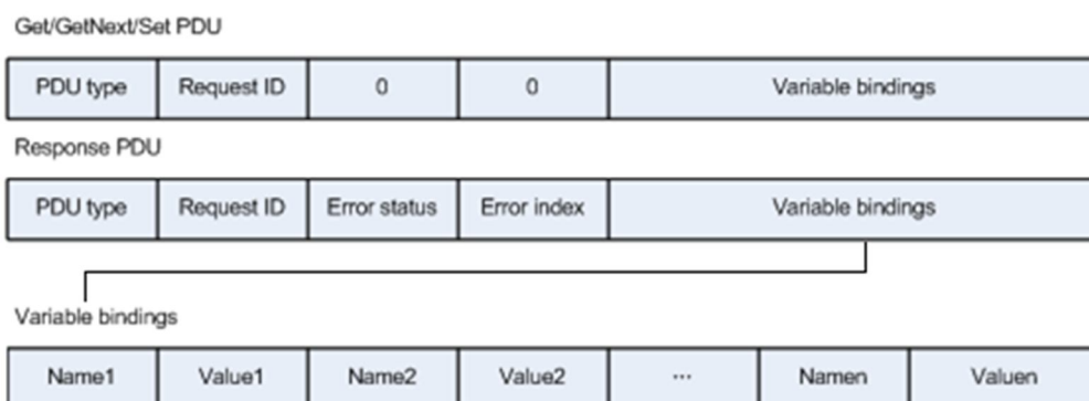
Figura 2.10 – Formato de la PDU v1 y v2. [5]
