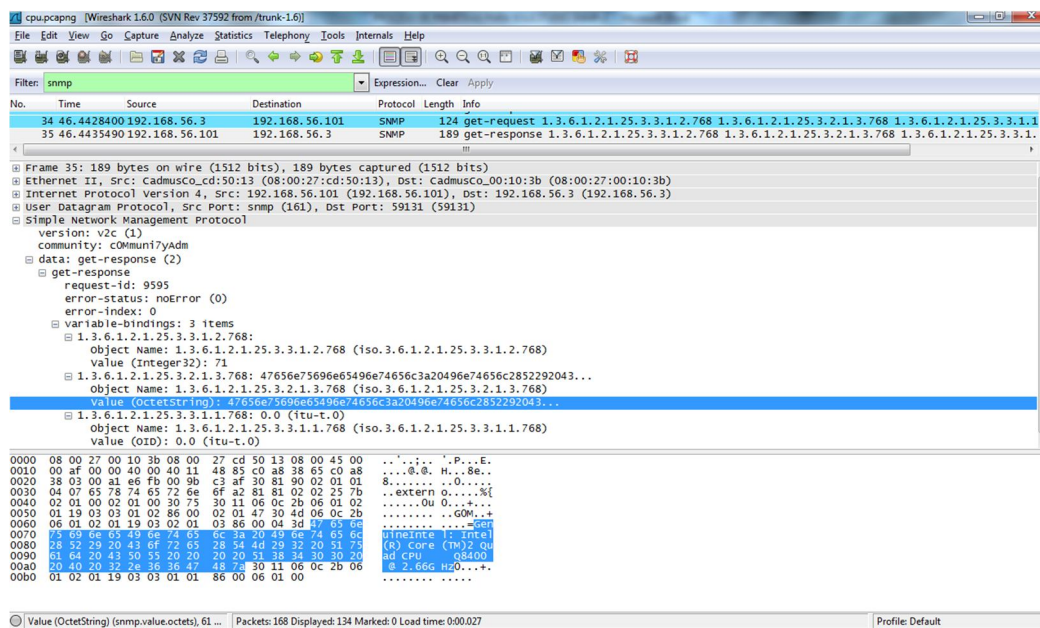
Figura 4.7- Paquete respuesta datos de uso CPU - v2
