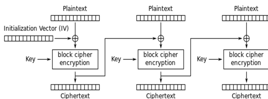
Figura 2.6 - Cifrado DES en modo Encadenamiento de Bloques de Cifrado. [28]
