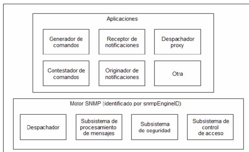
Figura 2.5 - Diagrama de una entidad SNMPv3. [23]
