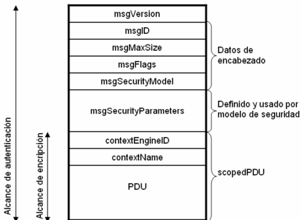
Figura 2.12 – FORMATO DE MENSAJE SNMPv3. [23]
