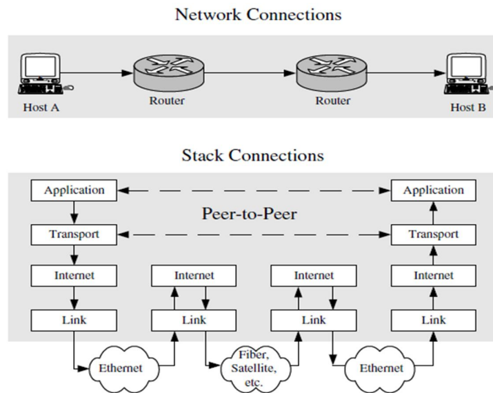
Figura 2.2 – Modelo de referencia TCP/IP. [4]
