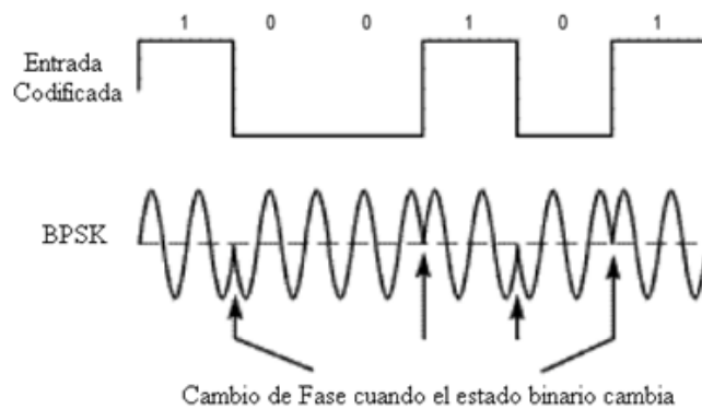
Figura 2.11. Ejemplo de la Modulación BPSK [8]
