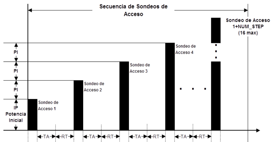
Figura 3.6. Escalera de Sondeos de Acceso.
