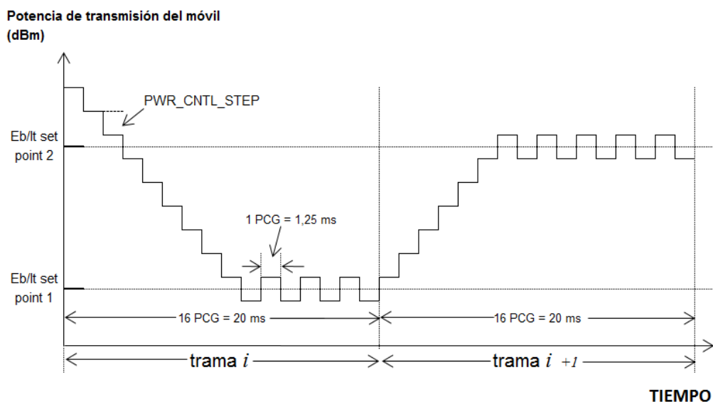
Figura 3.14 Comportamiento de la potencia de transmisión de un móvil según el valor objetivo de E_b/I_t
