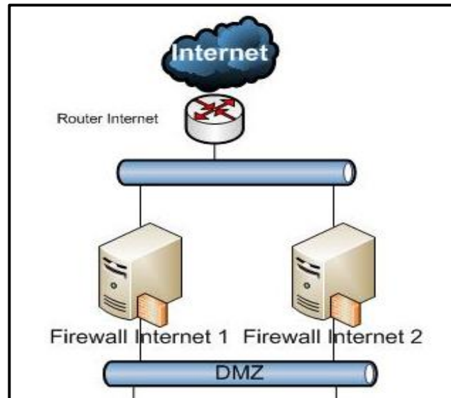
Figura 4.45. Arquitectura de una DMZ “Back to Back” con tolerancia a fallos [39]
