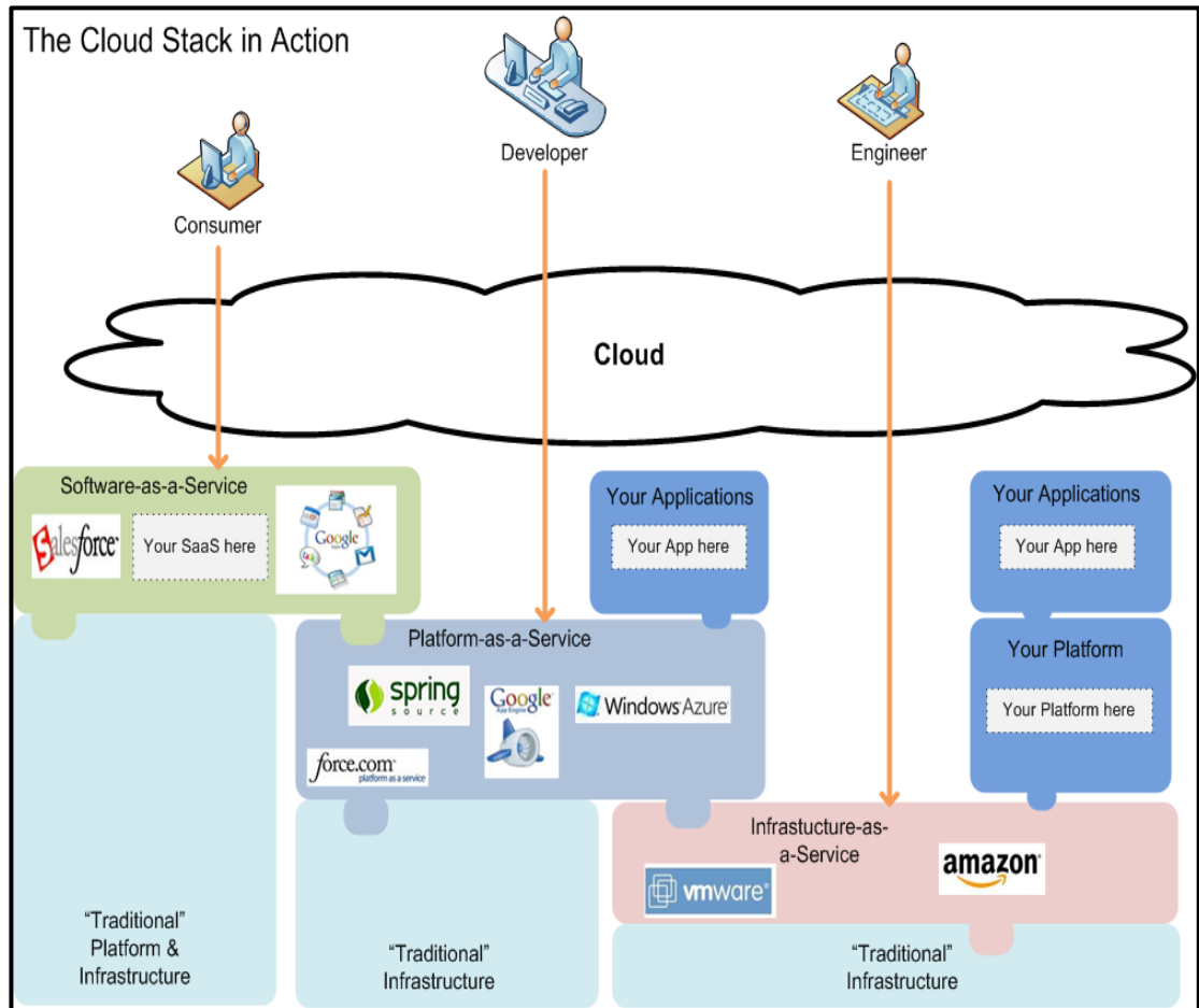
Figura 2.14. Modelo de despliegue CloudStack [27].
