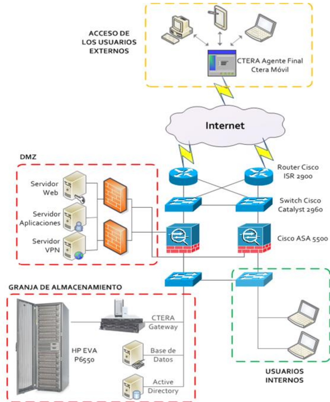
Figura 4.49. Diseño de arquitectura CTERA y HP EVA [31] [46]
