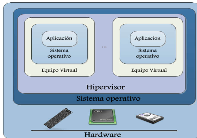
Figura 2.15. Arquitectura Con Virtualización [21].
