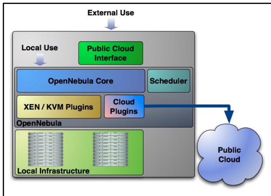
Figura 2.12. Diagrama de arquitectura OpenNebula [26].
