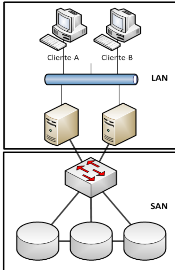
Figura 3.19. Red de área de almacenamiento [20].
