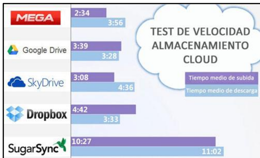
Figura 3.27. Velocidad de los servicios de almacenamiento [18].
