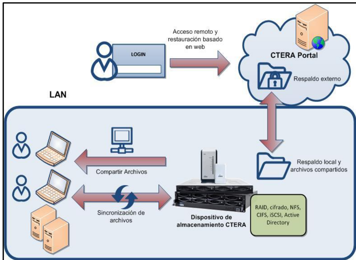
Figura 4.32. Funcionamiento de CTERA [36].
