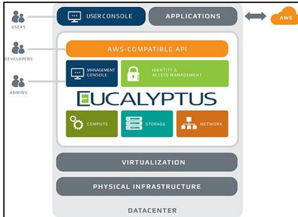
Figura 2.13. Arquitectura de Eucalyptus [26].
