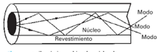
Fig. 5.5 Fibra Óptica Multimodo [15]
