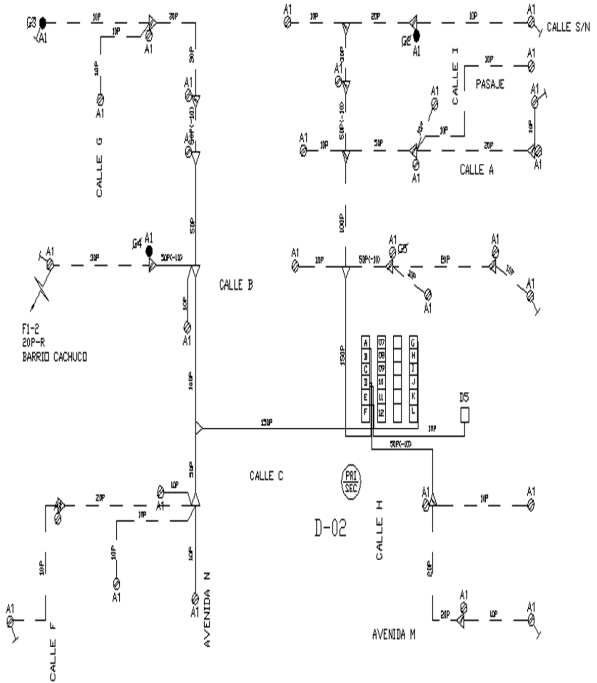
ESQUEMA DE EMPALMES DISTRITO 02
