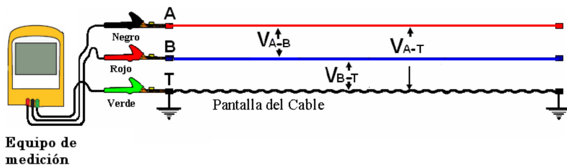
Fig. 5.33 Voltaje Inducido [19]
