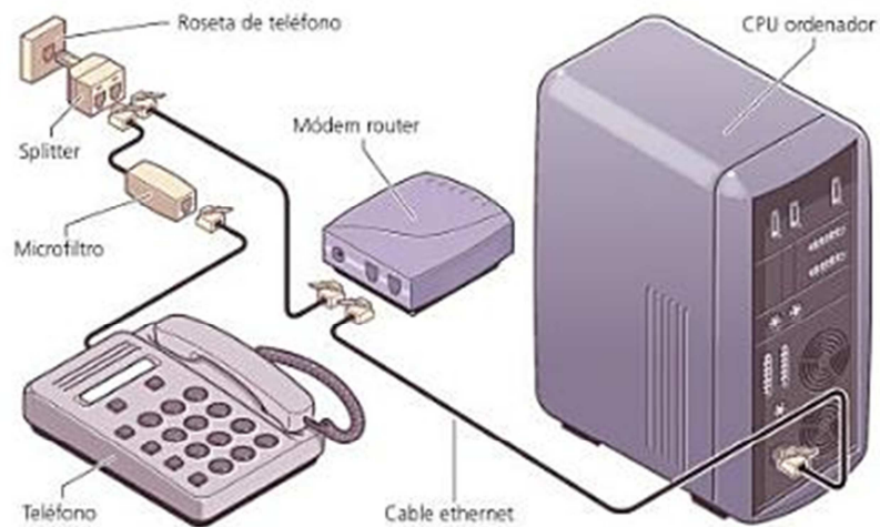
Fig. 3.2 Conexión ADSL [5]
