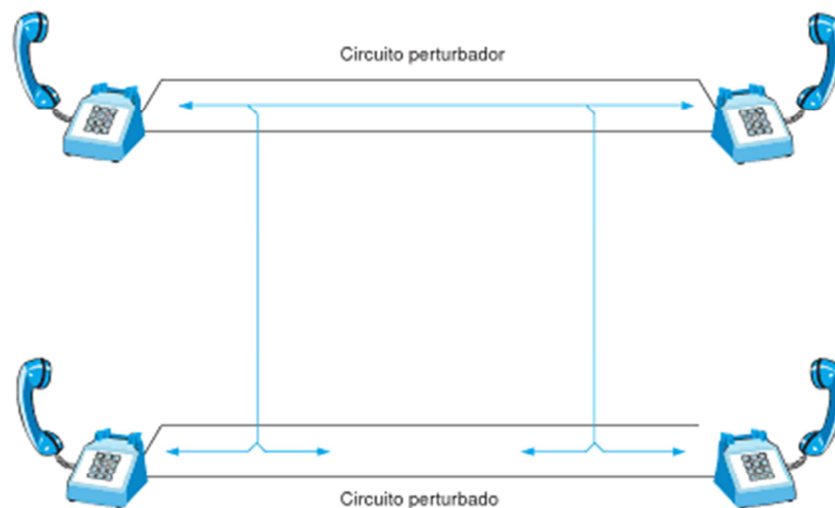
Figura 4.13. Diafonía.
