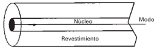
Fig. 5.6 Fibra Óptica Monomodo [15]
