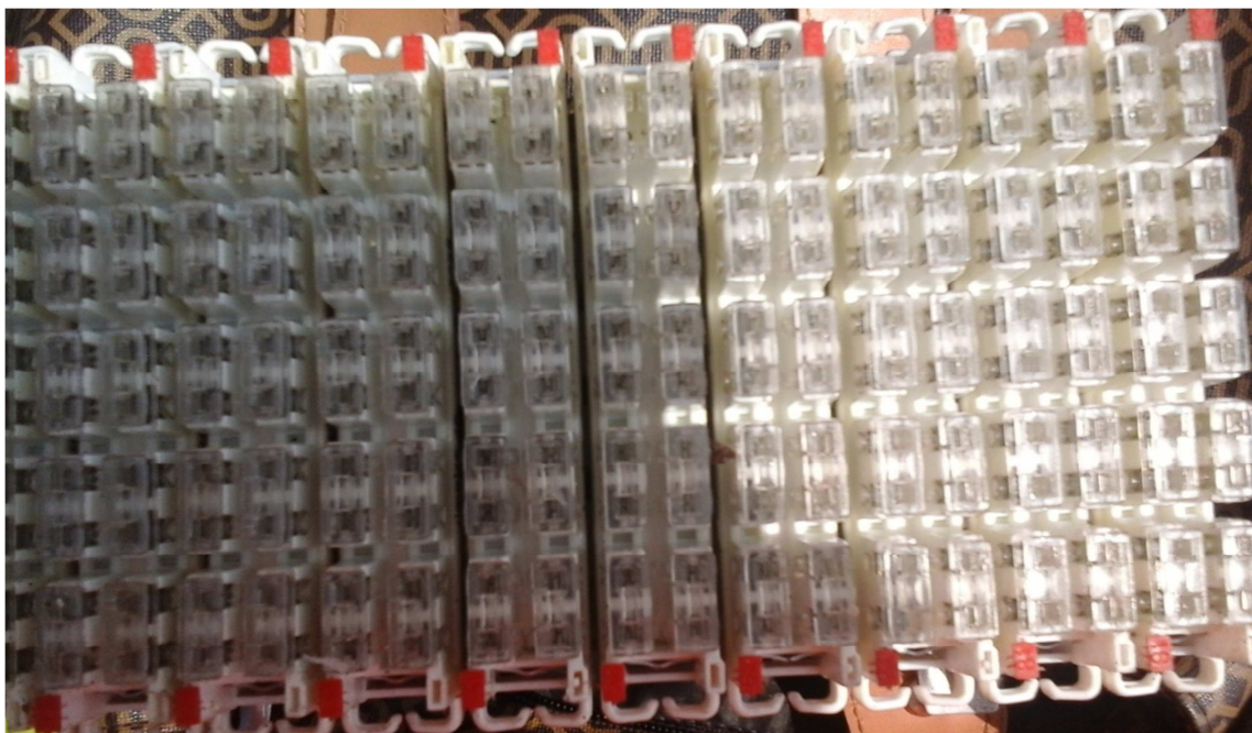
Fig. 5.24 Bloque de Conexión de 100 pares
