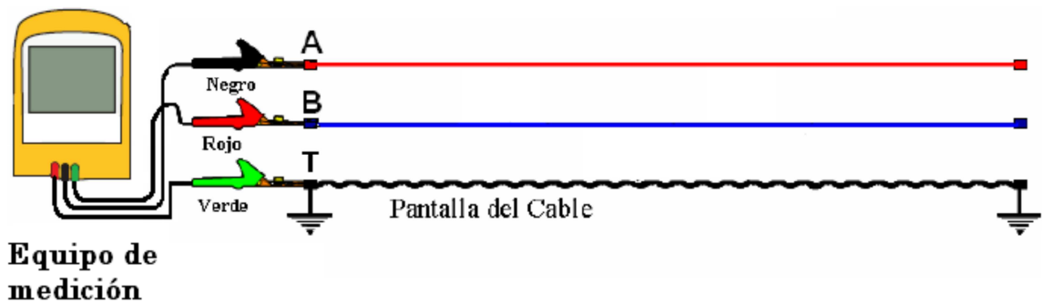
Fig. 5.39 Ruido a Tierra [19]
