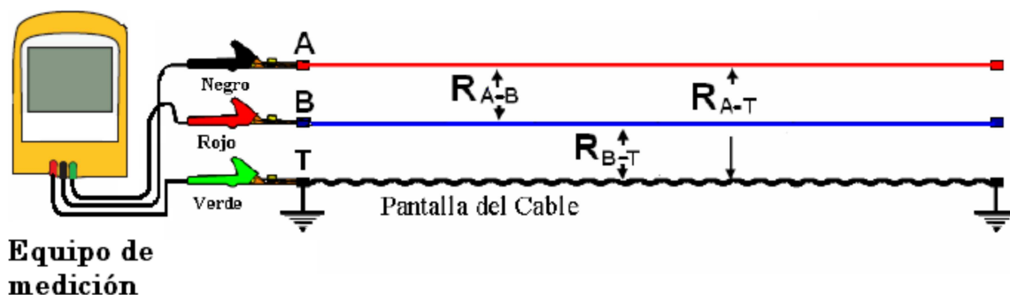
Fig. 5.35 Resistencia de Aislamiento en una Red Nueva [19]
