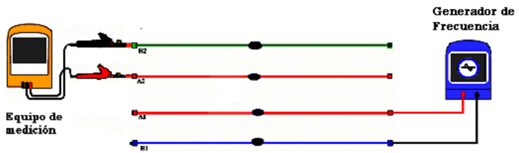
Fig.5.41 Diafonía [19]
