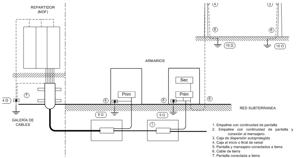
Fig. 4.1 Planta Externa
