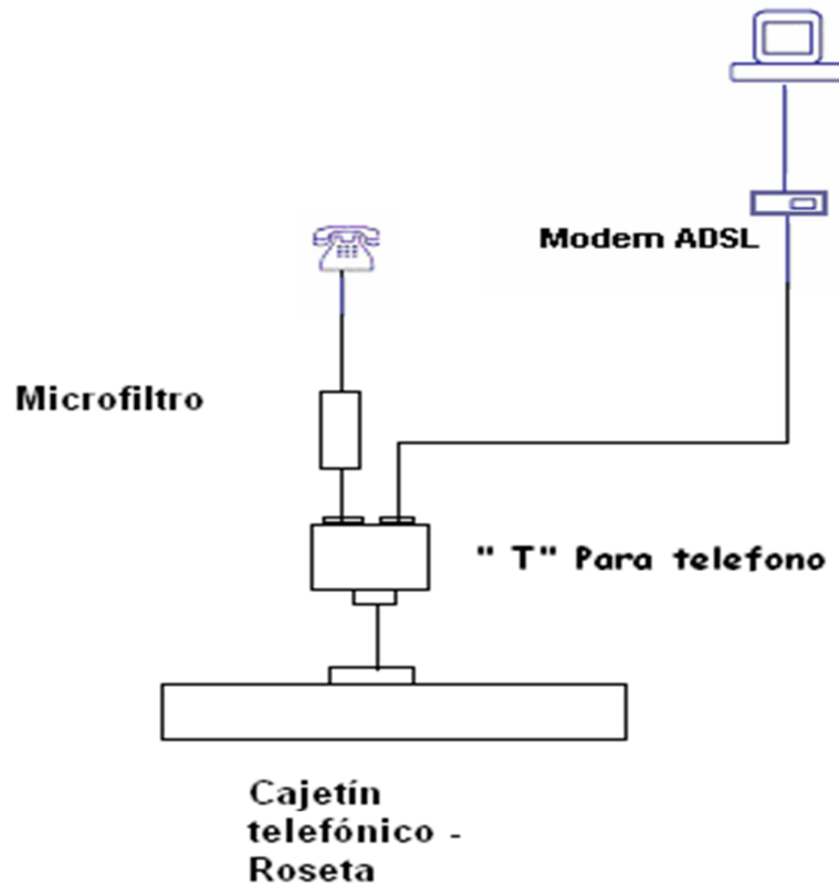
Fig. 3.1 Conexión en Abonado ADSL [5]
