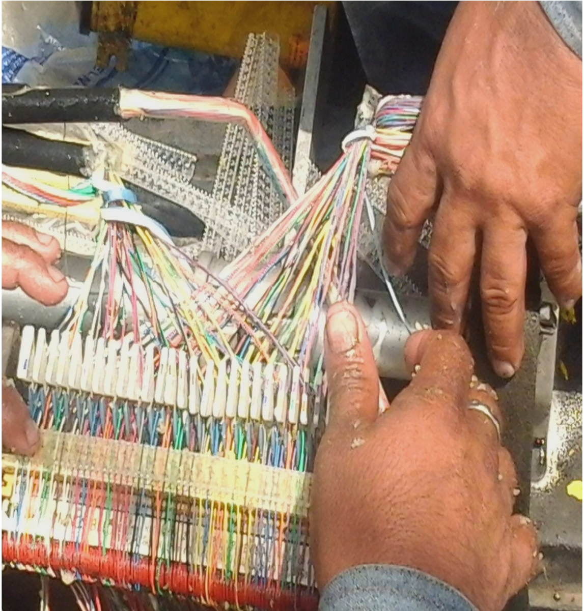
Fig. 5.26 Empalmado
