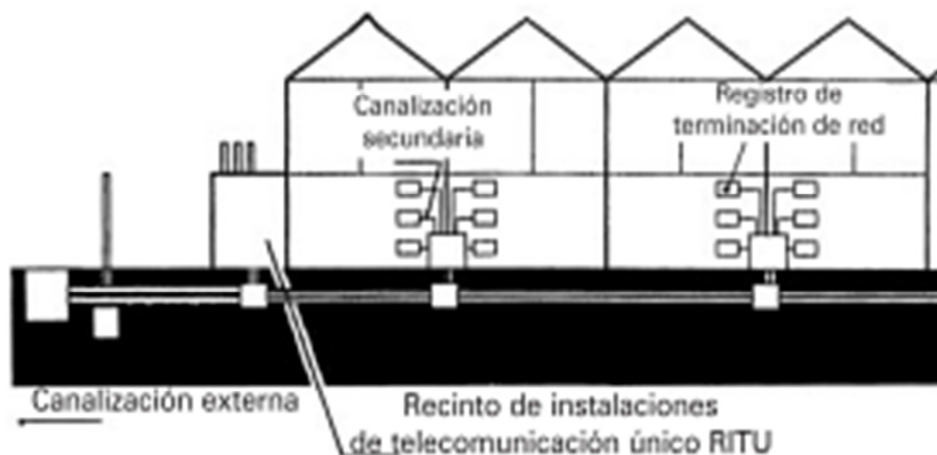
Fig. 5.28 Instalación de Cajas Dispensoras [18]
