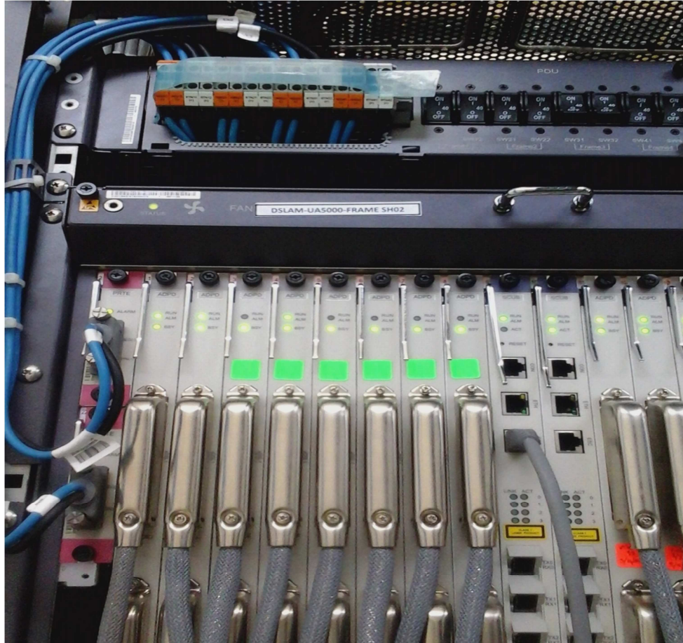
Fig. 5.9 Dslam Huawei
