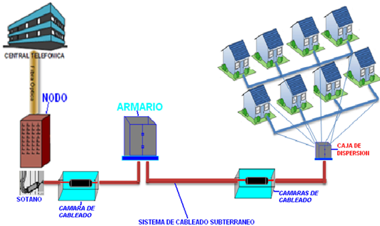
Fig. 5.3 Planta Externa
