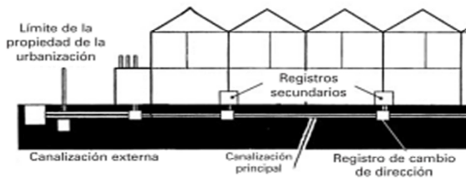
Fig. 5.20 Canalizaciones [18]
