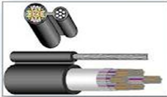
Fig. 5.12 Cable eKKx [18]
