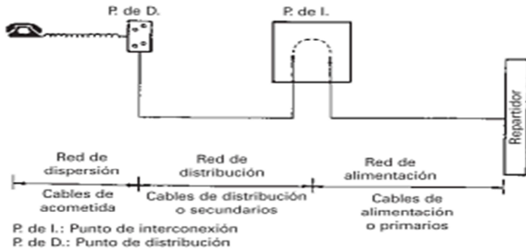
Fig. 5.1 Diseño de Planta Externa
