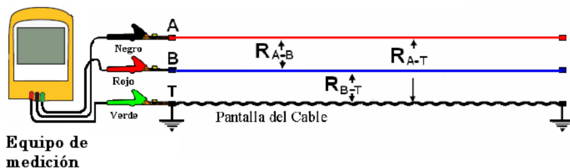
Fig. 5.34 Resistencia de Aislamiento [19]
