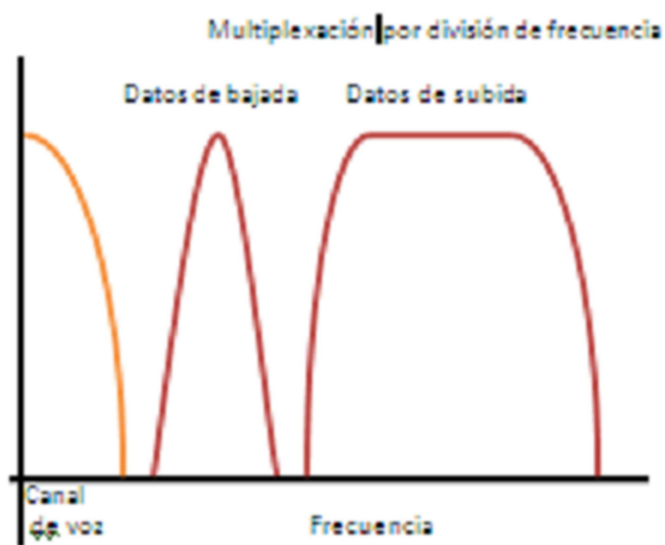
Fig. 2.1 Multiplexación por división de frecuencia [2]
