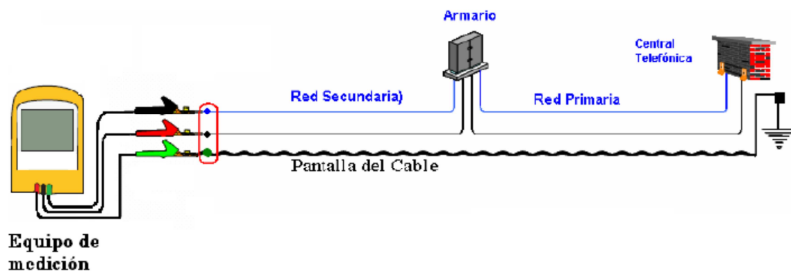
Fig. 5.37 Continuidad de Pantalla [19]
