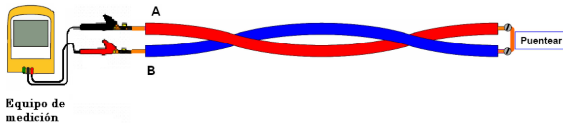
Fig. 5.36 Resistencia de Bucle [19]
