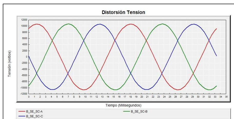
Figura 2.12: Distorsión de tensión en la barra principal 13,2 kV Caso 6.
