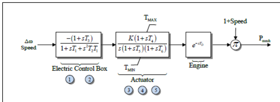
Figura 3.10: Modelo del Gobernador DEGOV. [21]
