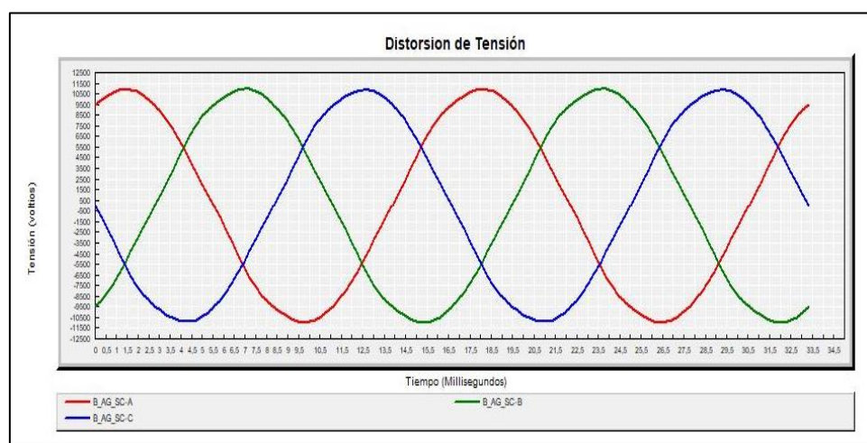
Figura 2.11: Distorsión de tensión en la barra aerogeneradores 13,2 kV Caso 6.
