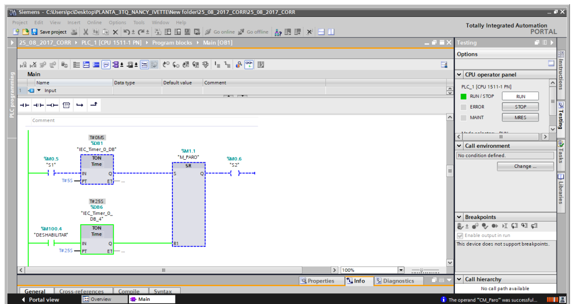
Figura 4.25: Programación para el sistema de paro (3).
