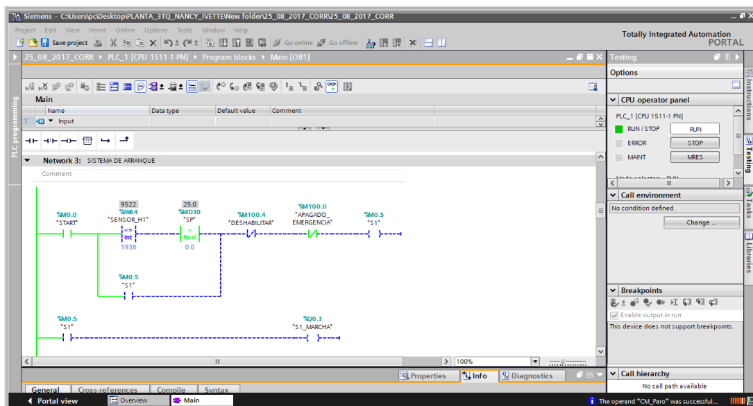
Figura 4.23: Programación para el sistema de paro (1).
