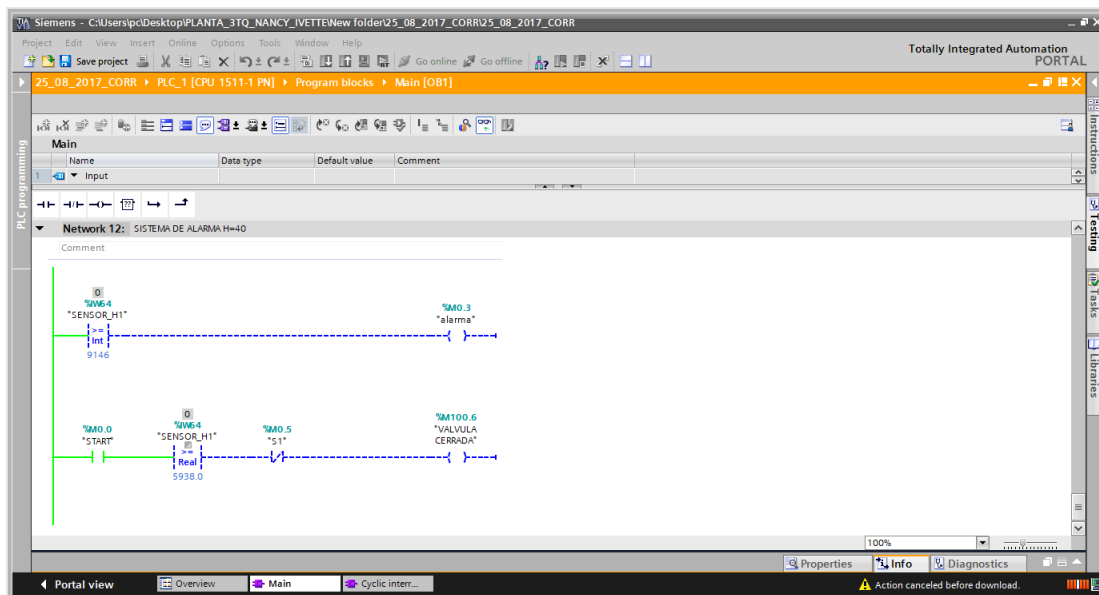
Figura 4.28: Programación para el sistema de alarmas (1).
