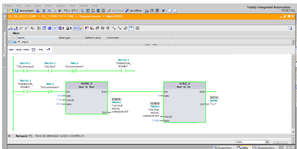
Figura 4.15: Programación para el sistema de arranque (6).
