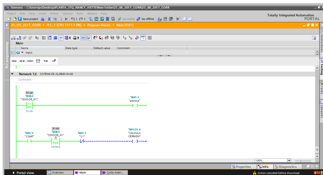
Figura 4.29: Programación para el sistema de alarmas (2).
