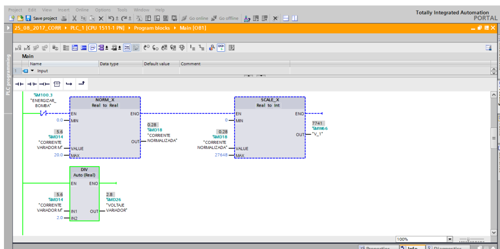
Figura 4.18: Programación para el sistema de control (3).
