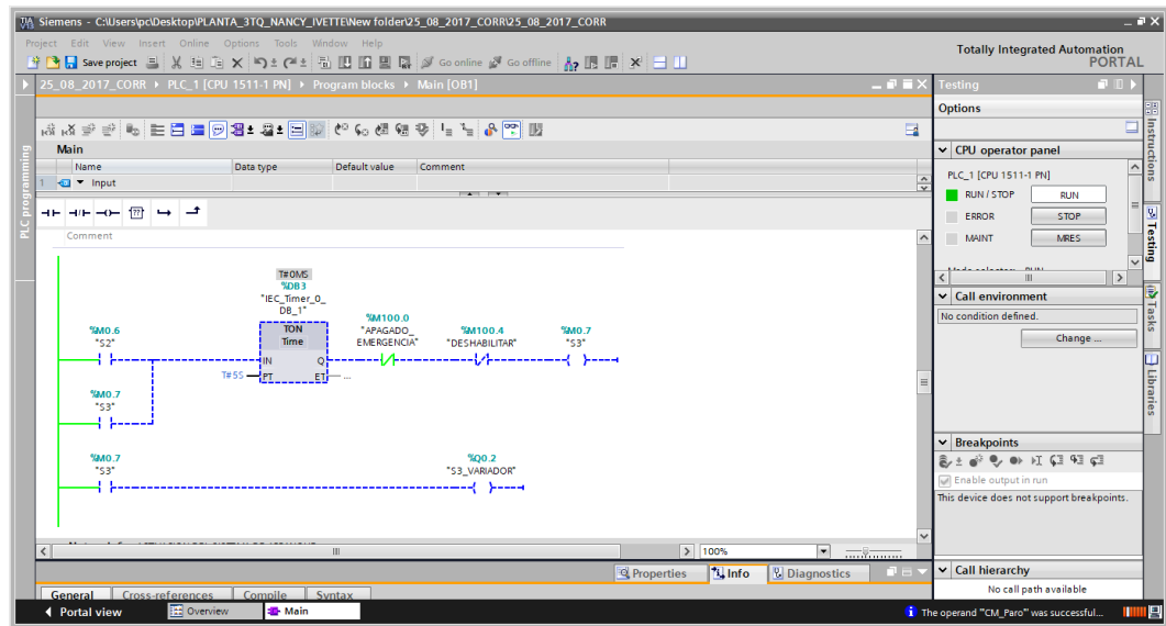
Figura 4.24: Programación para el sistema de paro (2).
