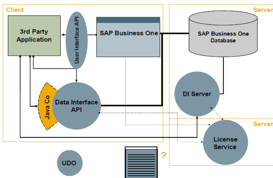
Figura 2. 12: Componentes SDK SAP BO
