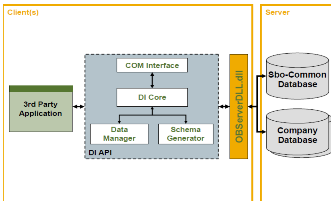
Figura 2. 14: Arquitectura de Software de DI API
