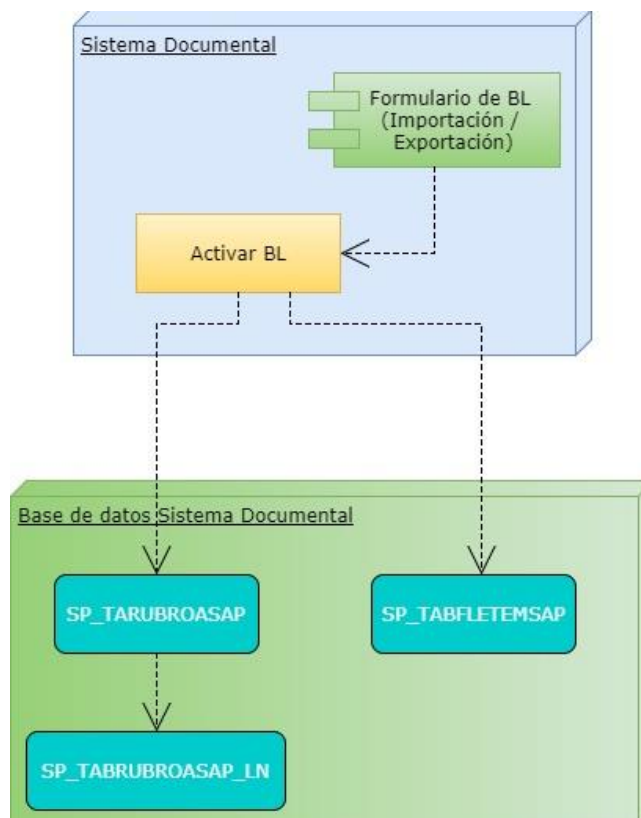
Figura 5. 6: Diagrama de ejecución de scripts de Generación de Gastos Locales y Fletes
