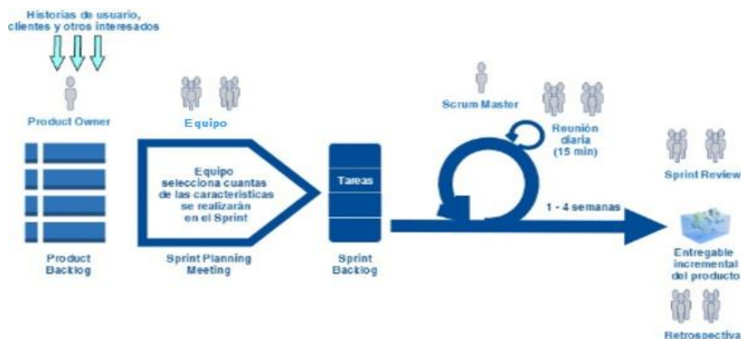
Figura 2. 6: Proceso SCRUM
