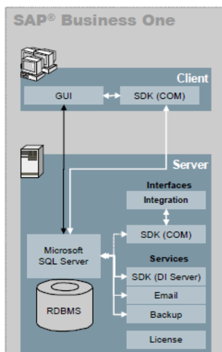
Figura 2. 11: Tecnología e interfaz de SAP BO
