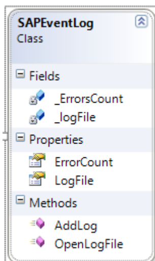
Figura 5. 21: Clase SAPEventLog
