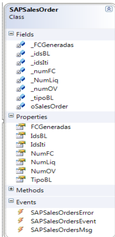
Figura 5. 18: Clase “SAPSalesOrder”
