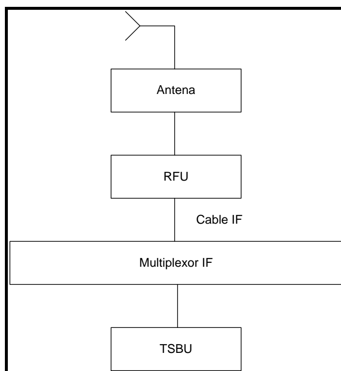
FIGURA 3.12: Estación Terminal
