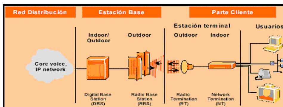
FIGURA 1.67: Esquema de Red LMDS
