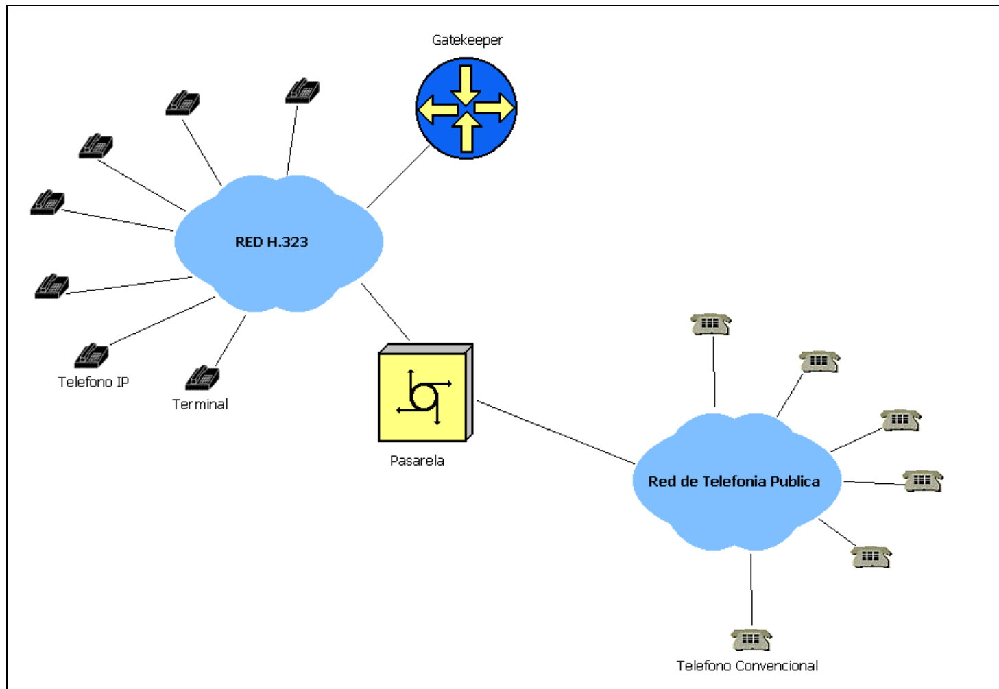
Figura 2.1 Arquitectura general de una red H.323
