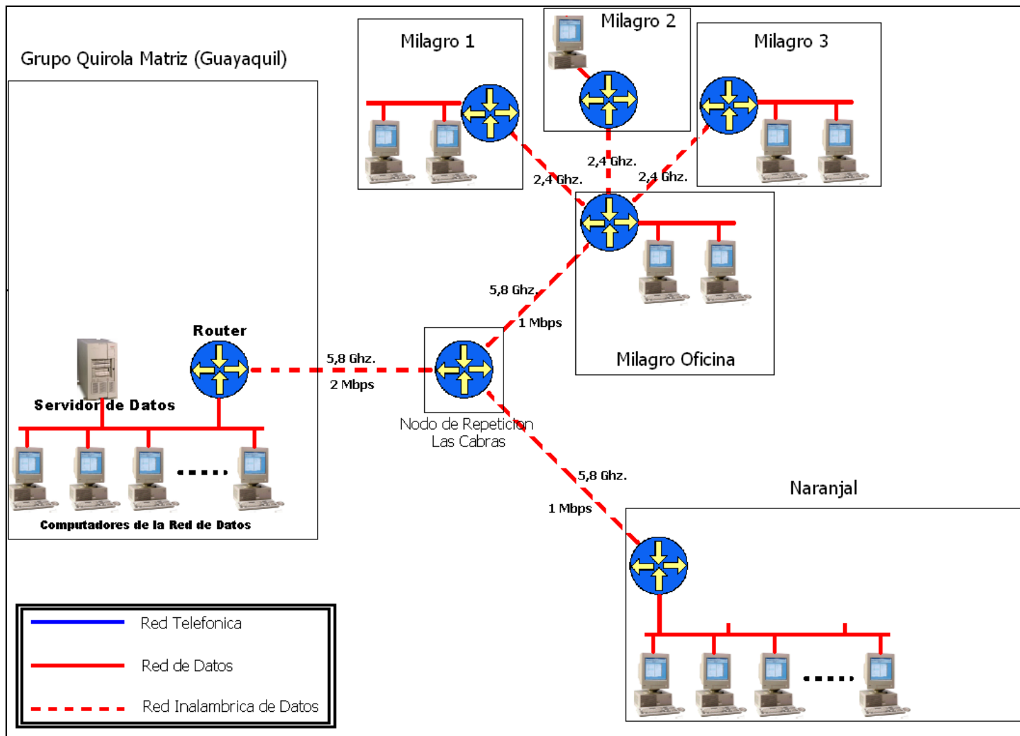
Figura 3.15 Sistema de comunicación de datos
