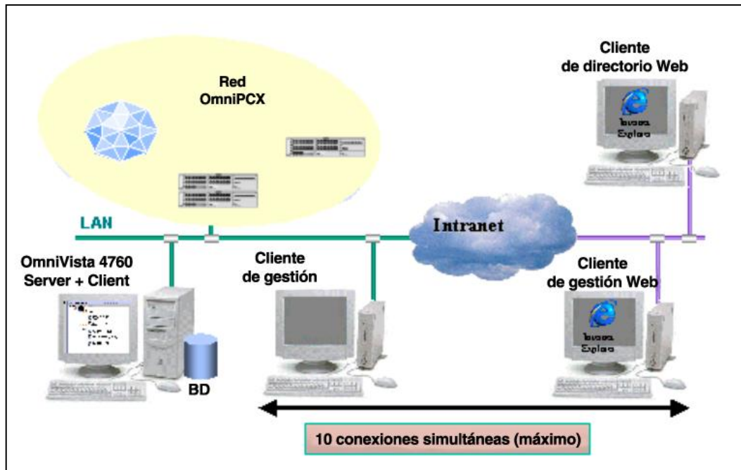
Figura 5.2 Esquema de arquitectura global
