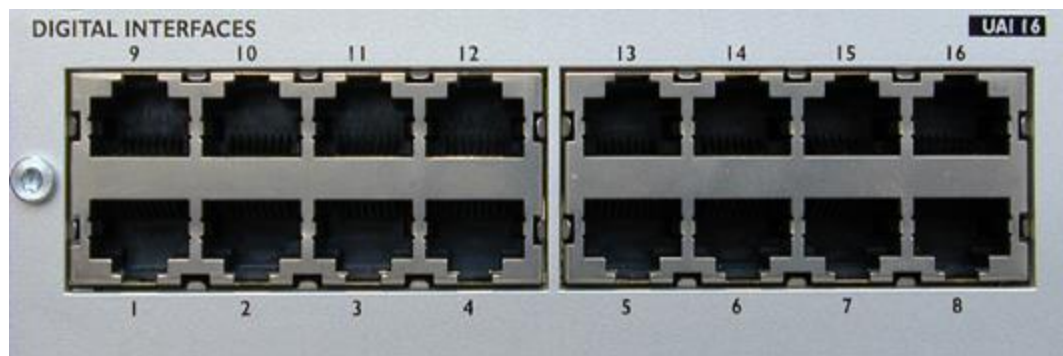
Figura 3.7 Tarjetas UAI-X
