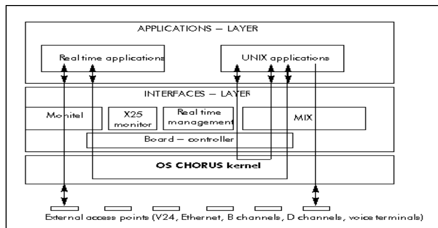
Figura 3.4 Arquitectura Lógica
