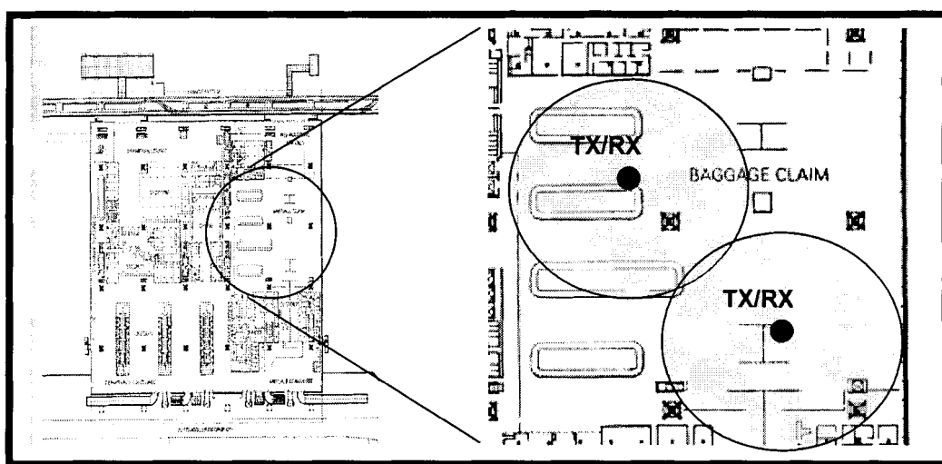
Figura 2.36.- Ubicación sugerida de más de una antena Omni
