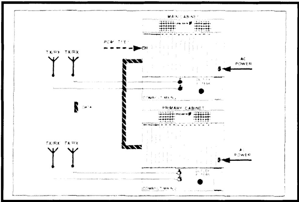
Figura 2.29.- Sectorizada / 2 Gabinetes – 2 Tx/Rx
