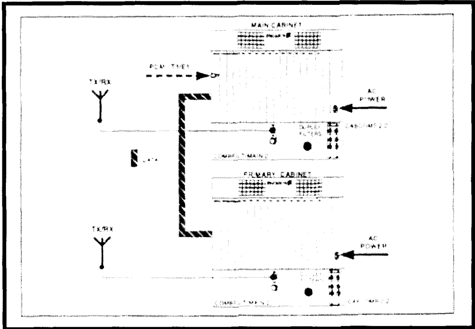
Figura 2.27.- Sectorizada / 2 Gabinetes – 1 Tx/Rx por sector
