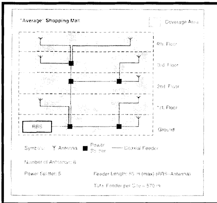
Figura 2.43.- Sistema distribuido de antenas
