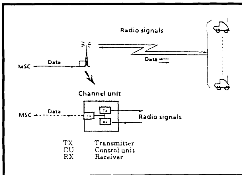
Figura 1.7.- Canal de Control
