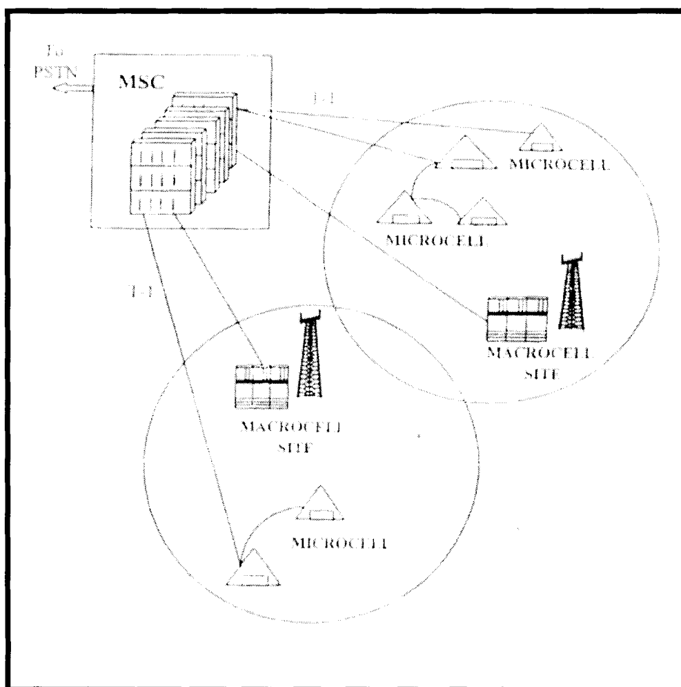
Figura 2.1.- Microceldas en un sistema celular básico
