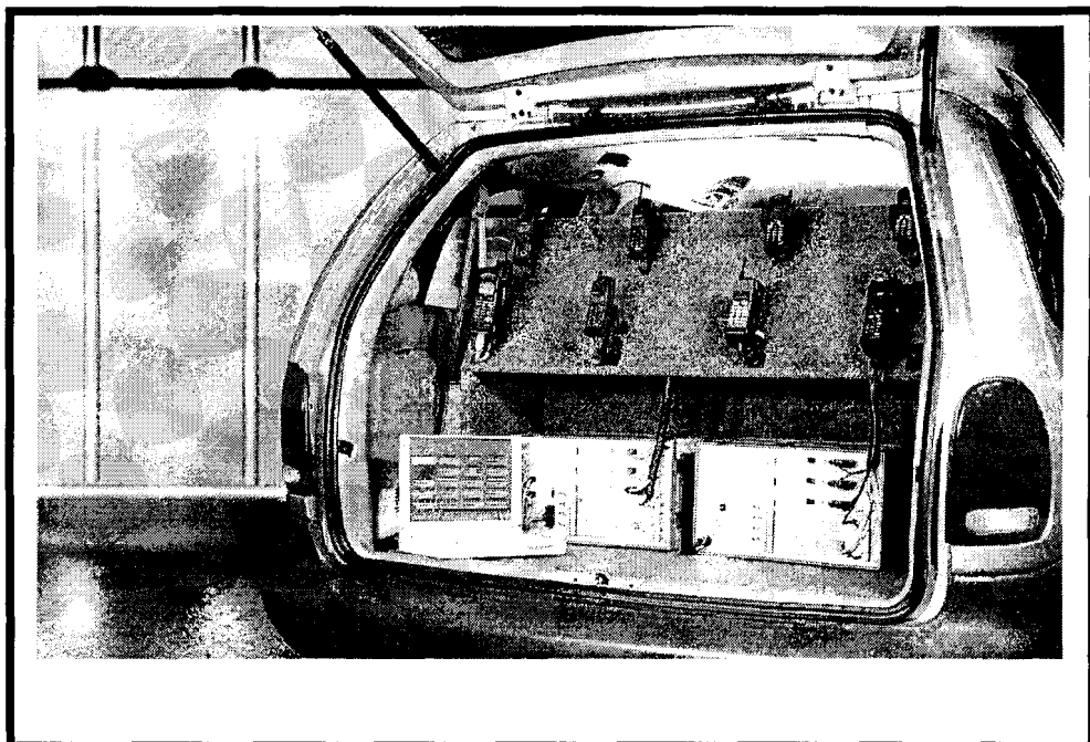
Figura 2.10.- Equipo para realizar mediciones en exteriores
