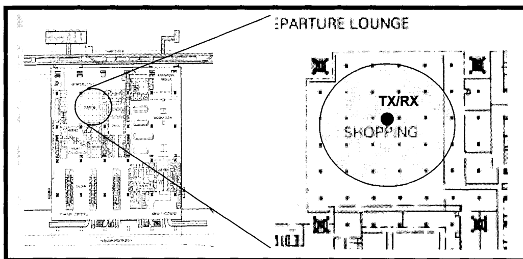
Figura 2.35.- Ubicación de antena Omni en un área regular
