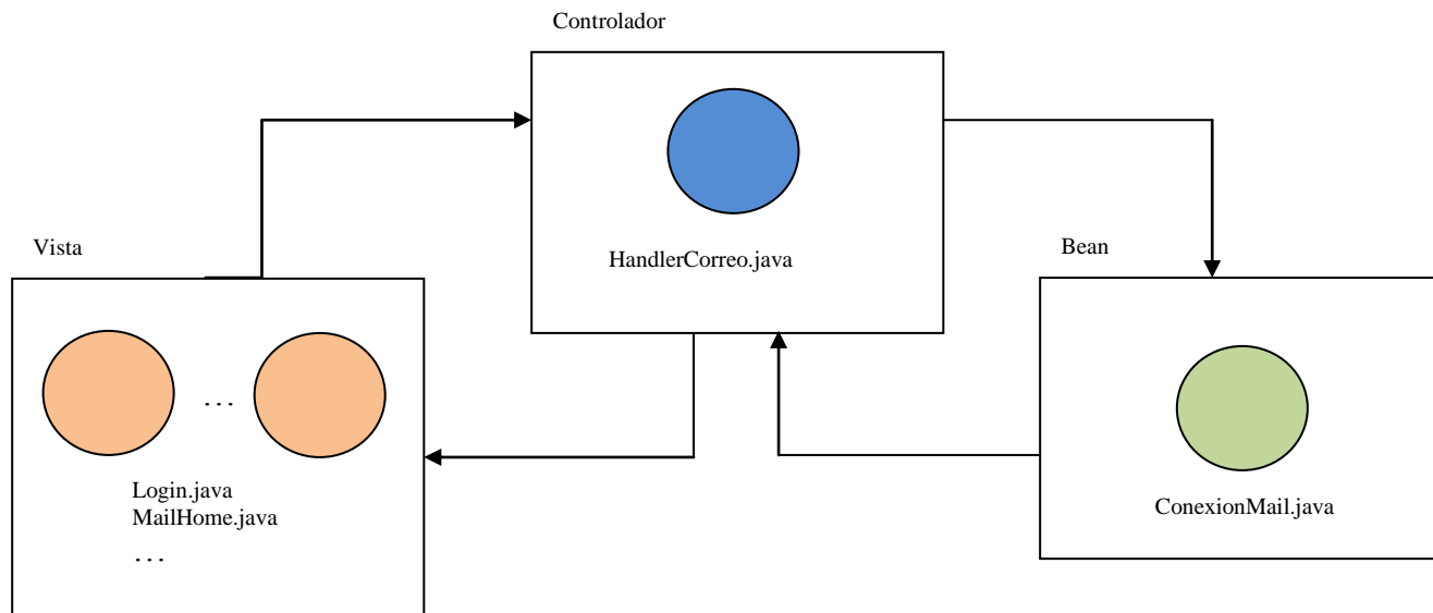
Modelo MVC del módulo del Correo
