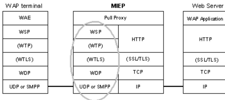
Figura 3.5.- Modelo del funcionamiento WAP1
