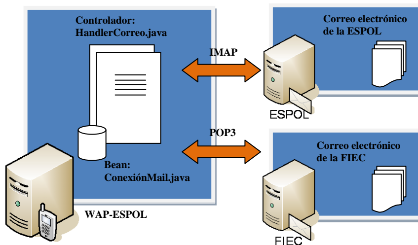
Figura 5.6.- Diagrama de flujo de información del correo ESPOL/FIEC
