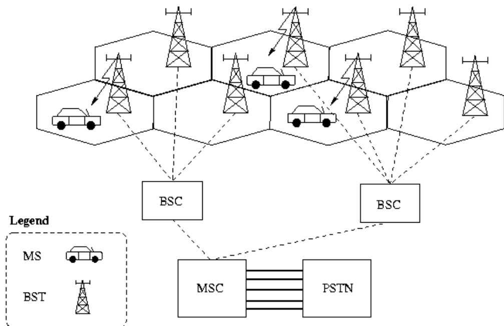
Figura 1.2.- Red de Telefonía celular
