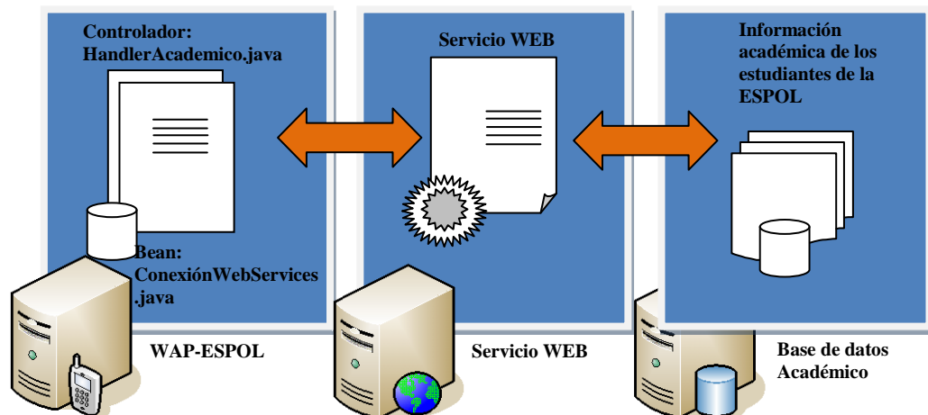
Figura 5.7. -Diagrama de flujo de información del Módulo Académico
