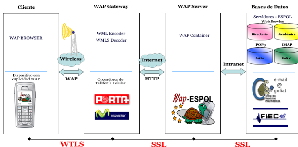
Figura 4.1-. Seguridad lógica a lo largo del canal de comunicación entre un dispositivo móvil y los repositorios de datos
