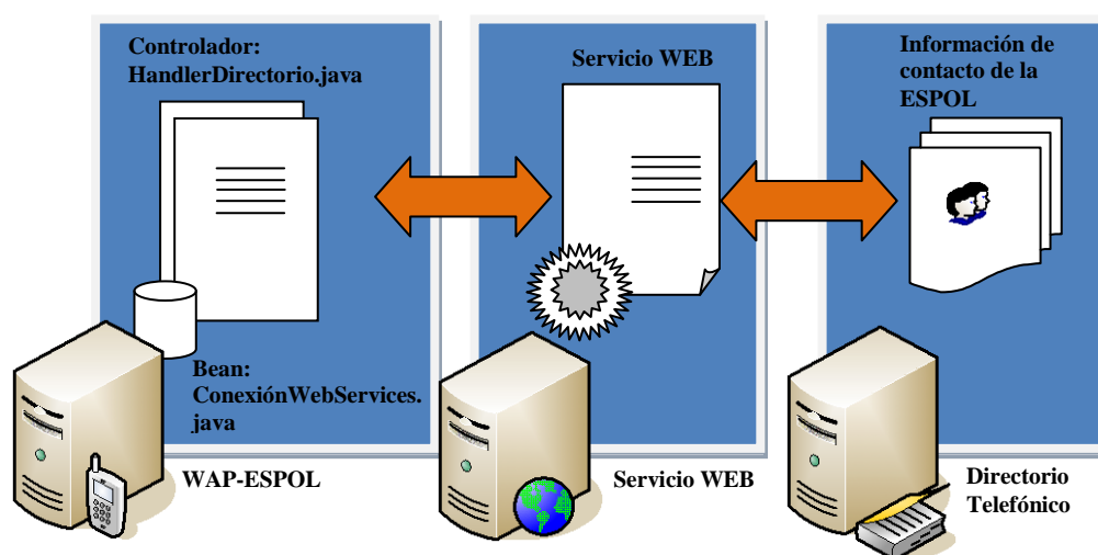
Figura 5.5.- Diagrama de flujo de información del Módulo Directorio. Acceso al Directorio Activo
