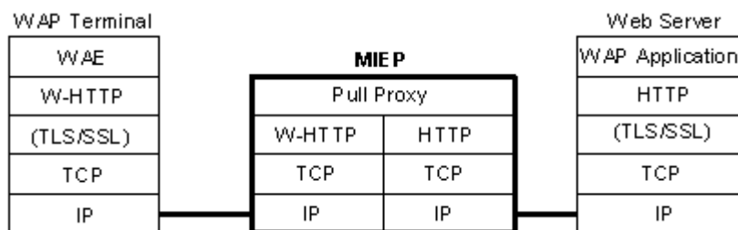
Figura 3.6.- Modelo del funcionamiento WAP2
