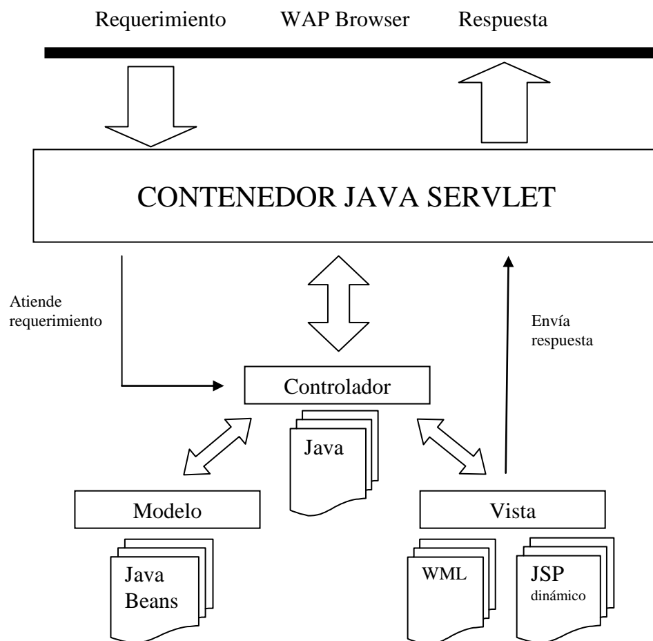
Figura 5.1.- Modelo MVC para el desarrollo WEB/WAP
