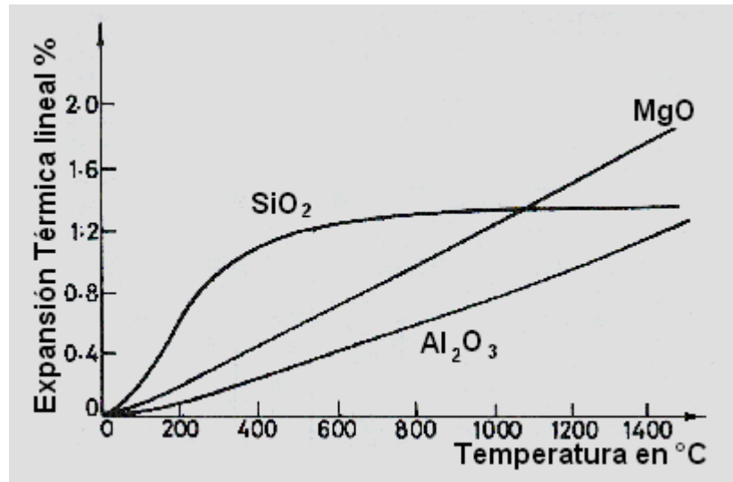
FIGURA 2.3 LÍNEA DE EXPANSIÓN TÉRMICA DE MATERIALES REFRACTARIOS APISONABLES.
