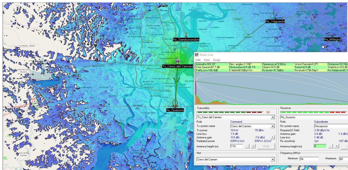
Figura 1.23: Intensidad de Campo Guasmo
