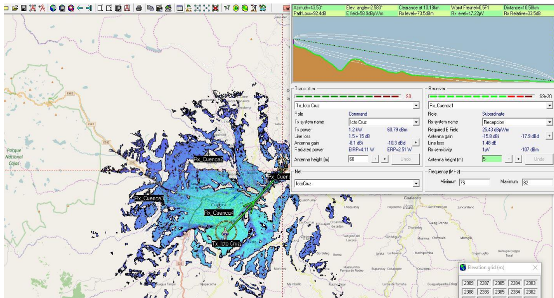
Figura 1.44: Intensidad de Campo Noroeste Cuenca
