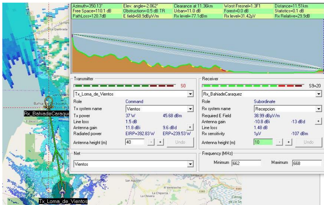
Figura 2.57: Intensidad de Campo Bahía de Caráquez
