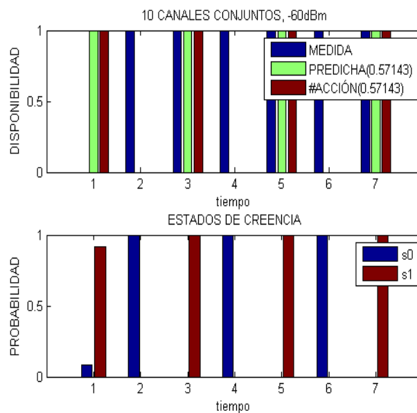
Figura 3.14: Predicción de la disponibilidad de un canal conjunto de 10 canales.
