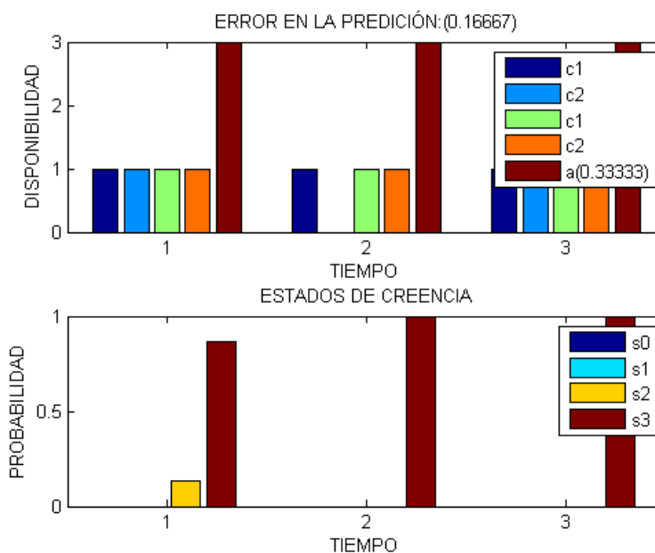
Figura 3.41: Predicción de la disponibilidad del canal 41(c1) al 42(c2) UHF.
