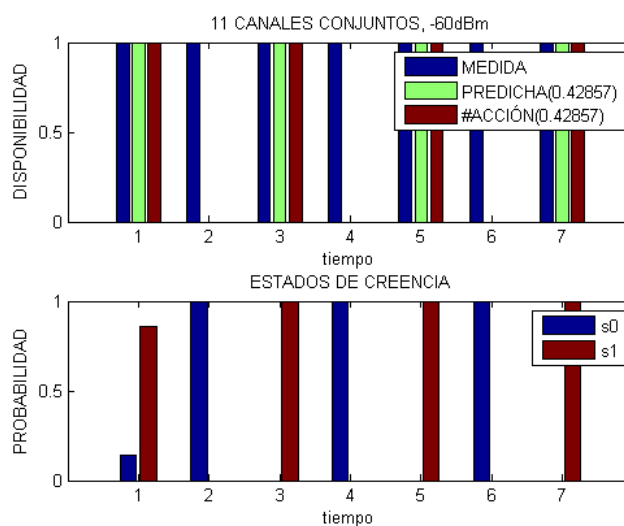
Figura 3.9: Predicción de la disponibilidad de un canal conjunto de 11 canales.
