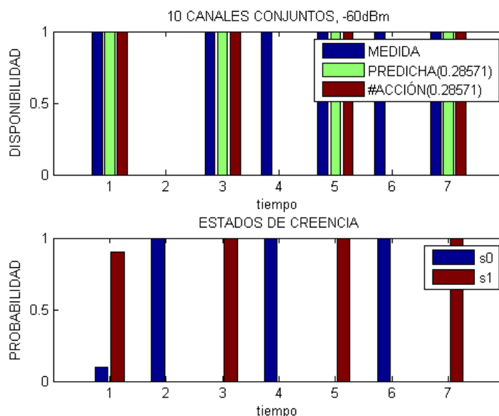
Figura 3.15: Predicción de la disponibilidad de un canal conjunto de 10 canales.
