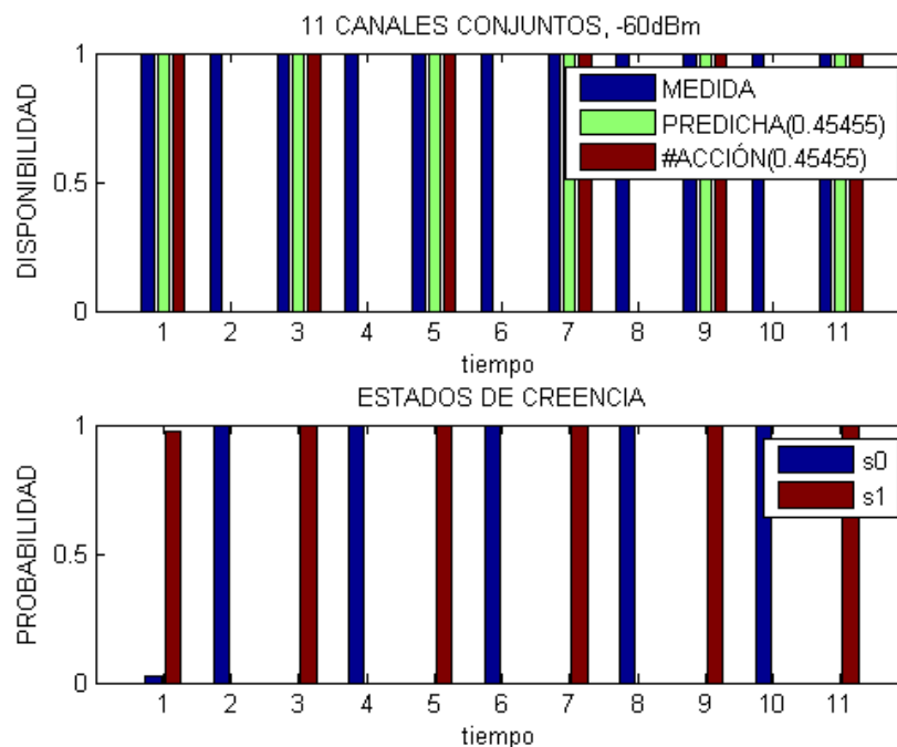
Figura 3.7: Predicción de la disponibilidad de un canal conjunto de 11 canales.
