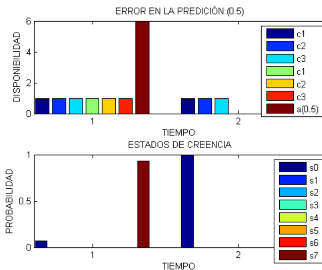
Figura 3.31: Predicción de la disponibilidad de un canal conjunto de 10(c1), 11(c2) y 12(c3) canales.
