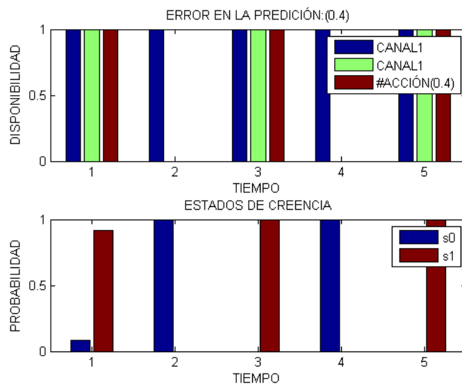
Figura 3.21: Predicción de la disponibilidad de un canal conjunto de 10 canales.
