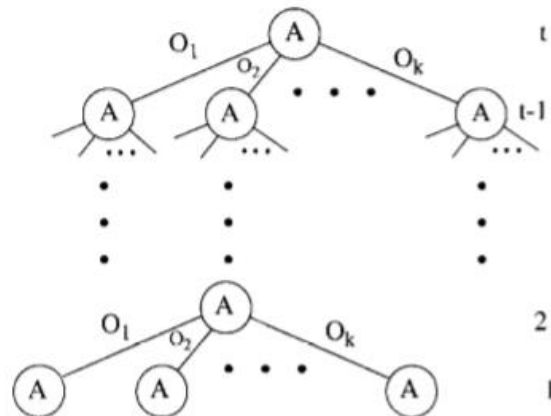
Figura 2.1: Un árbol de política de t pasos de tiempo.
