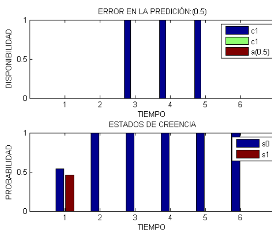
Figura 3.34: Predicción de la disponibilidad del canal 26 UHF
