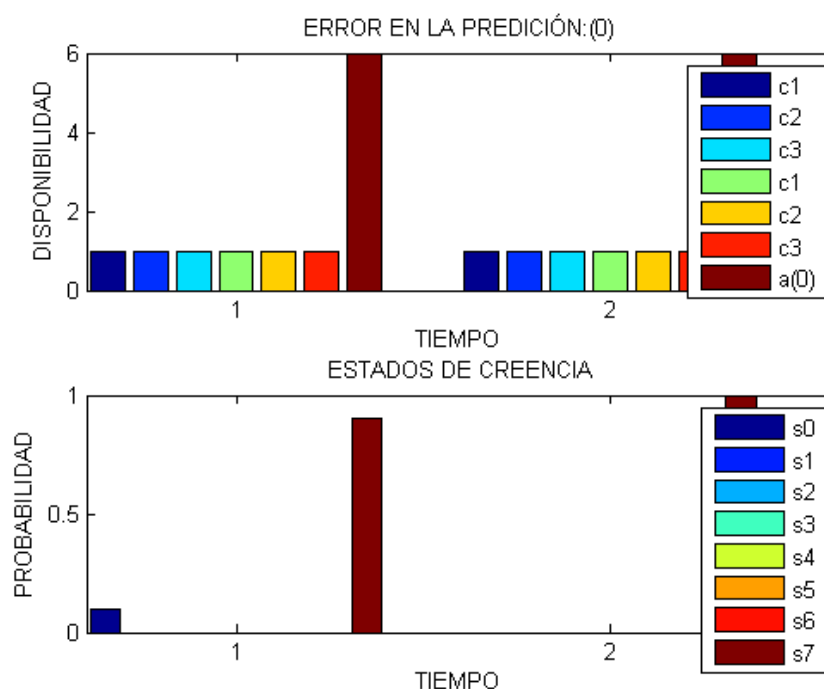
Figura 3.24: Predicción de la disponibilidad de un canal conjunto de 10(c1), 11(c2) y 12(c3) canales.
