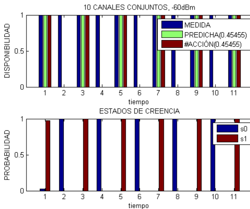
Figura 3.6: Predicción de la disponibilidad de un canal conjunto de 10 canales.
