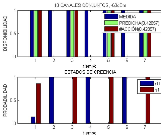
Figura 3.8: Predicción de la disponibilidad de un canal conjunto de 10 canales.
