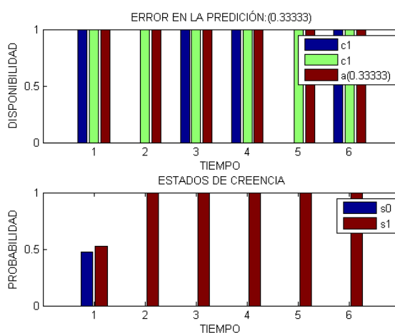
Figura 3.33 Predicción de la disponibilidad del canal 26 UHF.
