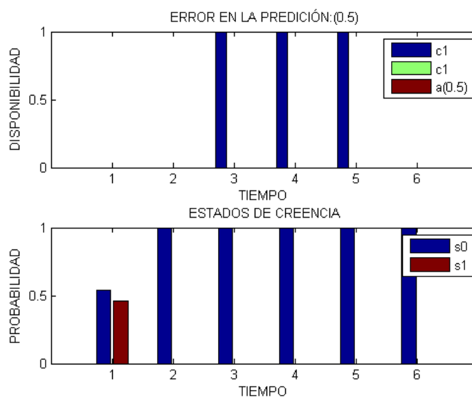
Figura 3.38: Predicción de la disponibilidad del canal 28 UHF.
