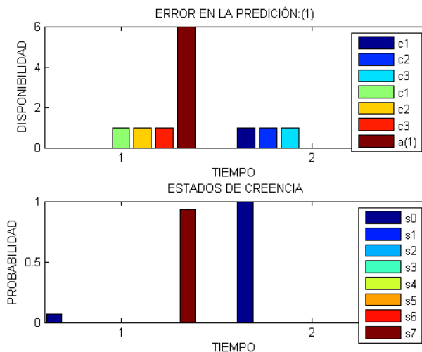
Figura 3.30: Predicción de la disponibilidad de un canal conjunto de 10(c1), 11(c2) y 12(c3) canales.
