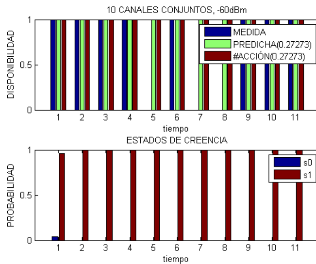
Figura 3.1: Predicción de la disponibilidad de un canal conjunto de 10 canales.
