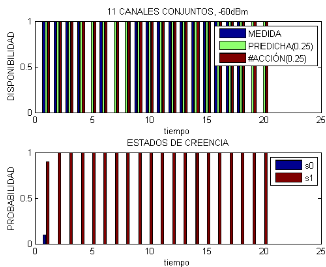
Figura 3.2 Predicción de la disponibilidad de un canal conjunto de 11 canales.
