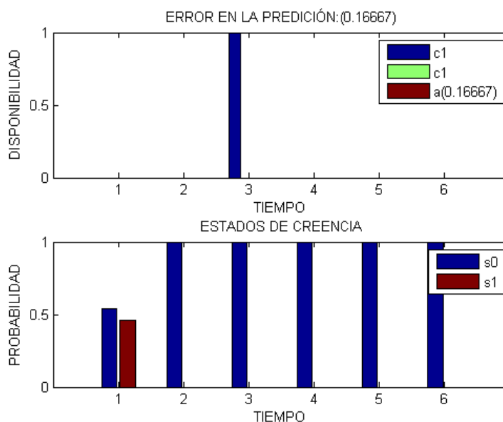
Figura 3.36: Predicción de la disponibilidad del canal 26 UHF.
