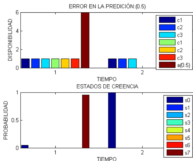
Figura 3.28: Predicción de la disponibilidad de un canal conjunto de 10(c1), 11(c2) y 12(c3) canales.
