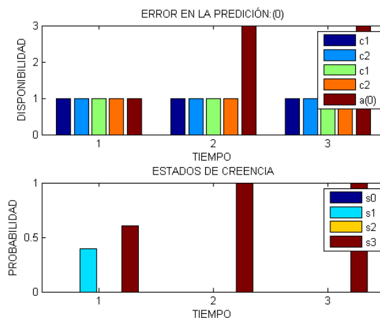
Figura 3.39. Predicción de la disponibilidad del canal 30 al 31 UHF.
