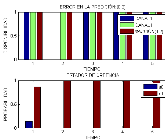
Figura 3.17: Predicción de la disponibilidad de un canal conjunto de 10 canales.
