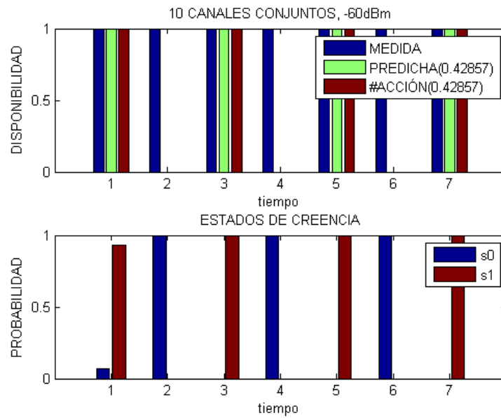
Figura 3.11: Predicción de la disponibilidad de un canal conjunto de 10 canales.
