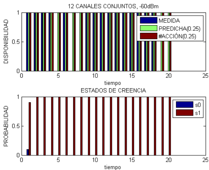
Figura 3.3: Predicción de la disponibilidad de un canal conjunto de 12 canales.
