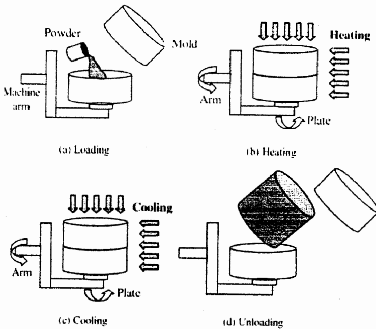
FIGURA 2.10 ESQUEMA DEL PROCESO DEL ROTOMOLDEO, SACADO DE ROTACIONAL MOLDING: A PRACTICAL GUIDE DE PAUL NUGENT
