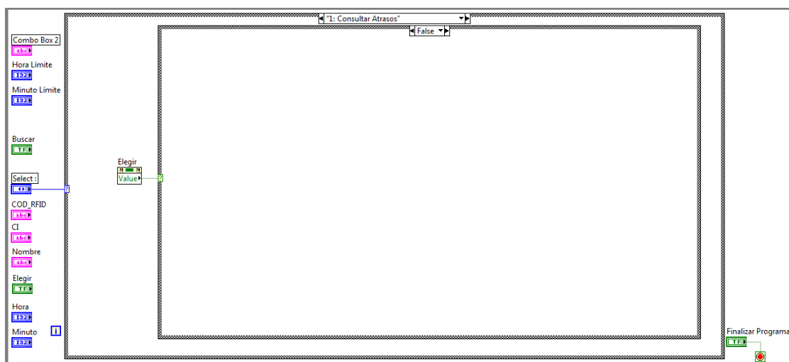
Figura 3.47 Diagrama de Bloques de Consulta Atrasos B
