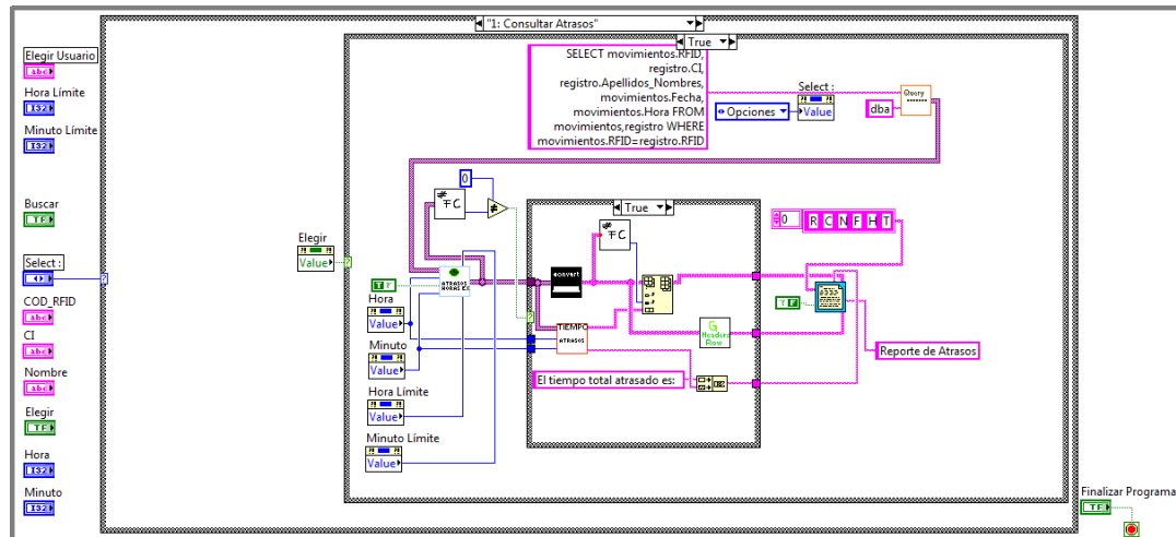
Figura 3.25 Diagrama de Bloques de Consulta Atrasos A
