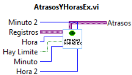
Figura 3.28 Query.vi
