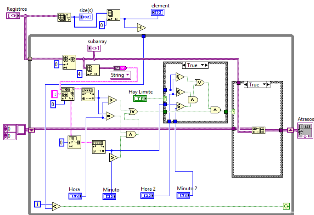
Figura 3.29 Diagrama de Bloques de AtrasosYHorasEx.vi A
