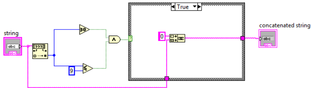
Figura 3.40 Diagrama de Bloques de FormatoMin.vi
