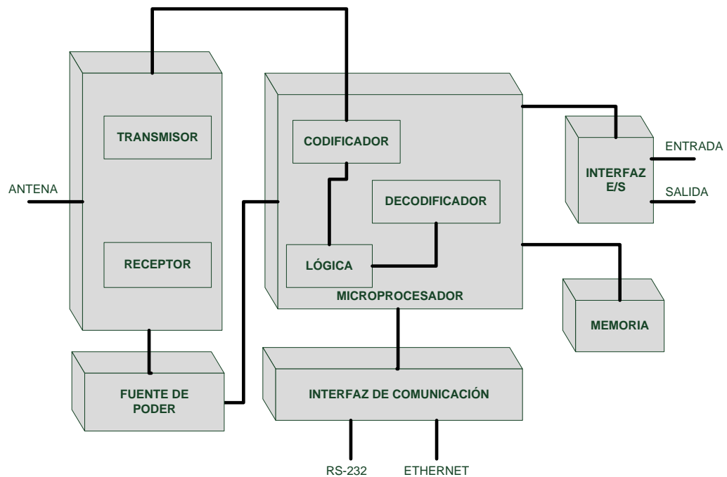
Figura 2.2 Componentes Lector RFID
