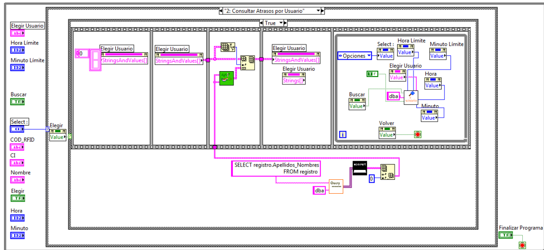
Figura 3.48 Diagrama de Bloques de Consulta Atrasos por Usuario A
