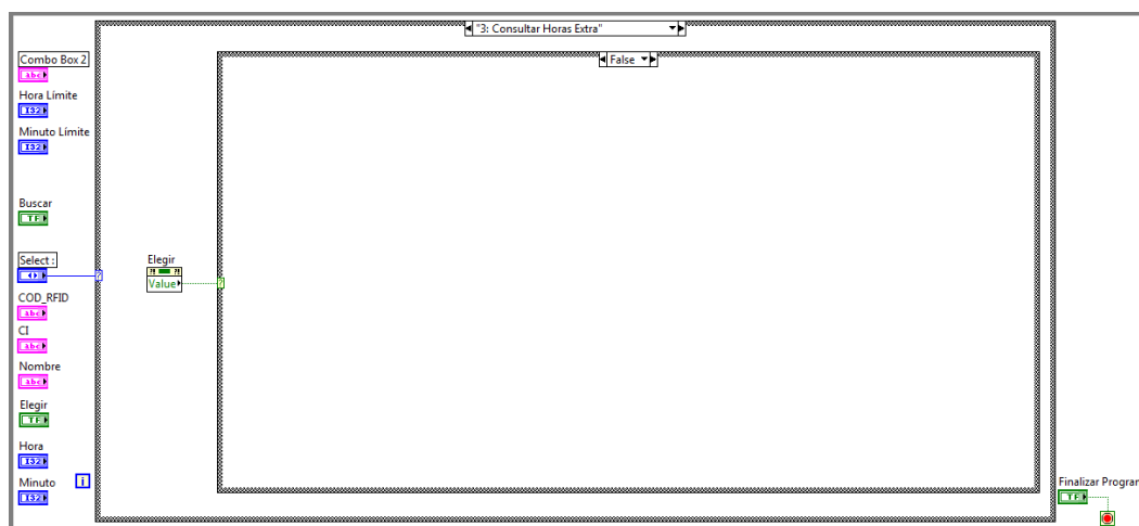
Figura 3.55 Diagrama de Bloques de Consulta Horas Extra B
