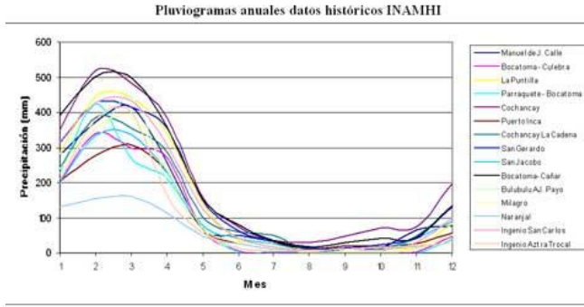
Figura 1.4 Pluviogramas anuales datos históricos INAHMI.
