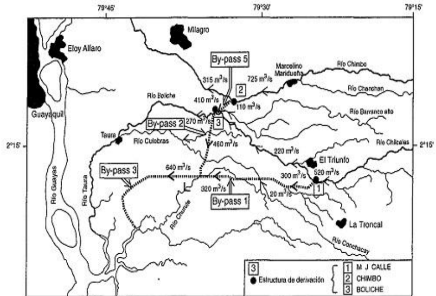
Figura 1.3 Descargas derivadas por los diferentes “bypass” (CEDEGE 1995).
