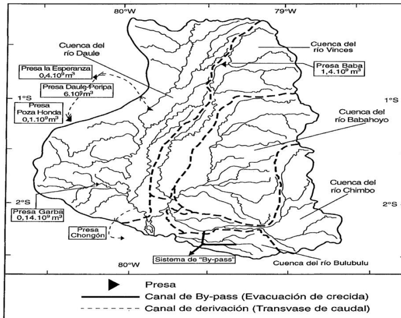
Figura 1.2 Ubicación de las principales obras de protección contra las inundaciones.
