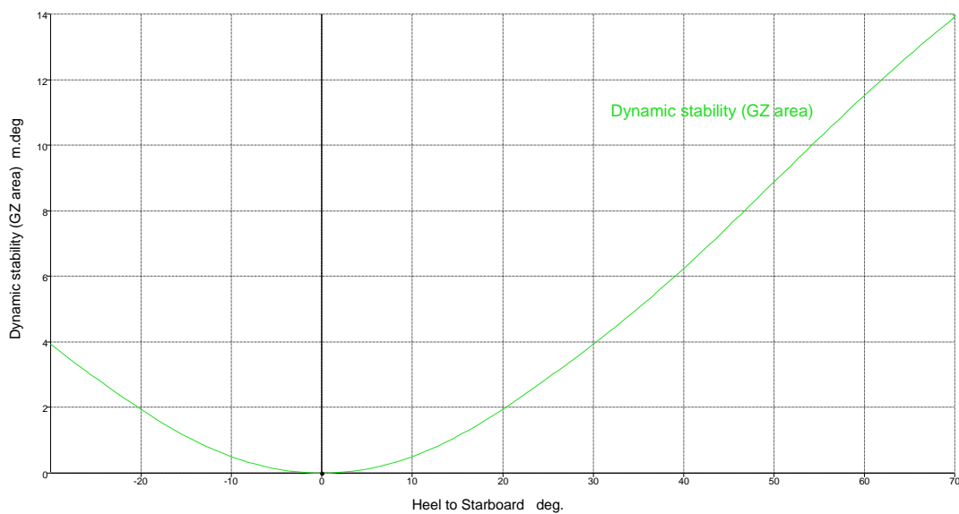
Figura No. 23 Curva de estabilidad dinámica a máxima carga, Atunero I. Fuente: Maxsurf Stability v.20- versión de prueba.
