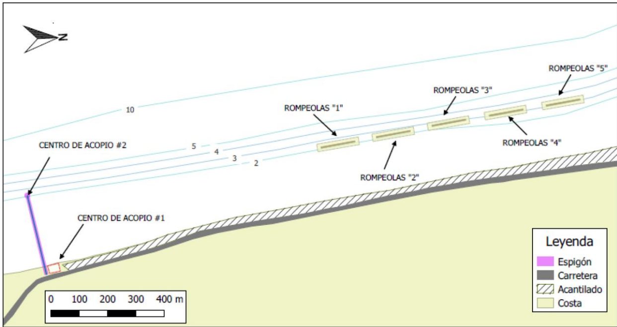
Figura 3.28 Propuesta de protección costera para el área de Playa Bruja propuesto por Cansing & Mena (2018)
