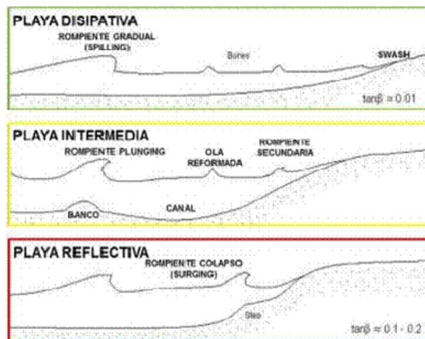
Figura 2.6 Caracterización morfodinámica de la playa.
