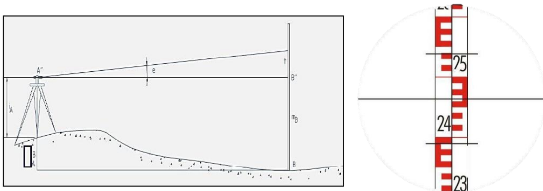
Figura 2.5 Esquema para realizar el perfil de la playa usando nivel y estadia.
