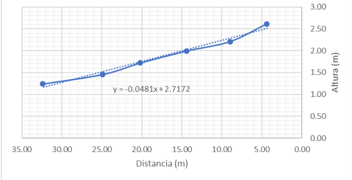
Perfil de Playa - Estación 5 - 15 de junio del 2019
