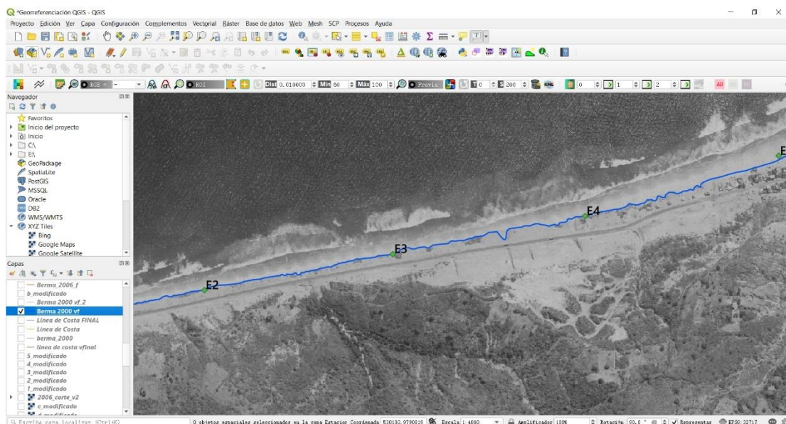
Figura 2.7 Imagen georreferenciada de la zona de estudio utilizando QGIS.
