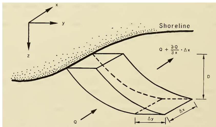
Figura 1.4 Esquema hipotético de un perfil de playa en equilibrio. (Larson, 1987)
