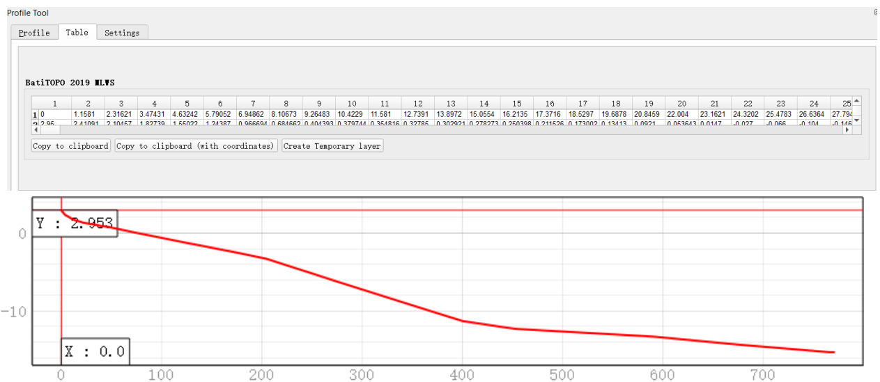
Figura 2.10 Perfil transversal de la playa con su respectiva tabla de valores.
