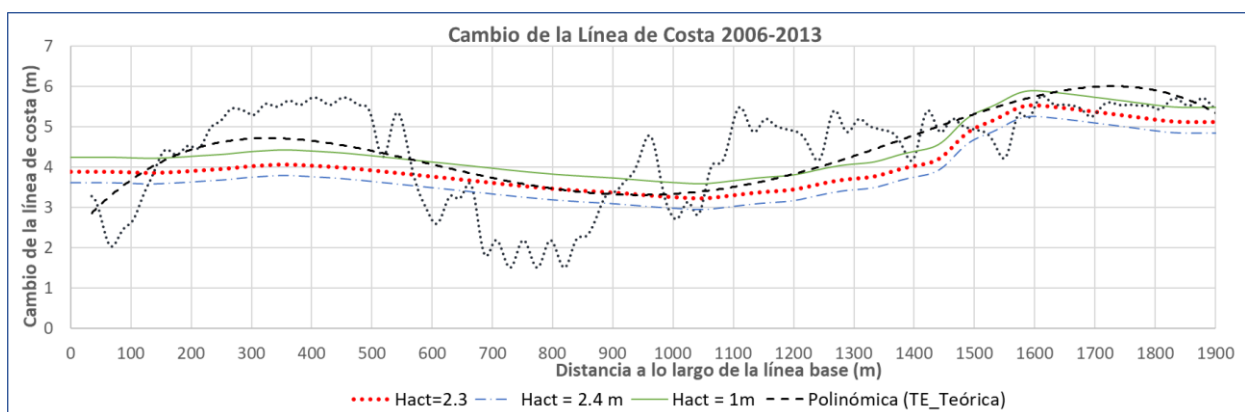
Figura 2.12 Calibración LITLINE para diferentes alturas activas (Autores, 2019)
