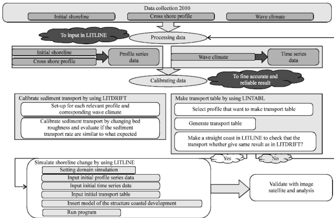
Figura 2.8 Esquema gráfico de la metodología de modelaje en LITLINE (Fadhi,2014)
