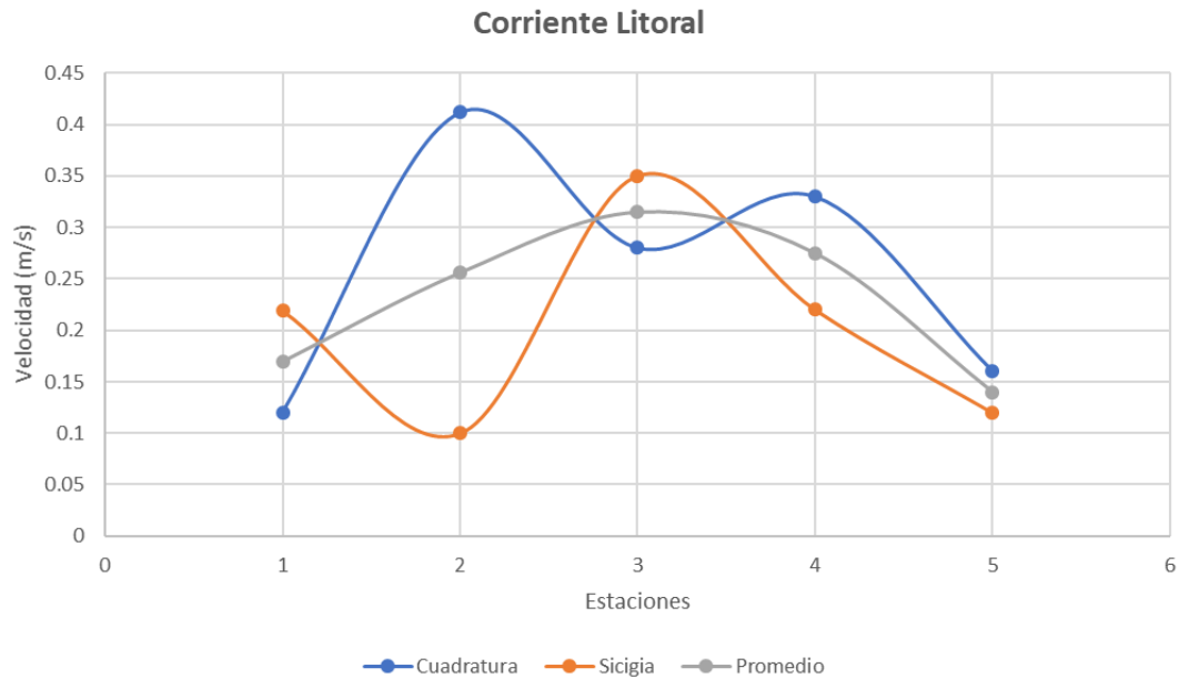
Figura 3.5 Velocidad litoral promedio por estación (Autores, 2019)
