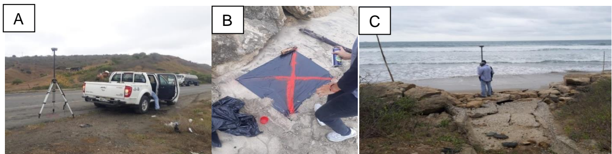
Figura 2.1 Instalación del equipo de topografía (Autores, 2019)
