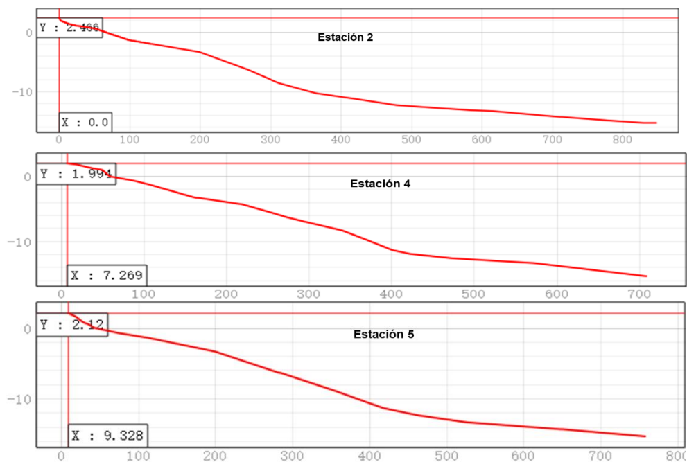
Figura 3.19 Perfiles transversales extraídos de QGIS (Autores, 2019)
