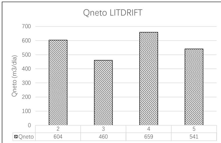
Figura 3.24 Transporte litoral promedio del período 2006-2013 para cada perfil (Autores, 2019)
