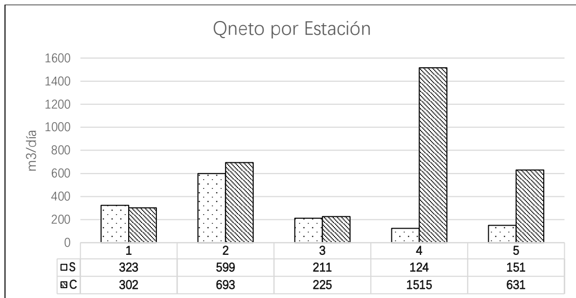
Figura 3.13 Transporte litoral promedio in situ para cada perfil en cuadratura y sicigia (Autores, 2019)
