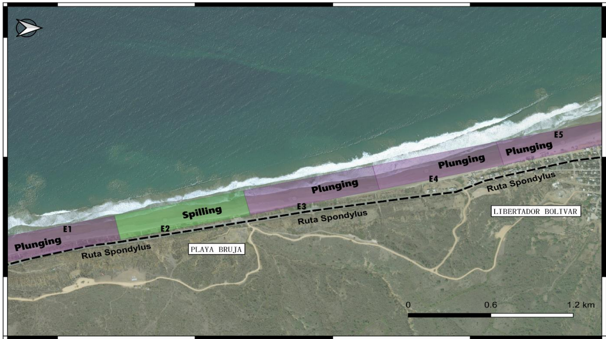
Figura 3.10 Tipo de ola rompiente de acuerdo al parámetro de Ibarren (Autores, 2019)
