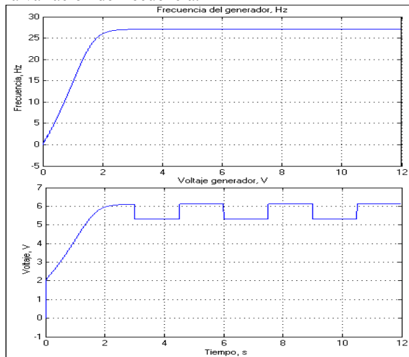
Figura 6. Respuesta del sistema frente a variaciones en la corriente de carga.
