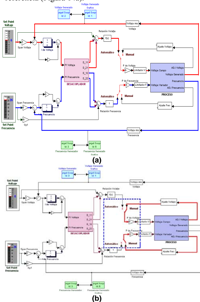
Figura 14. (a) Flujo de señales modo automático; (b) Flujo de señales modo manual.
