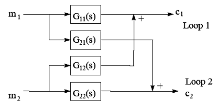
Figura 9. Estructura de un modelo multivariable 2x2.
