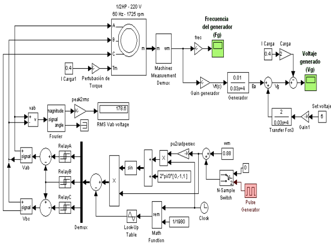
Figura 3. Diagrama del sistema real usando bloques de Simulink.
