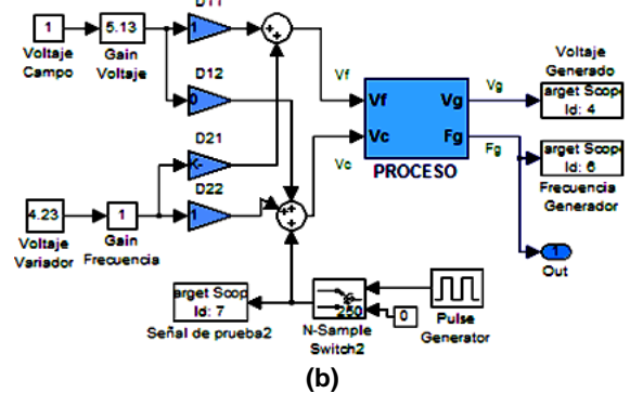
Figura 8. (a) Diagrama de bloques para un sistema 2x2 con bloque desacoplador; (b) Sistema real con bloque desacoplador.
