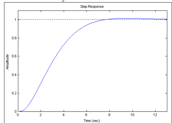
Figura 12. Respuesta al escalón del sistema Fg/Vc con el controlador PI.
