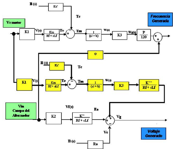
Figura 2. Sistema a controlar con relación entre variables.
