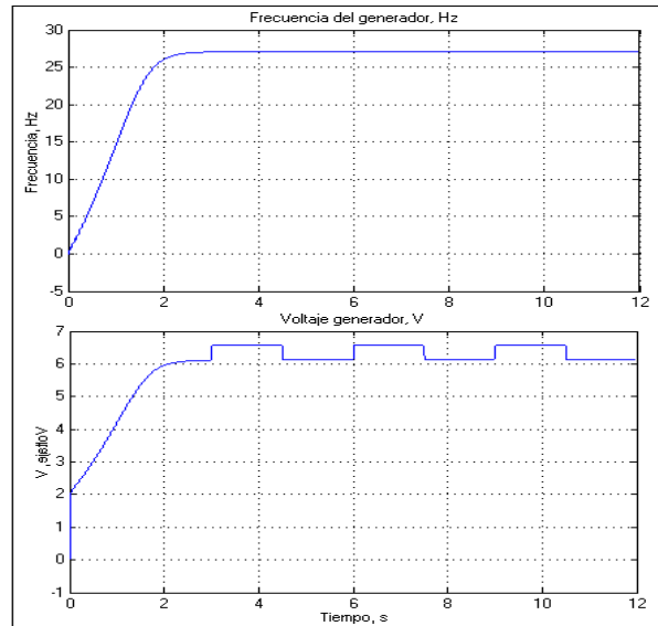
Figura 5. Respuesta del sistema frente a variaciones de V_f (voltaje de campo del alternador).
