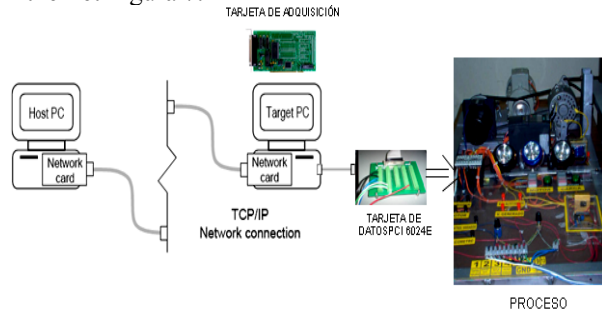
Figura 7. Sistema de adquisición de datos.
