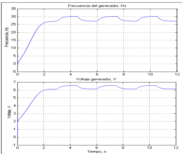
Figura 4. Respuesta del sistema frente a variaciones de V_c (voltaje de control del variador de frecuencia).
