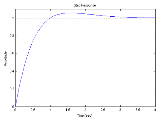
Figura 13. Respuesta al sistema V_g/V_f al escalón con el controlador PI.
