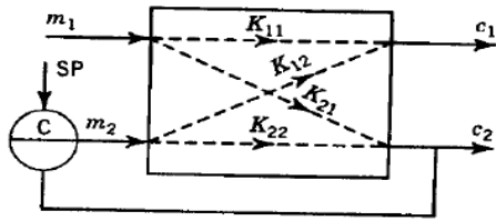
Figura 10. Estructura de un modelo multivariable manteniendo constante c_2 por medio de un lazo de control.
