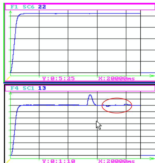
Figura 15. Señales frente a variación de carga a 16W. Superior: Frecuencia del generador; inferior: Voltaje del generador
