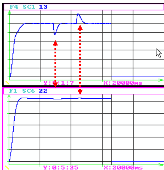
Figura 16. Señales frente a variación de carga a 33W. Superior: Voltaje del generador; inferior: Frecuencia del generador.
