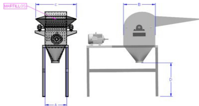
Gráfico 1.1 Proceso de la Molienda
