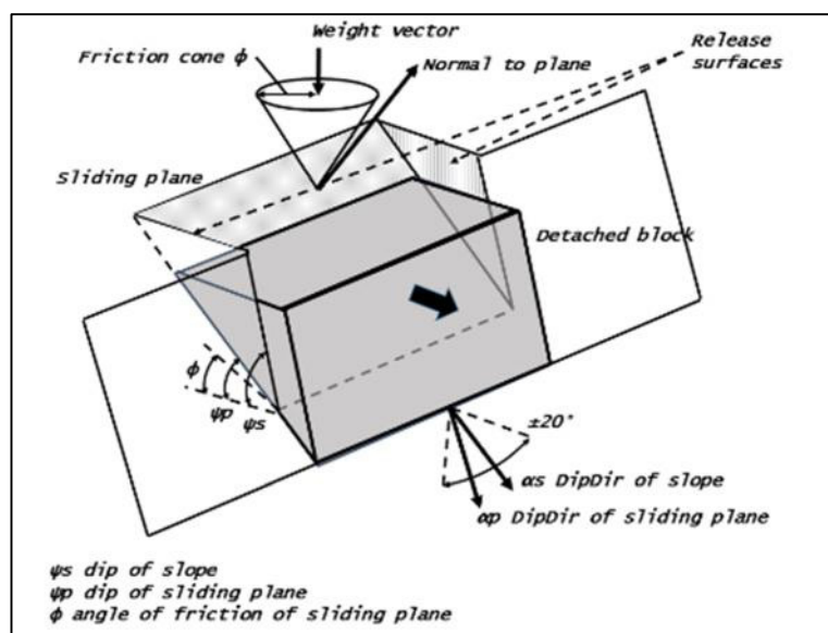
Figura 24 Esquema de un potencial deslizamiento plano, con las geometrías y elementos que intervienen.
