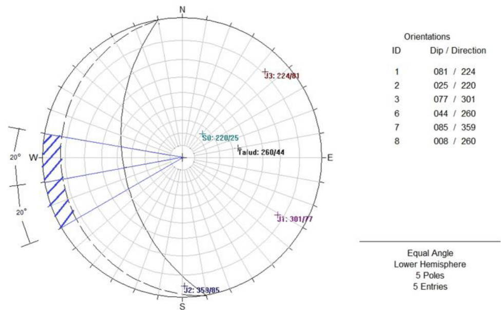
Figura 66 Análisis de susceptibilidad. Vuelco o toppling. Talud general
