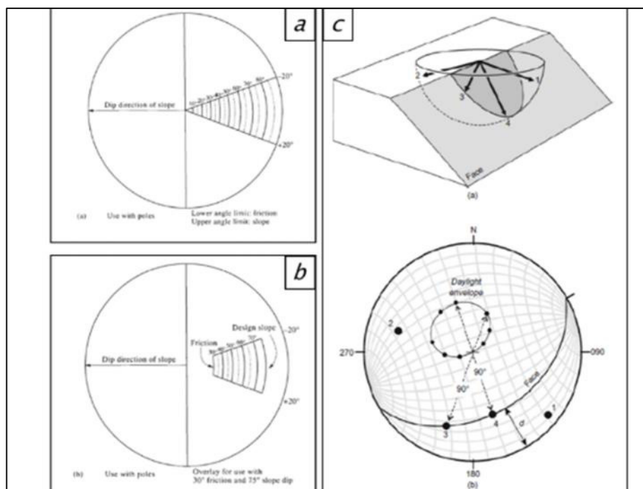
Figura 23 Criterios geométricos simples requeridos para una inestabilidad plana.
