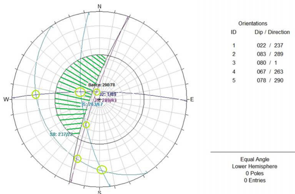
Figura 64 Análisis de susceptibilidad. Cuña. Banco. EGM 4
