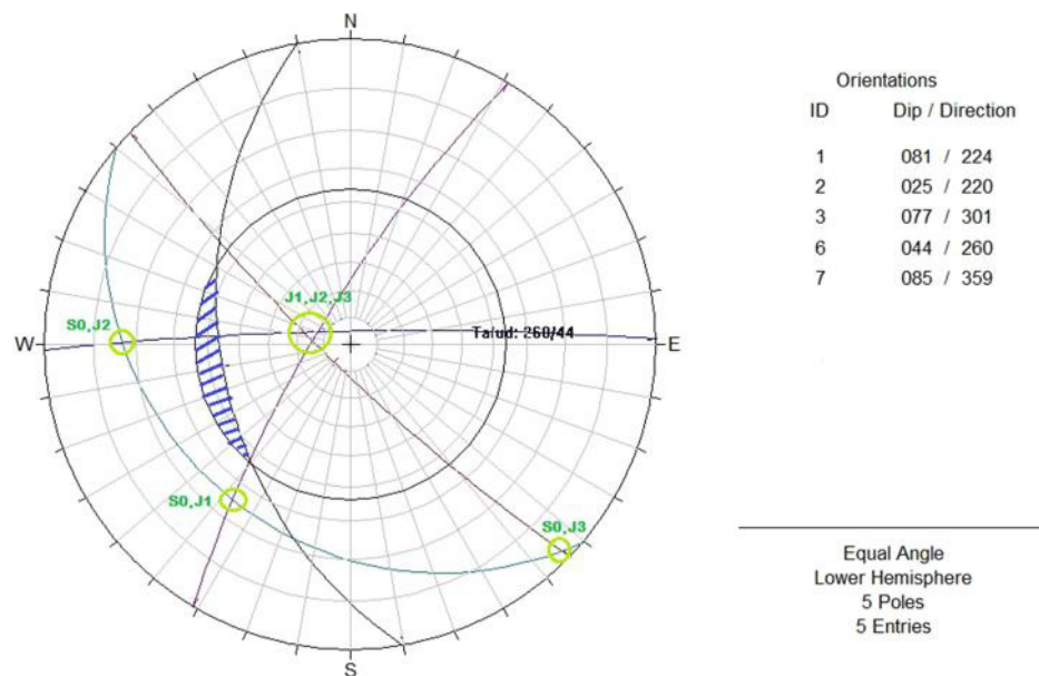
Figura 62 Análisis de susceptibilidad. Cuña. Talud
