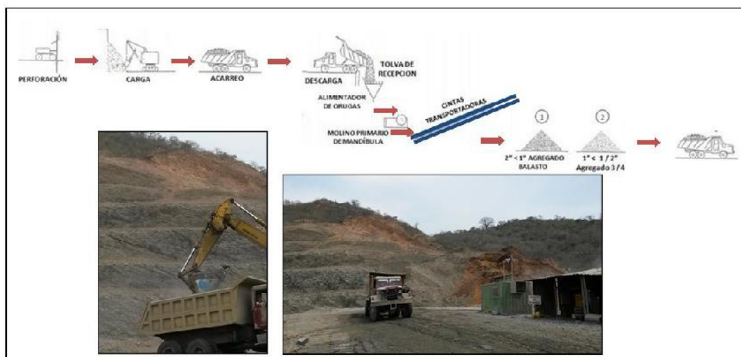
Figura 4 Proceso de explotación minera de la cantera BORCONS
