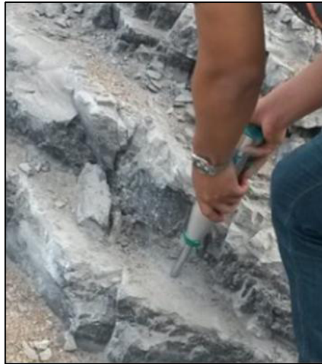
Figura 36 Detalle del esclerómetro o martillo Schmidt (tipo N). Medidas esclerométricas en la superficie de una discontinuidad.
