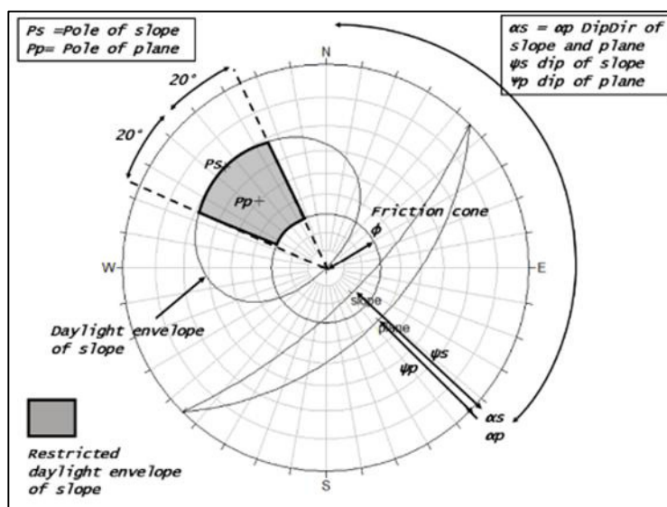
Figura 25 Esquema de las condiciones para deslizamiento plano en proyección estereográfica (igual ángulo).
