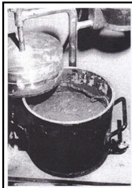
Ilustración 9.4 Aparato Vebe-Coherencia de la Prueba con el Anillo de Mortero en la Muestra Consolidada, Tomado de ACI 2011-207.5R.
