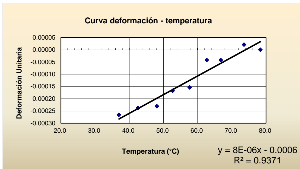
Ilustración 5. 15 Curva Deformación vs Temperatura Espécimen 1.
