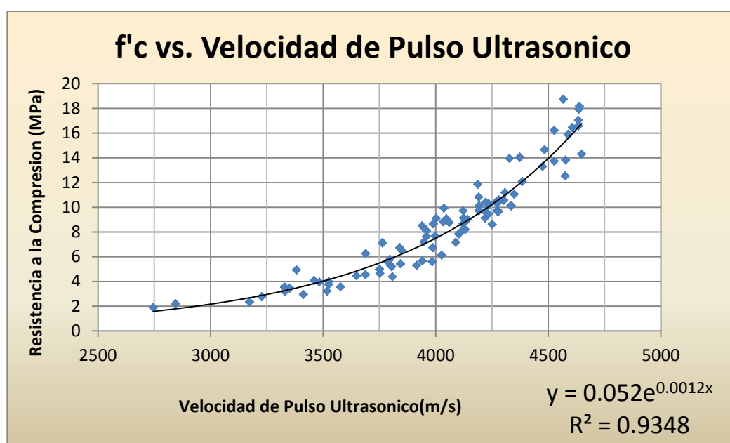
Ilustración 6. 20 Gráfica f'c vs Velocidad Pulso Ultrasonico.
