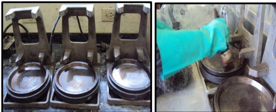
Ilustración 5. 2 Engrasado de Moldes para Refrentar.
