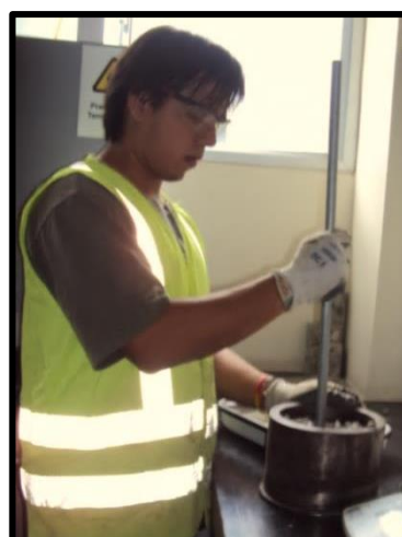
Ilustración 3. 10 Ensayo Valor de Trituración.
