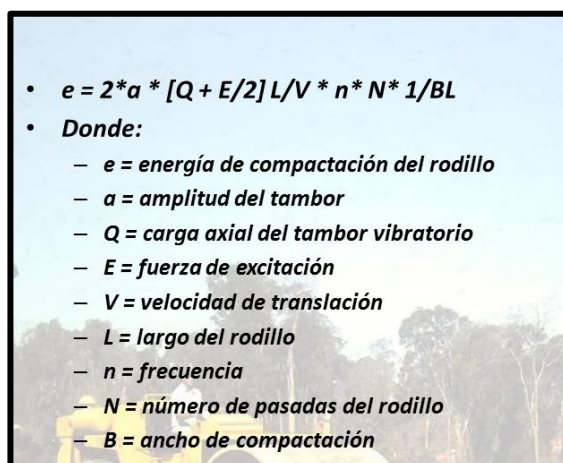
Ilustración 8. 23 Energía de Compactación, Tomado de la Presentación: HCR Evolución y Nuevos Horizontes - Ing. Miguel A. Golik.
