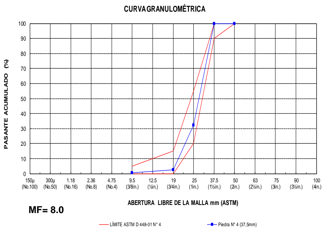
Ilustración 3. 8 Curva Granulométrica Piedra 38mm, ASTM C33M-11.
