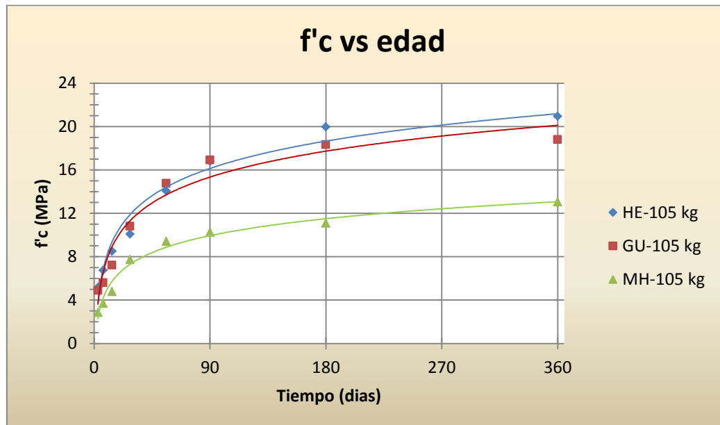
Ilustración 6. 3 Variación f'c vs Edad, 105 kg de Cemento (TMA 38mm).
