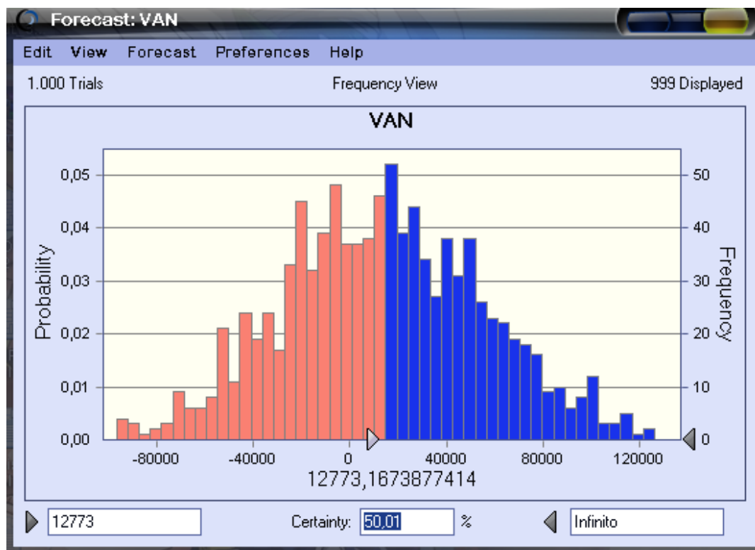
Gráfico 3.3.1 Análisis de Probabilidad del VAN
