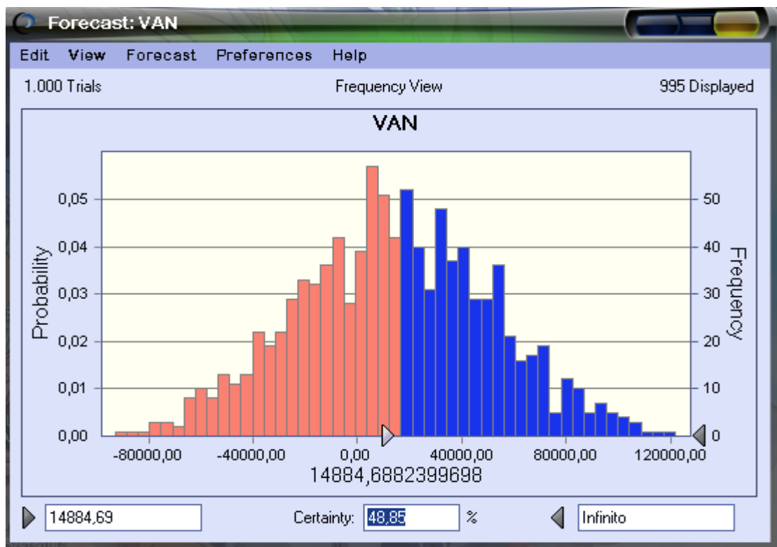
Gráfico 3.4.1 Análisis de Probabilidad del VAN Actual
