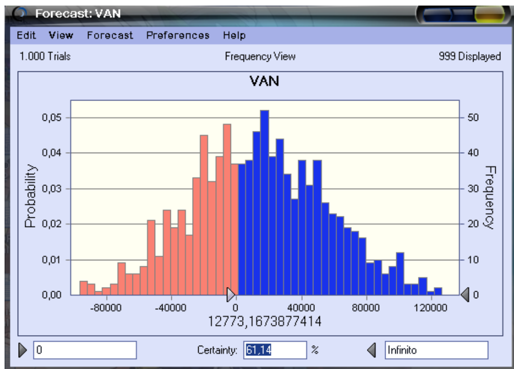
Gráfico 3.2 Análisis del VAN con el Proyecto
