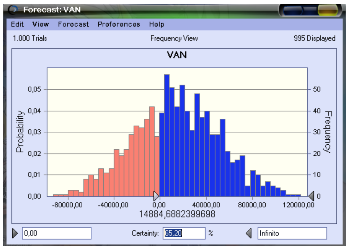
Gráfico 3.4 Análisis del VAN en la Situación Actual
