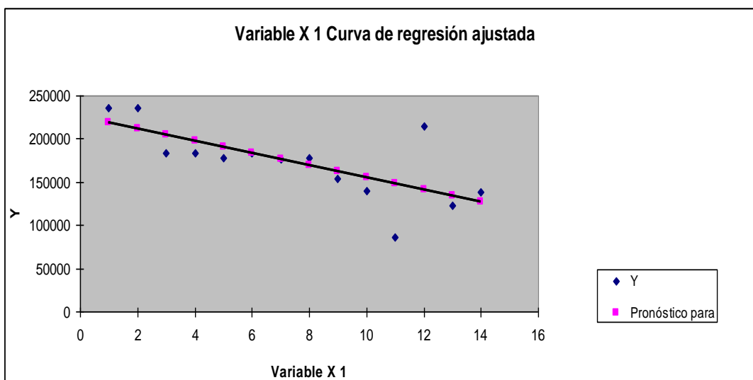
Gráfico 3.1 Regresión sobre ventas
