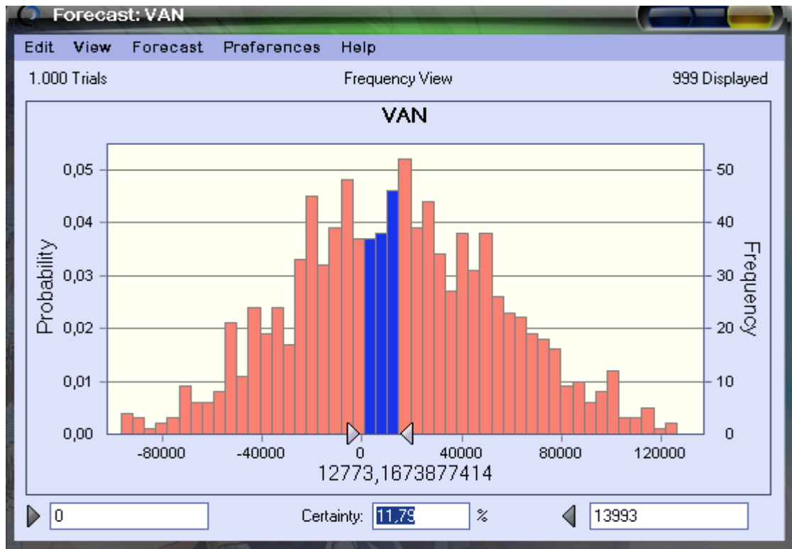
Gráfico 3.3.2 Análisis de Probabilidad del VAN
