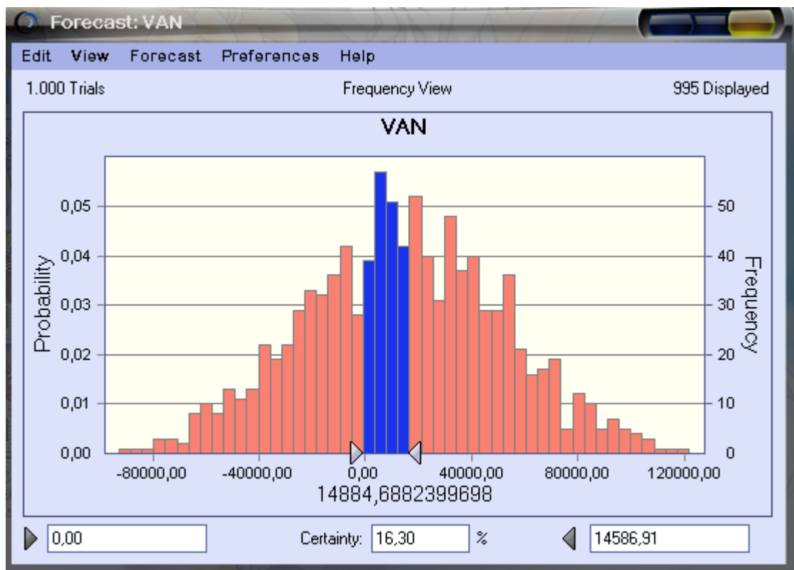
Gráfico 3.4.2 Análisis de Probabilidad del VAN Actual
