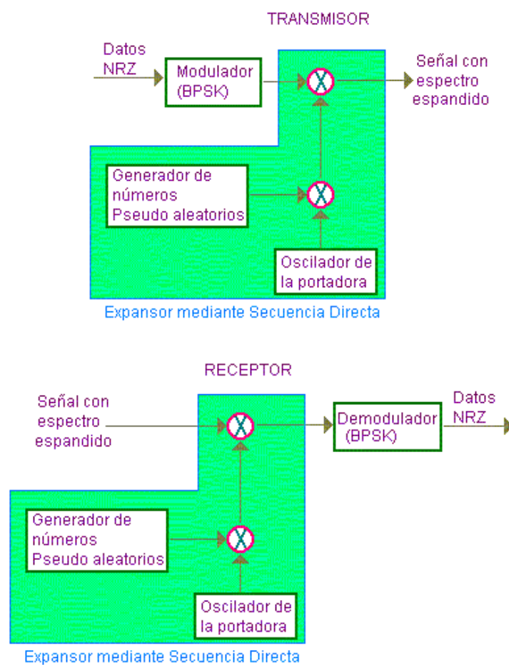
FIGURA 1. 16 Sistema de E.E. mediante Secuencia Directa
