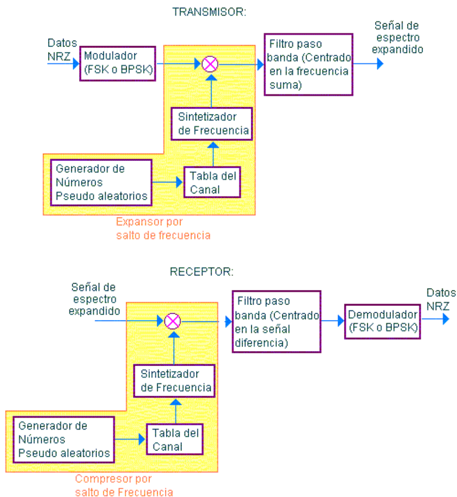
FIGURA 1. 13 Sistema de E.E. mediante salto de Frecuencia
