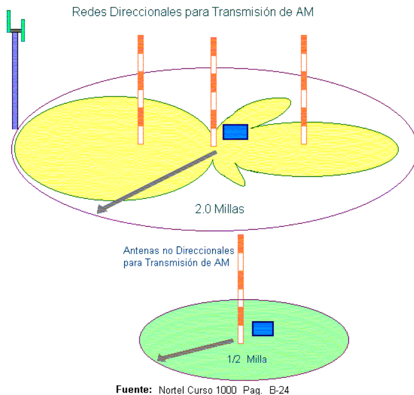
FIGURA 4.7 Transmisión de antenas AM
