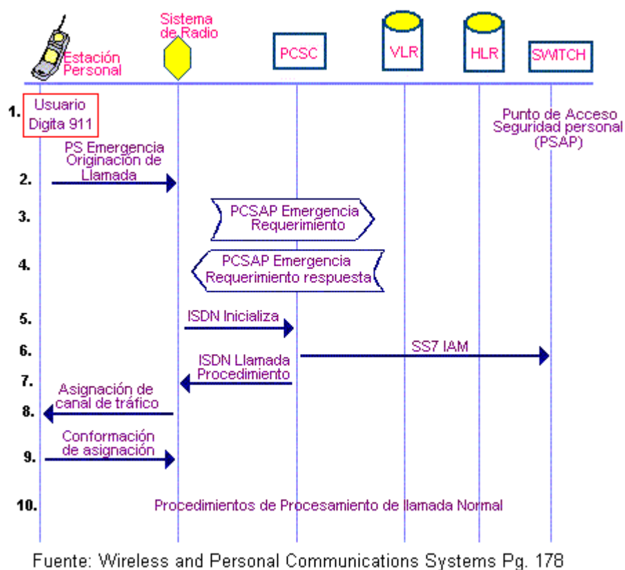
FIGURA 1. 23 Llamada de Emergencia de PS
