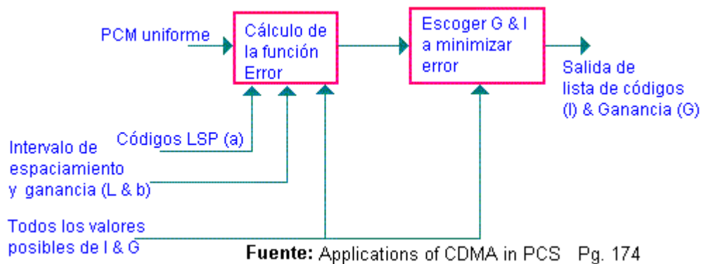
FIGURA 5.6 Codificador CELP para parámetros de densidad
