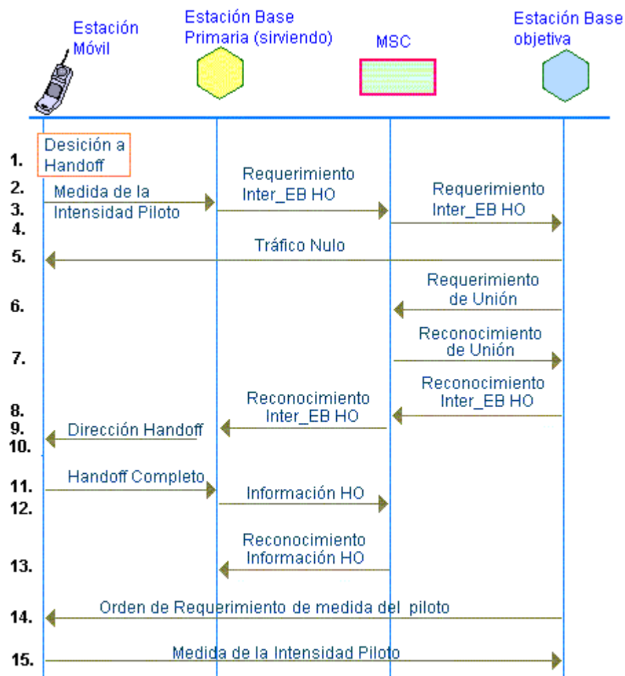
FIGURA 1. 30 Principio de Handoff suave CDMA
