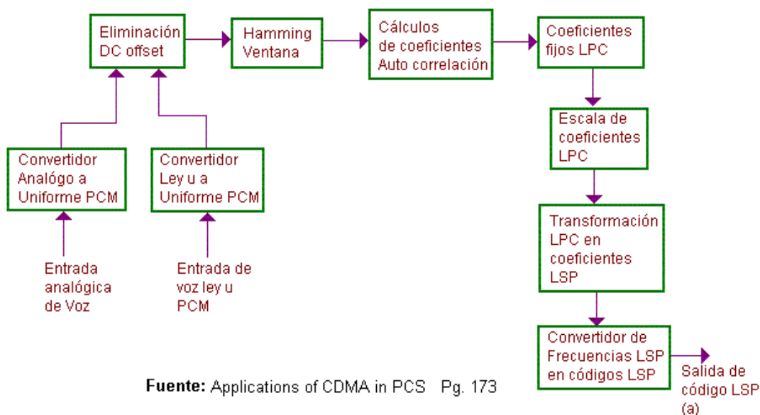
FIGURA 5.5 Codificador CELP para códigos LSP
