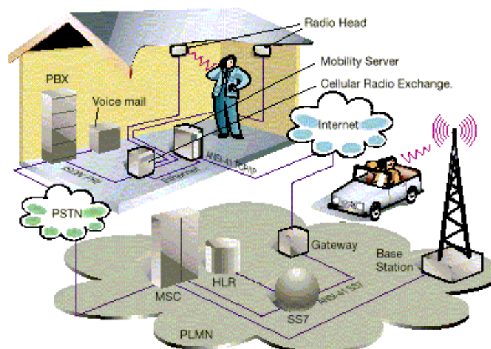
FIGURA 1. 1 Red de Telecomunicaciones
