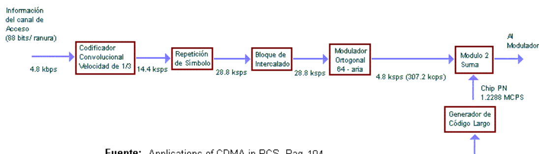
FIGURA 5.18 Canal de Acceso de Reversa CDMA
