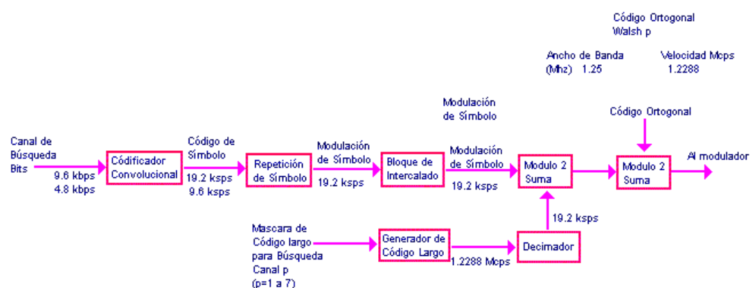
FIGURA 5.13 Bloques del Canal de Búsqueda CDMA delantero
