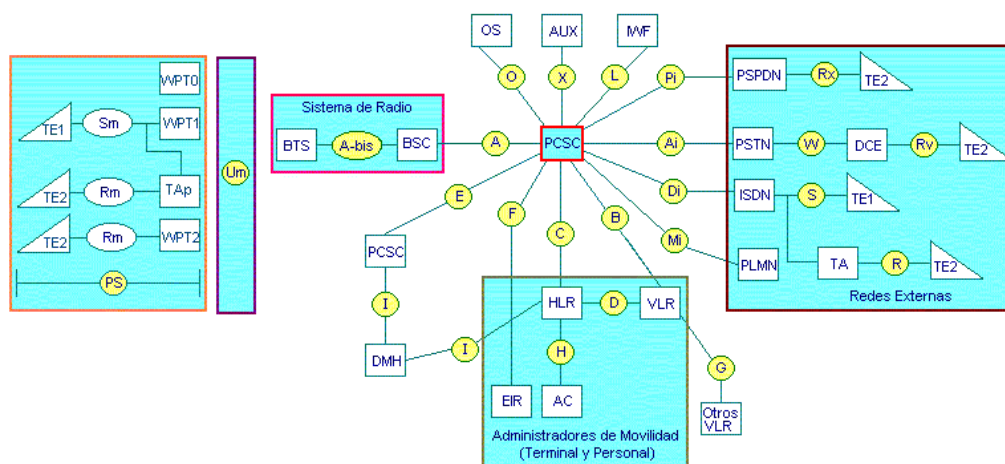
FIGURA 2. 7 Modelo de Referencia TR 45/46
