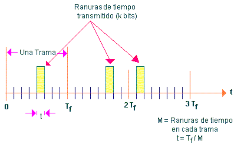
FIGURA 1. 17 Aproximación de E.E. por Salto de Tiempo
