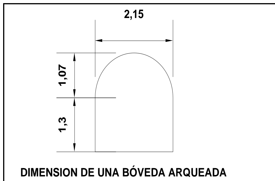
Fig. 3. Dimensiones de la Bóveda ( Crespo J. 2007)
