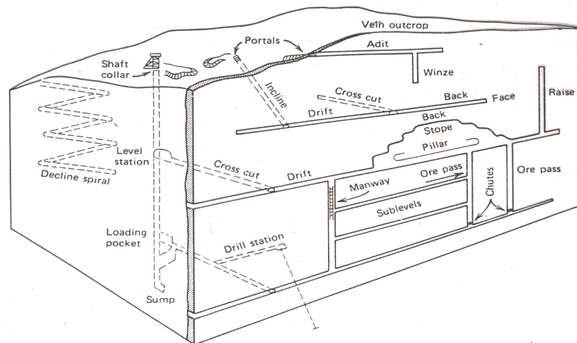
Fig. 9 Distintos elementos constitutivos de una mina subterránea.
