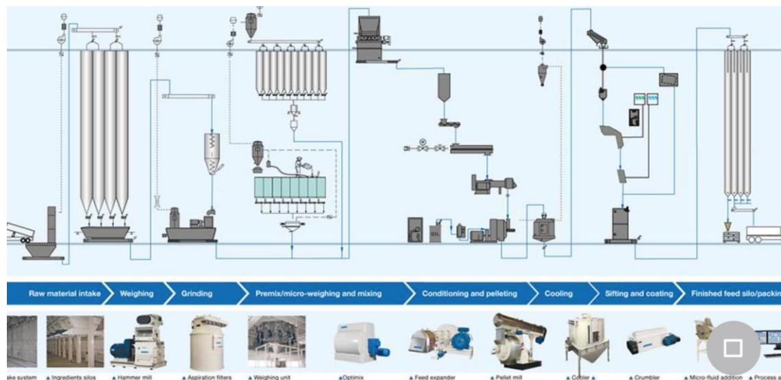
Ilustración 16, Flujo de proceso para el procesamiento de alimentos para mascotas
