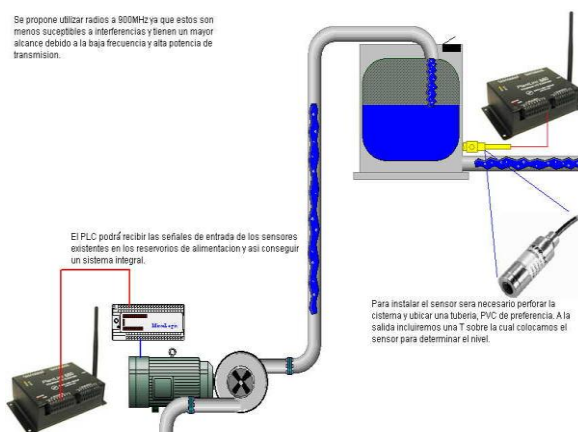
Figura 6. Estación reguladora de presión
