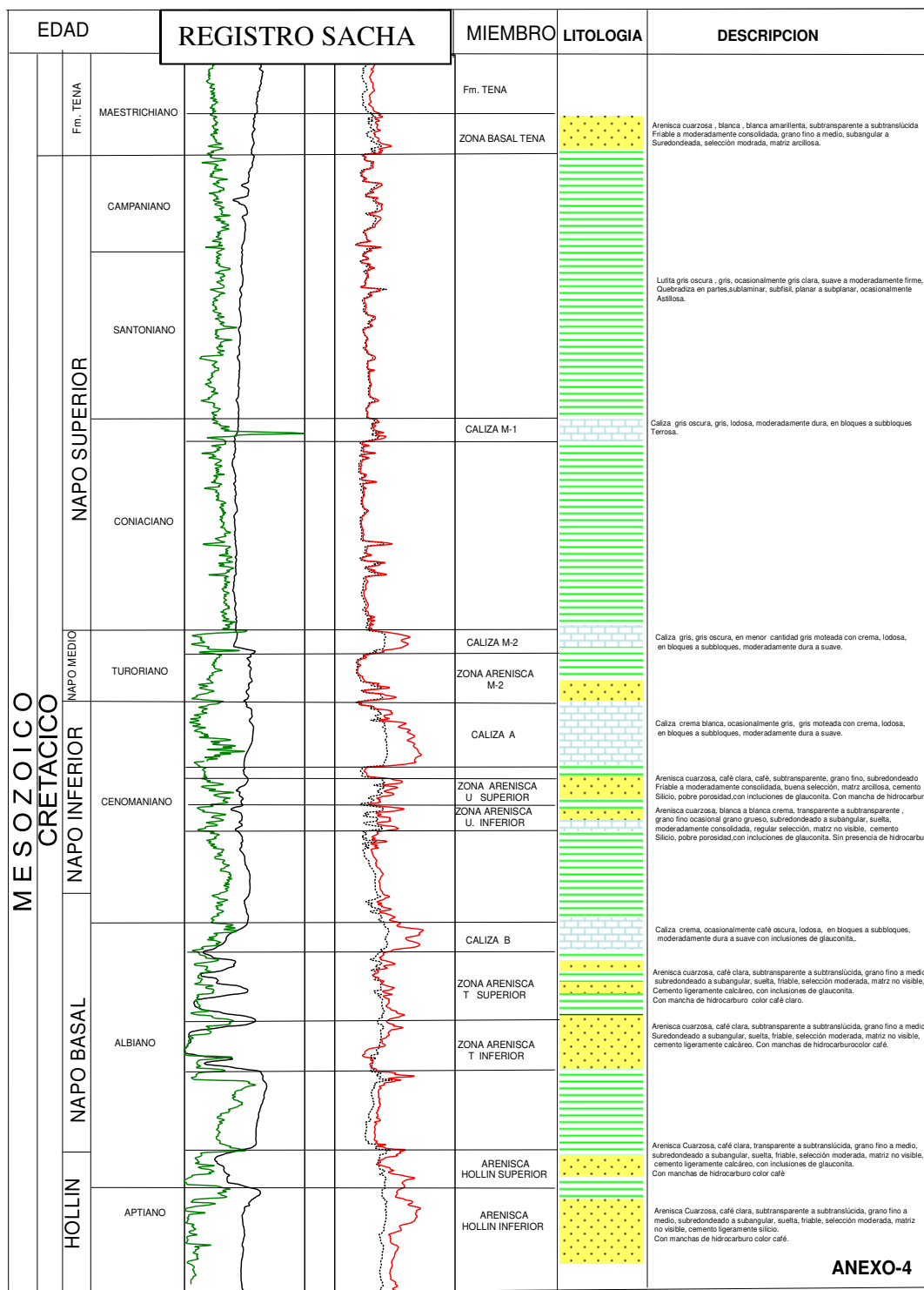
COLUMNA ESTRATIGRAFICA
