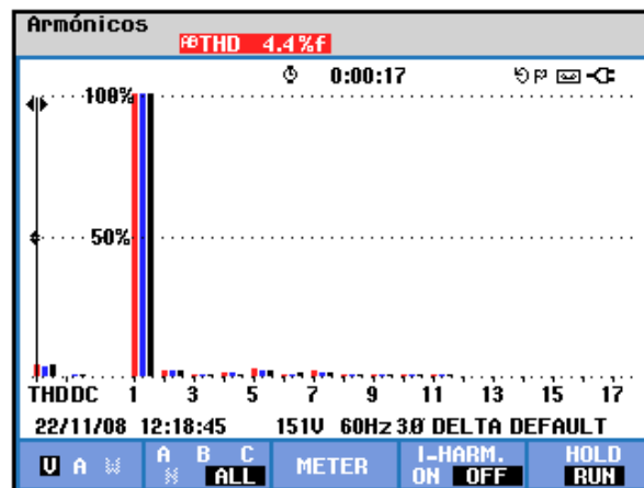
Figura 18 THD del voltaje durante la compensación del voltaje sag
