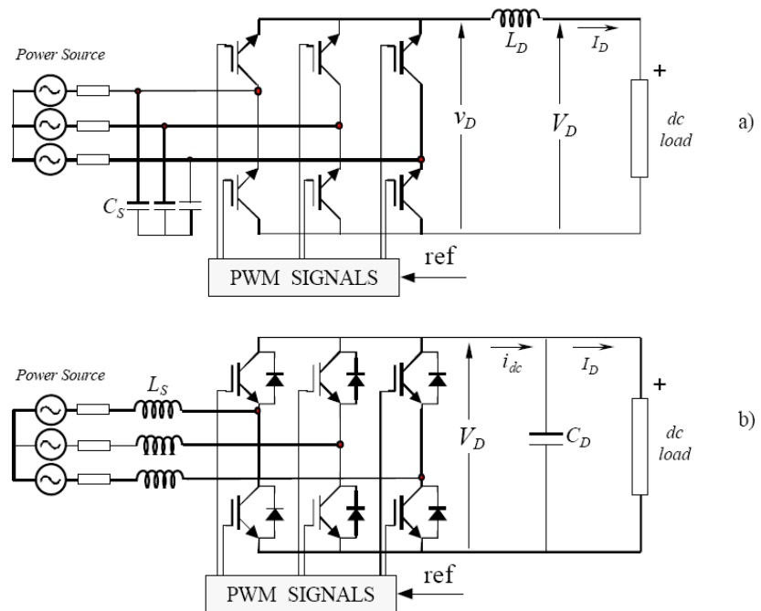
Figura 3.10 Topologías básicas de rectificadores PWM trifásicos conmutadas por fuerza: (a) rectificador fuente de corriente (CSR); (b) rectificador fuente de voltaje (VSR) (Fuente: Rashid).
