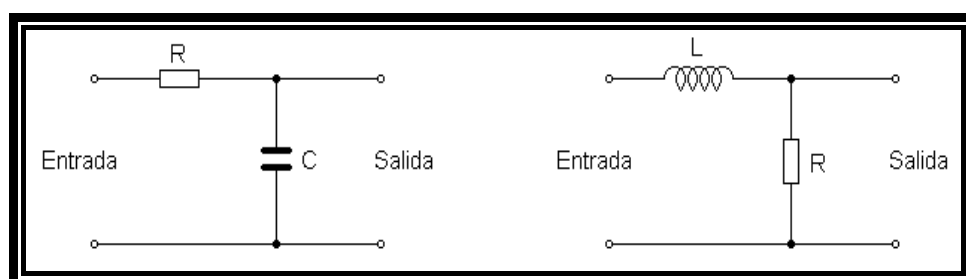
Figura 1.11 Filtros Pasivos.
