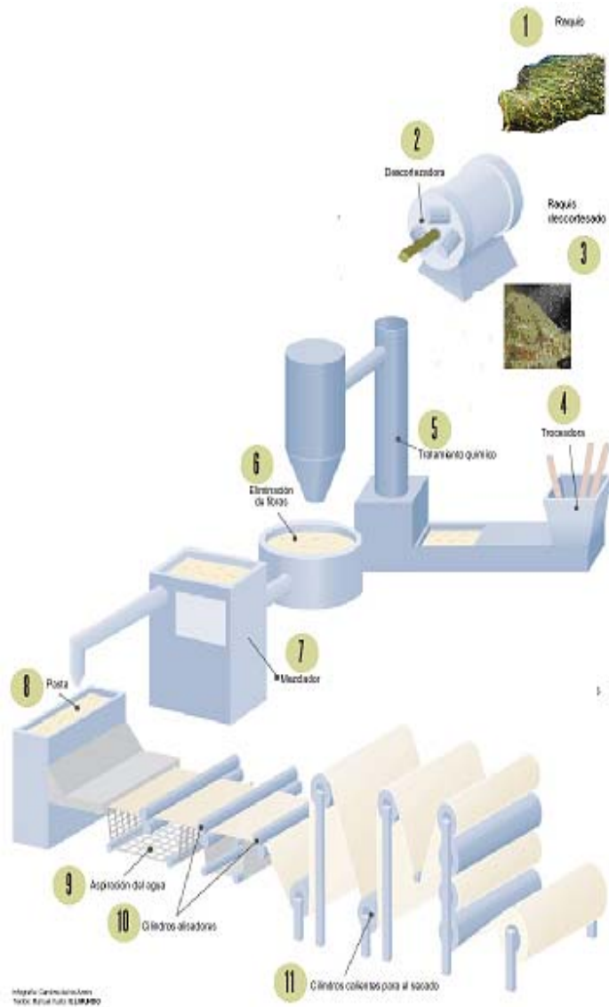
Figura 5.1 Proceso de elaboración de papel de banano
