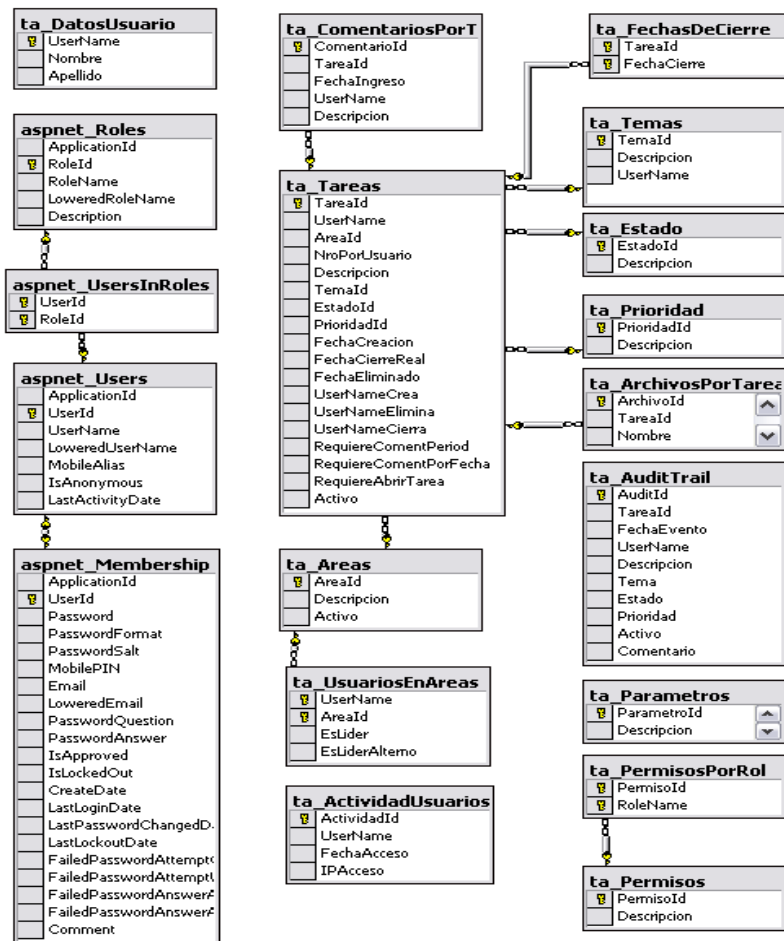
Figura 4.6 Diagrama de base de datos
