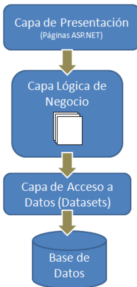
Figura 4.1 Modelo 3 capas
