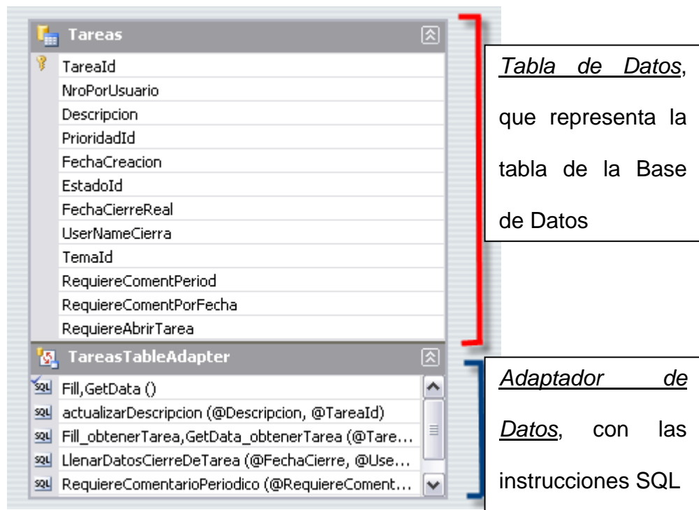
Figura 4.7 Ejemplo de un adaptador de datos
