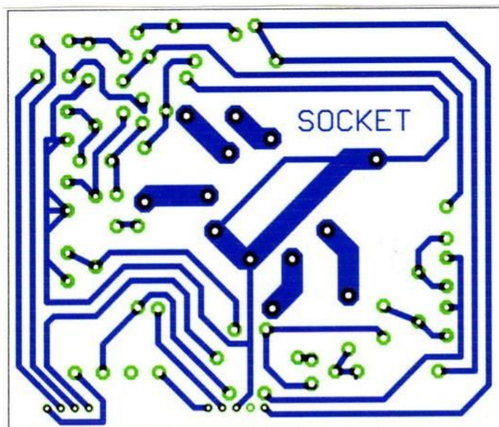
Figura 2.3.8 Sección SOCKET trazado superior e inferior
