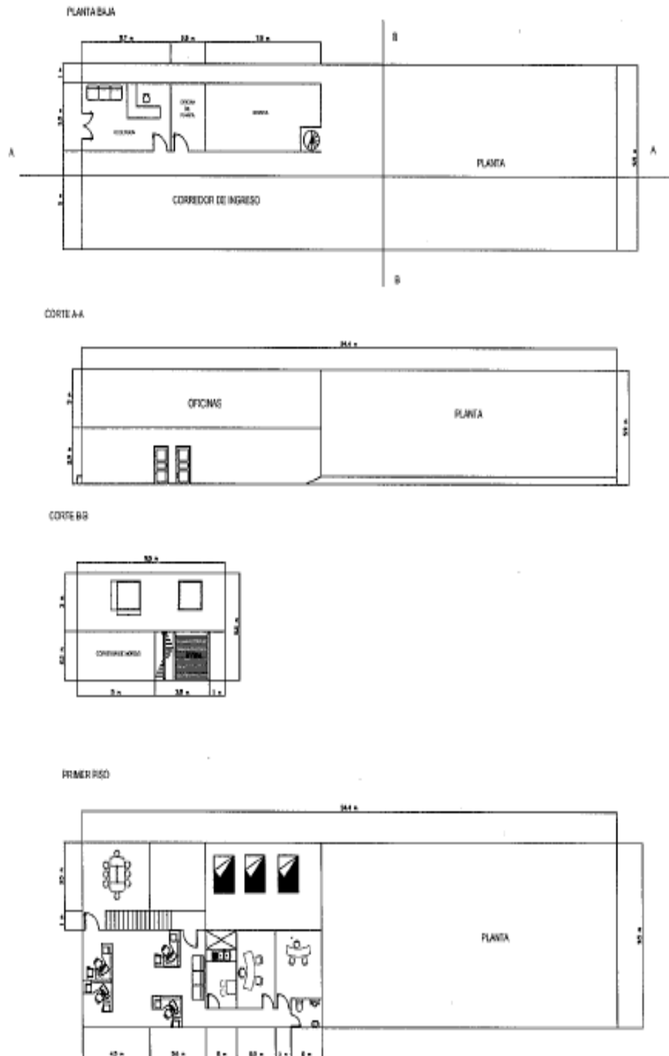
Figura 1.2 Plano de la Corporación J.P.
