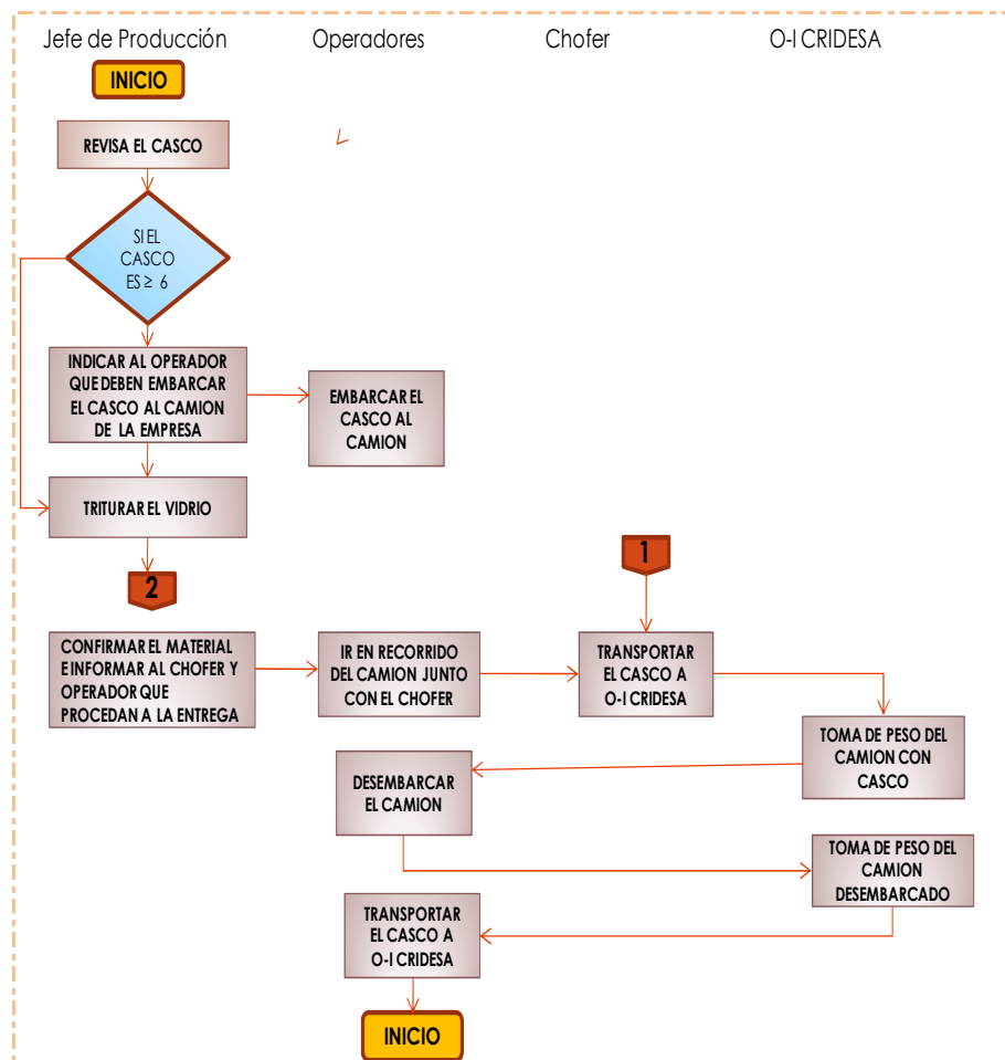
Figura 2.7 Procedimiento de la Etapa de Traslado
