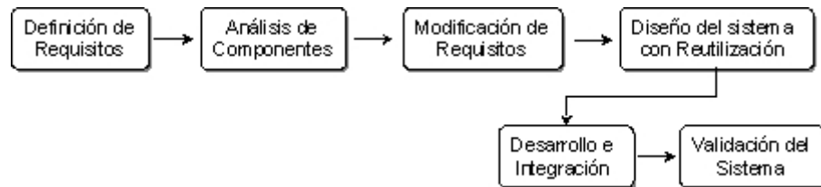
Figura 2.1.5 Desarrollo basado en reutilización de componentes
