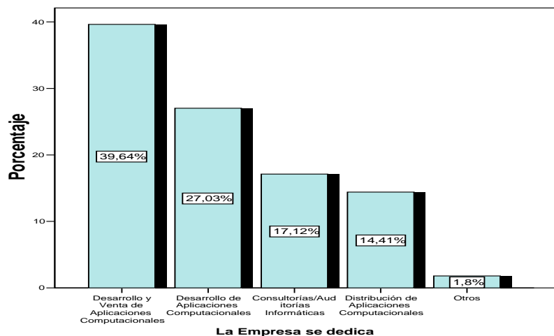
Figura 2.9.3. Ejemplo de un histograma
