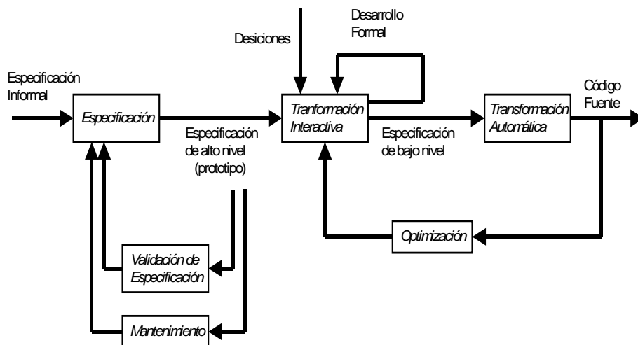
Figura 2.1.4 Paradigma de programación Automática
