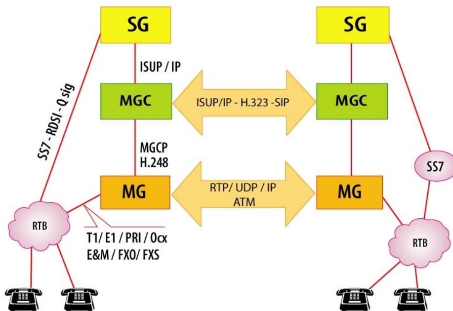
Fig. 3.13 Arquitectura Megaco
