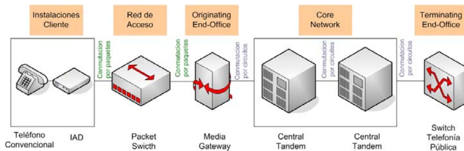
Fig. 4.7 Red Conmutada
