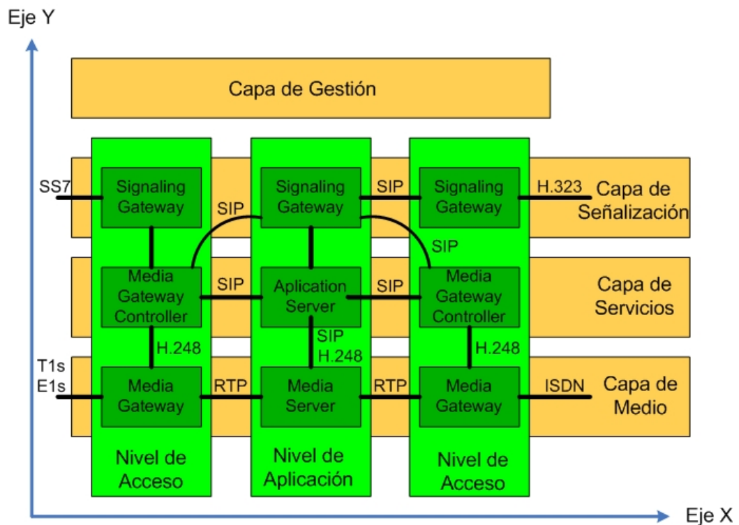
Fig. 4.3 Funciones de la Arquitectura Softswitch
