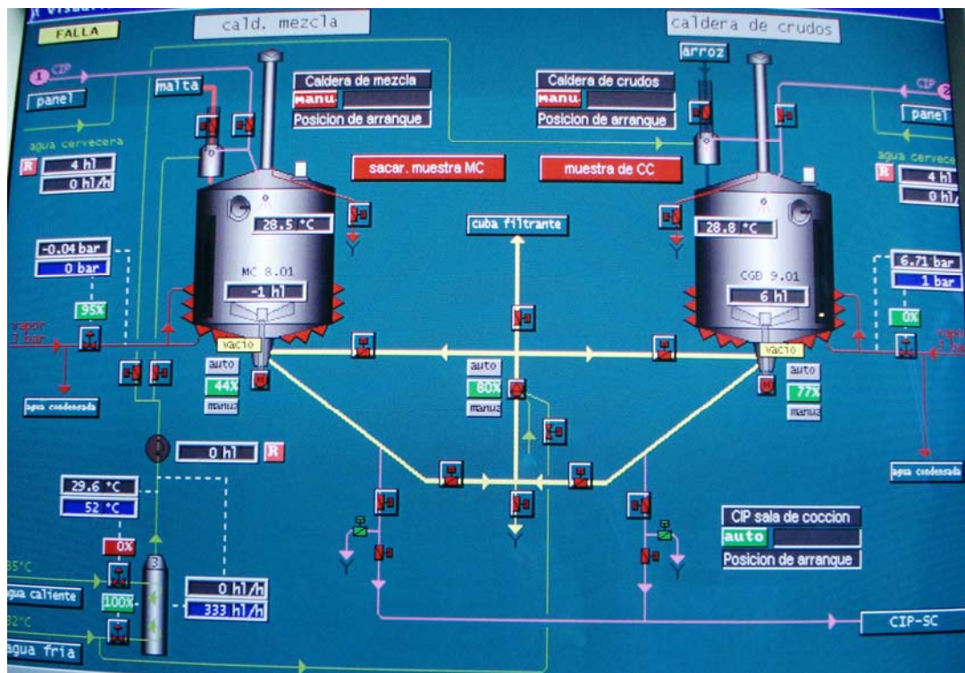
FIGURA 1.4 Proceso de Mosturación de Malta y Arroz
