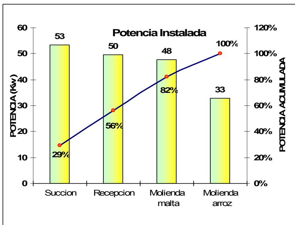
Figura 4.1 Potencia instalada por sistema del proceso de recepción y molienda de materia prima.
