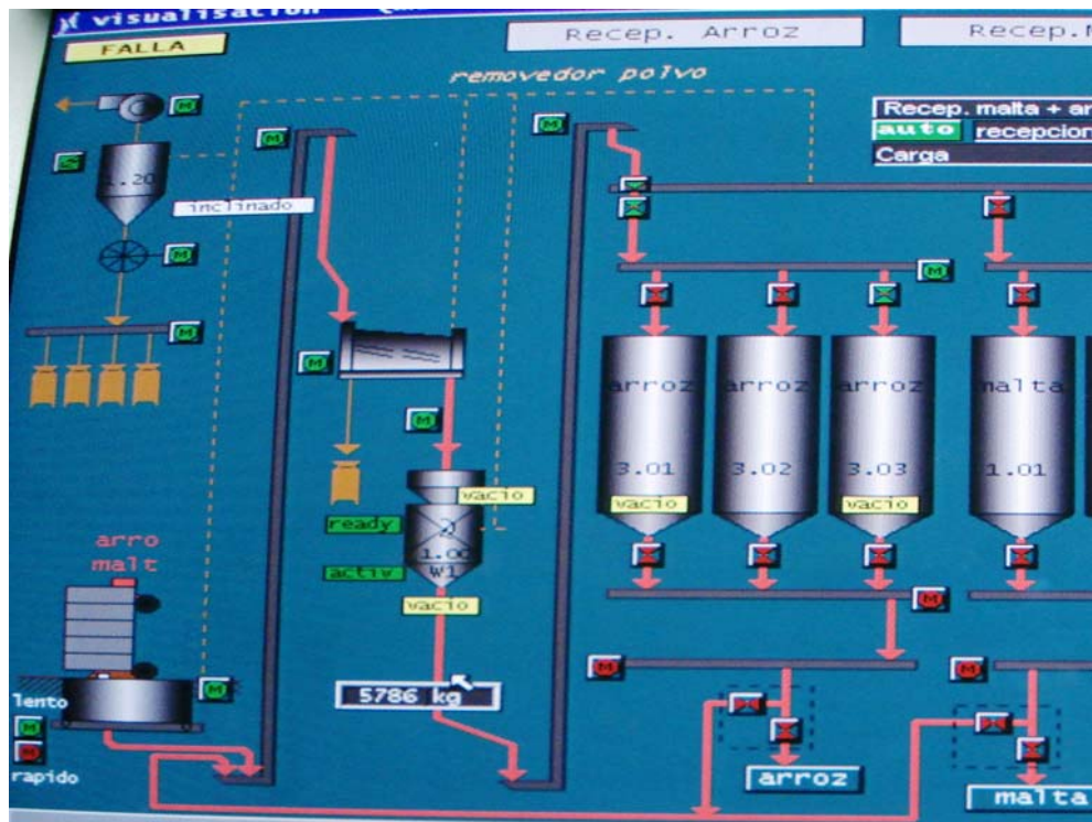
FIGURA 1.1 Sistema de recepción de materia prima
