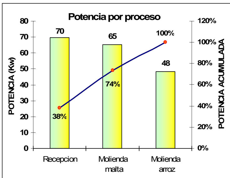
Figura 4.2 Demanda de potencia por sistema del proceso de recepción y molienda de materia prima
