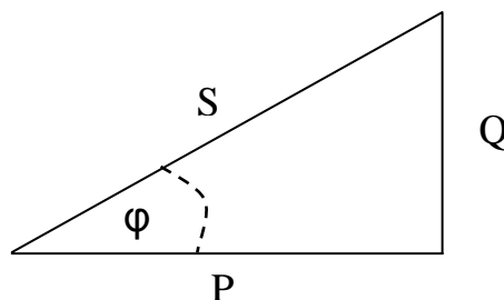
Figura 3.4.- Factor de potencia de la carga
