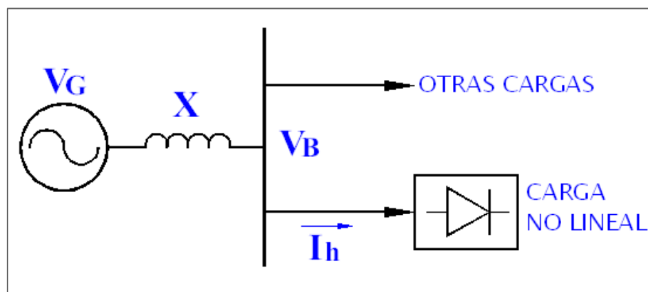
Figura 3.2.- Esquema básico de distorsión Armónica
