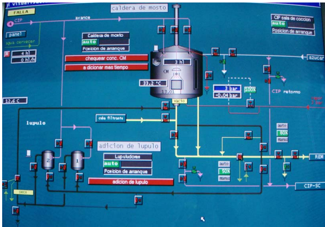
FIGURA 1.7. Proceso de ebullición de mosto
