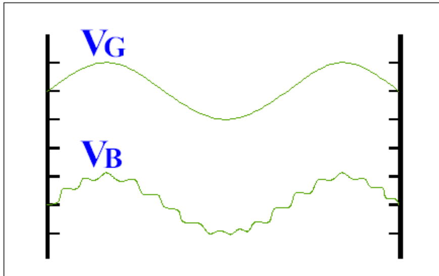
Figura 3.3.- Distorsión de forma de onda de voltaje
