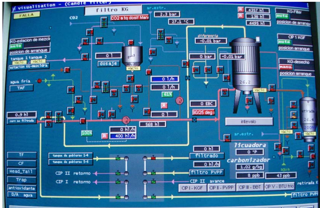
FIGURA 1.12 Proceso de Filtración
