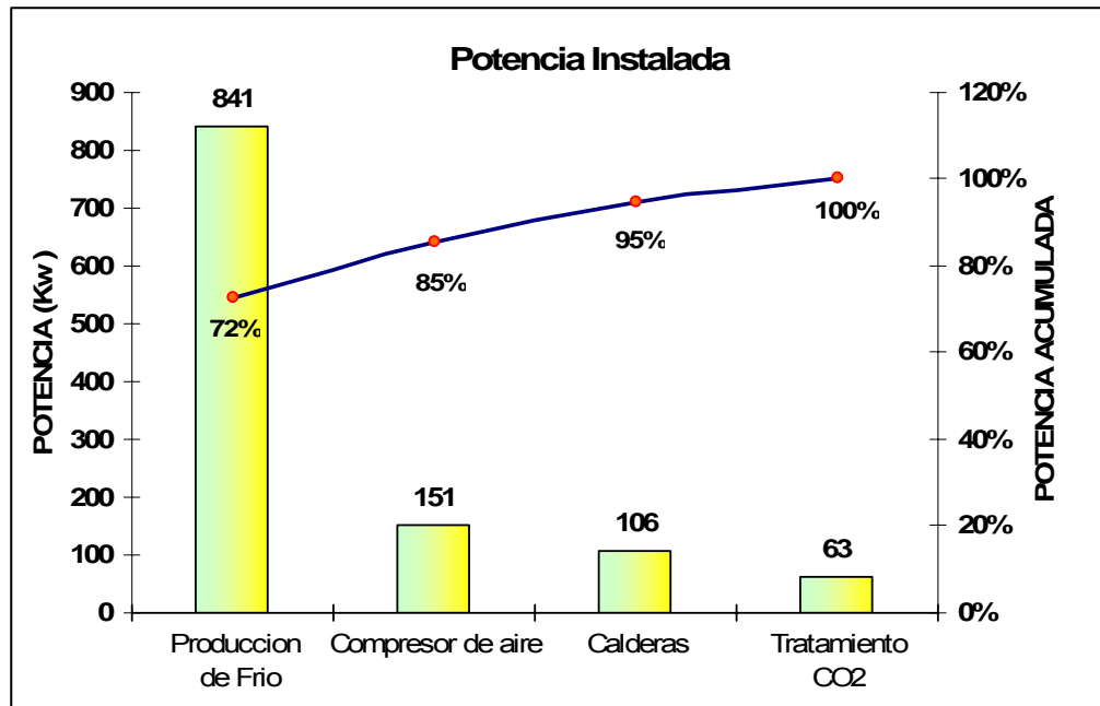
Figura 4.3 Potencia instalada por sistema en área de utilidades
