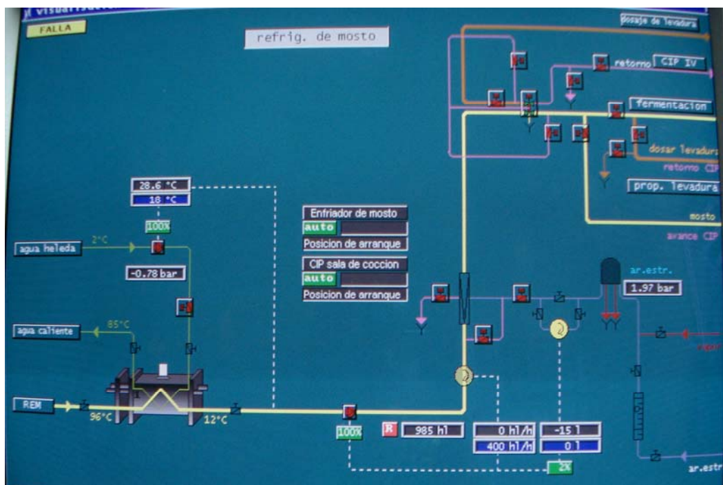
FIGURA 1.9 Proceso de enfriamiento y aireación
