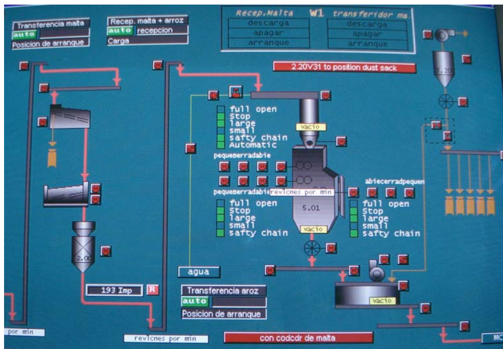
FIGURA 1.2 Sistema de molienda de malta
