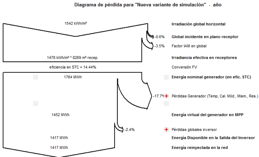
Figura 3.38: Diagrama Pérdidas de la Planta Fotovoltaica.
