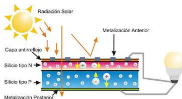
Figura 2.1: Efecto Fotovoltaico [7].
