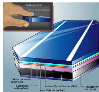
Figura 2.8: Célula Fotovoltaica [14].
