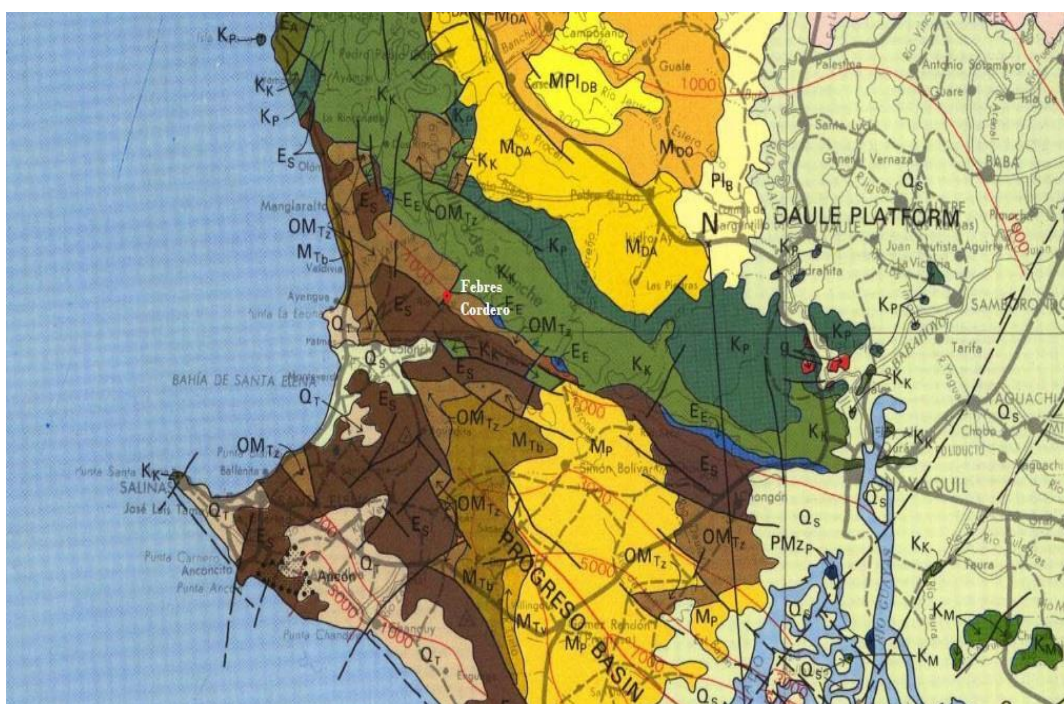
Figura 2.4 Formaciones geológicas presentes en la zona de estudio
