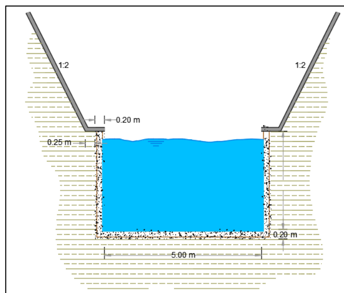
Figura 5.2 Eje de implantación del aliviadero.
