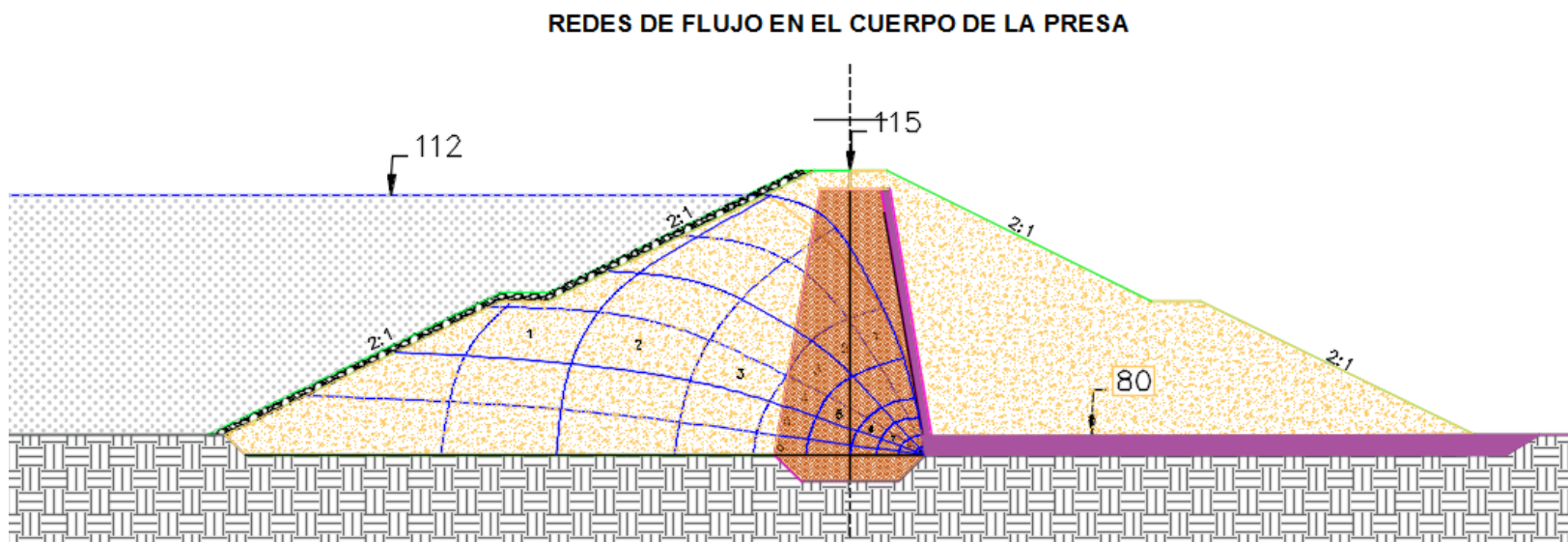
Figura 4.1 Redes de flujo en el cuerpo de la presa.
