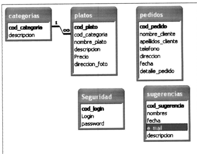
Figura 6.1 Modelo Entidad Relación
